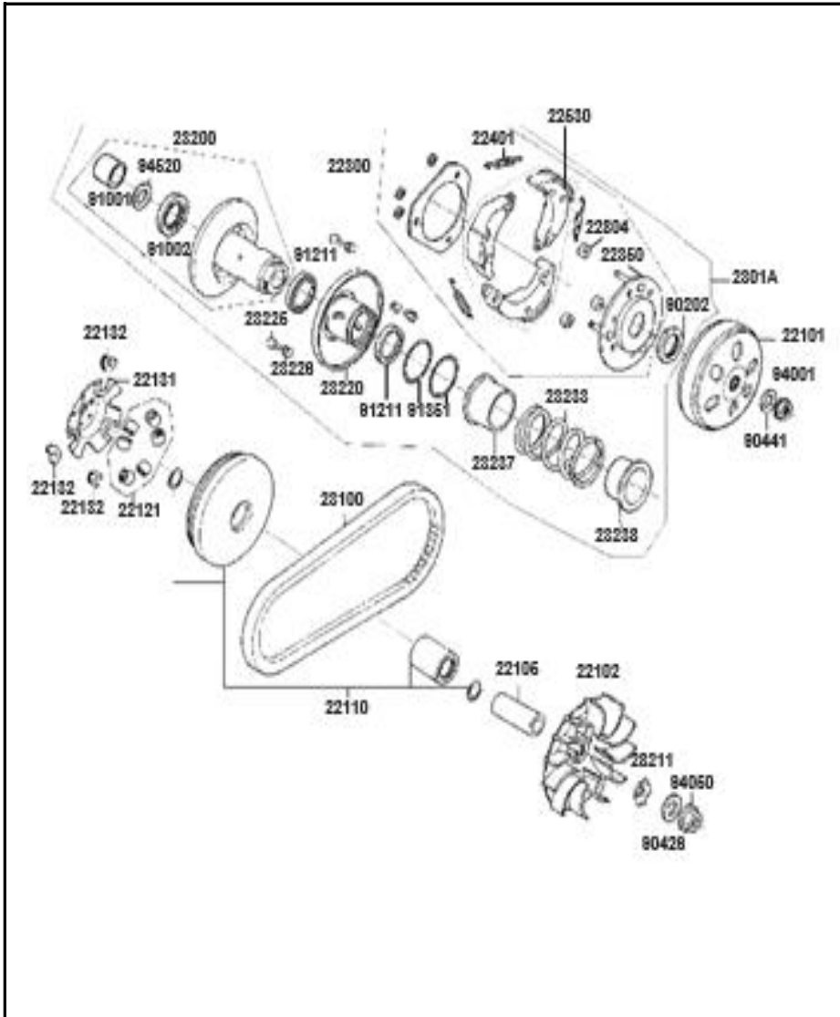
FIGURA N° 5: CLUTCH CENTRIFUGO 1/2
