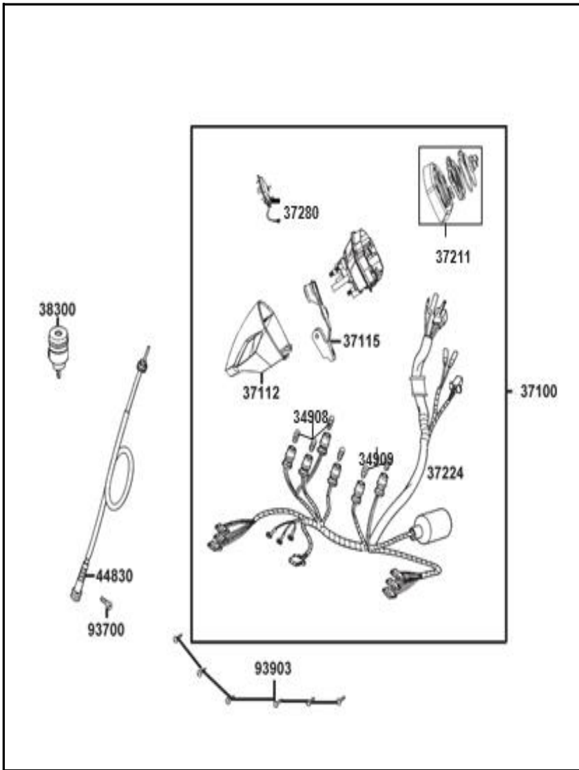
FIGURA N° 11: VELOCÍMETRO
