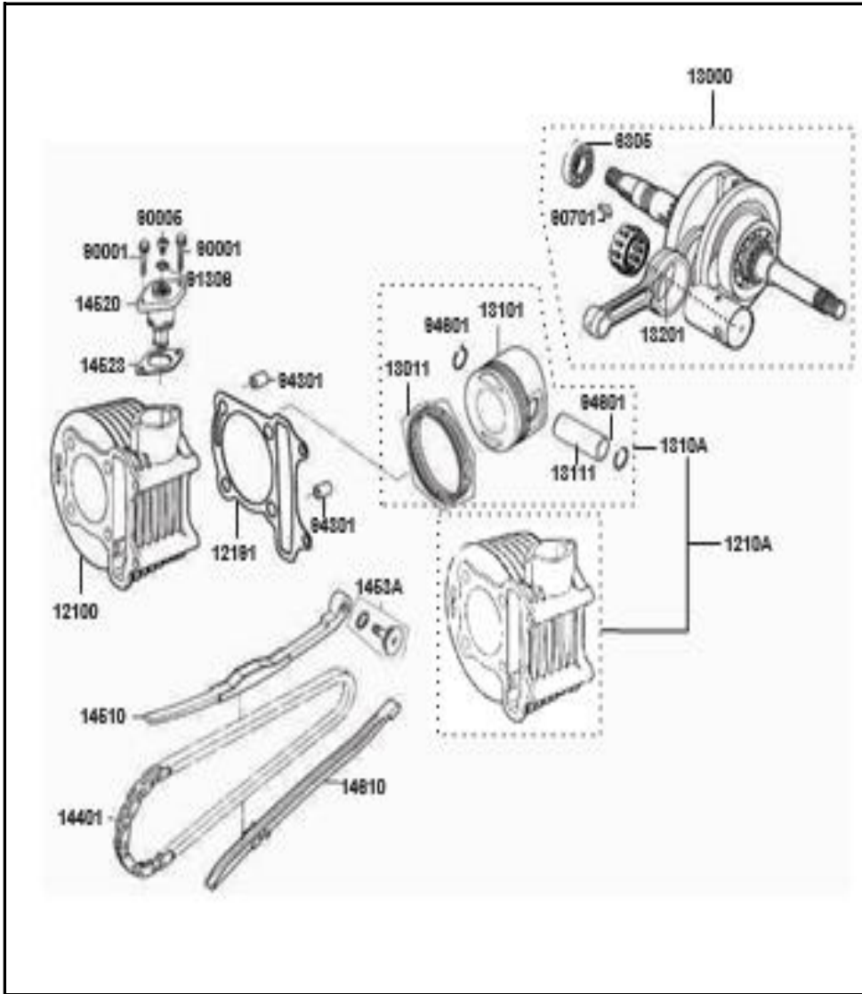
FIGURA Nº 3: CILINDRO - PISTÓN - CIGÜEÑAL
