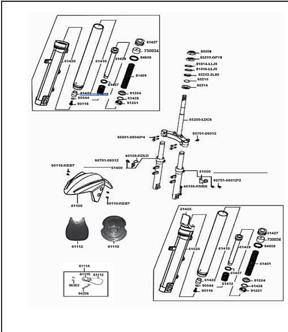
FIGURA N° 15: SUSPENSION DELANTERA 1/2
