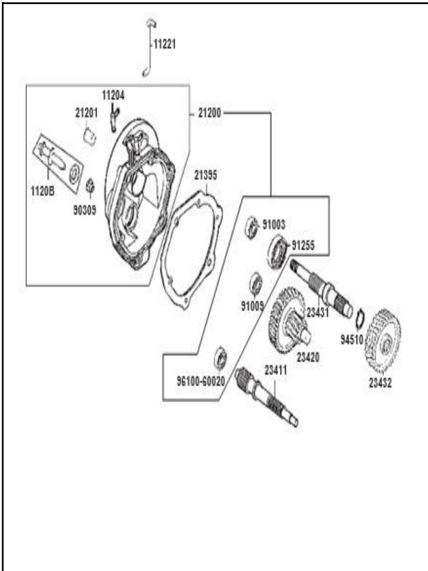
FIGURA N° 8: TRANSMISIÓN
