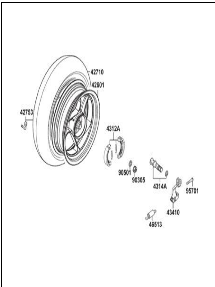
FIGURA N° 17: RIN TRASERO
