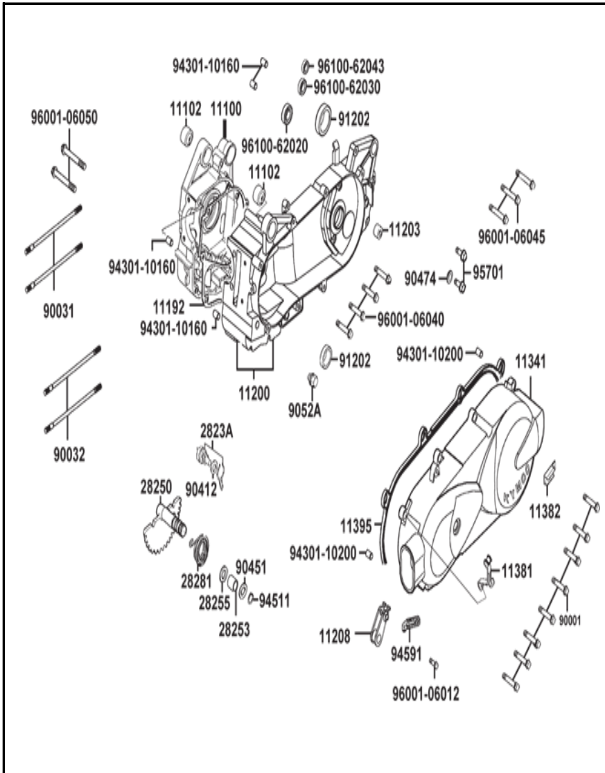
FIGURA N° 1: CARCASAS 1/2
