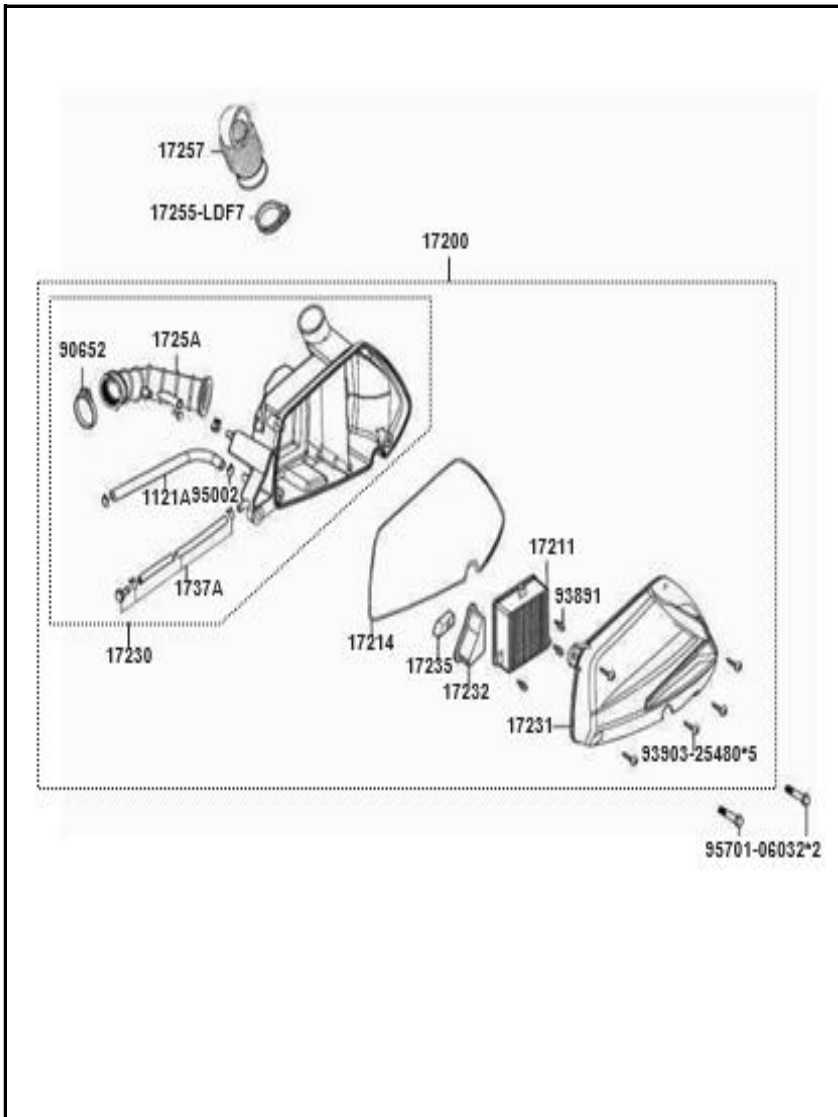
FIGURA N° 22 CAJA FILTRO DE AIRE
