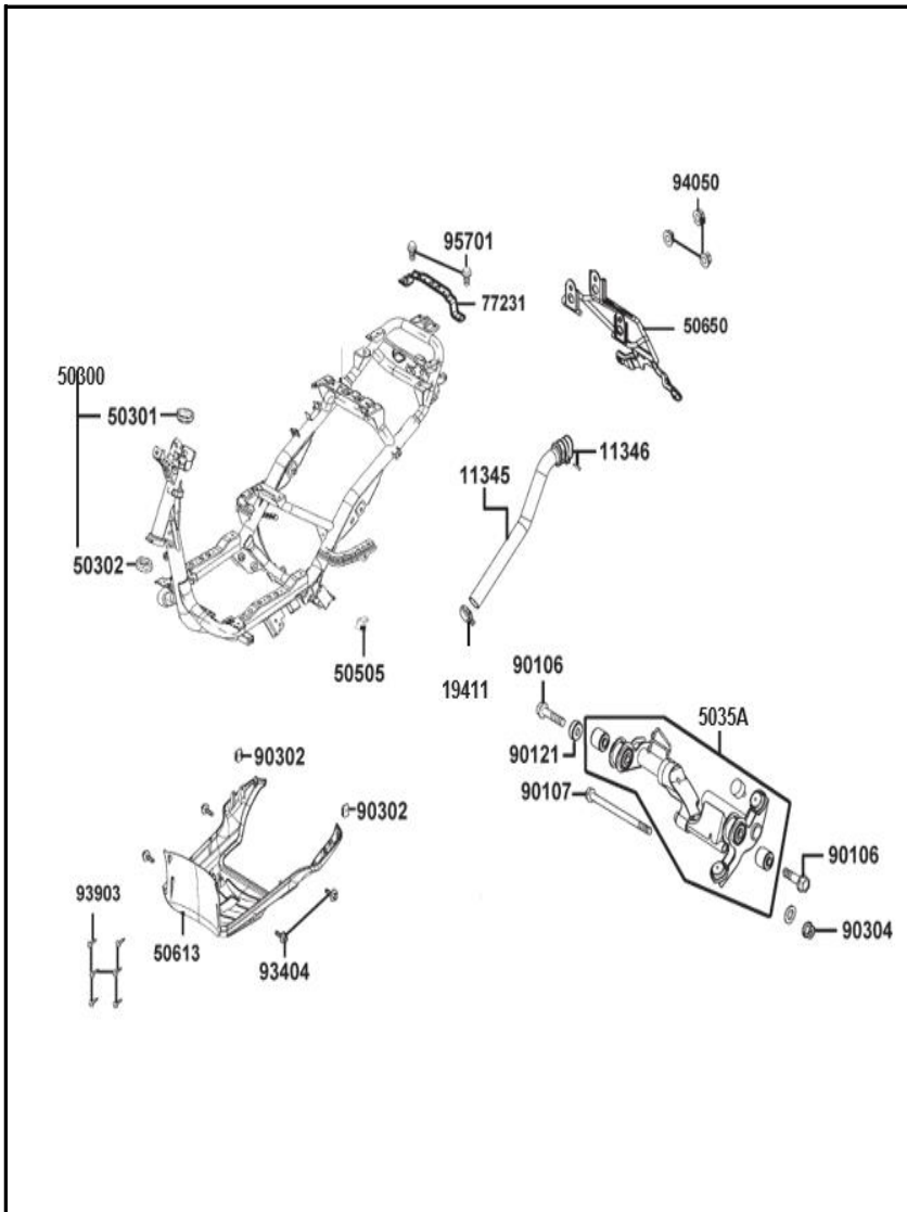
FIGURA N° 29: CHASIS
