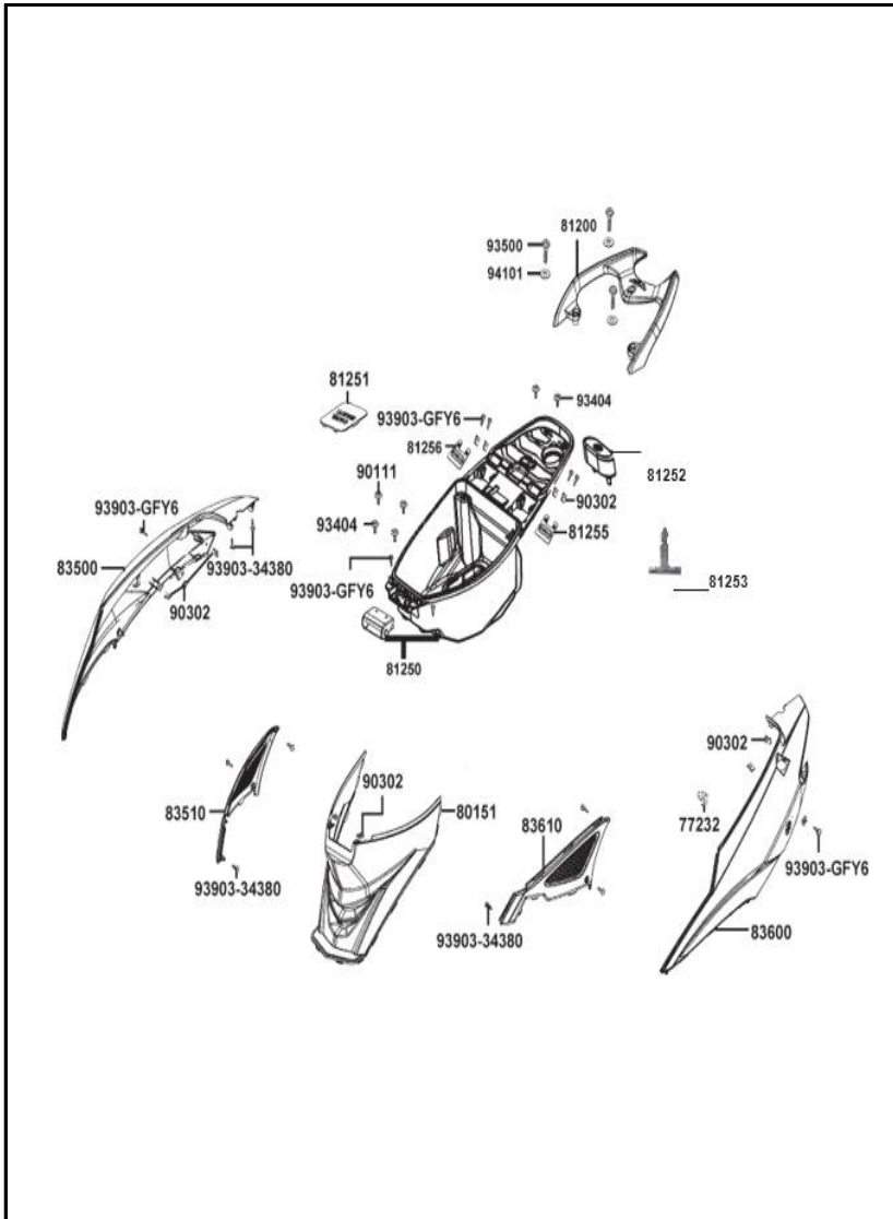
FIGURA N° 21 CUBIERTAS LATERALES - GUANTERA
