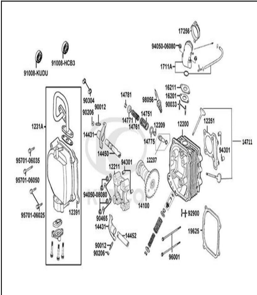
FIGURA N° 2: CULATA 1/2
