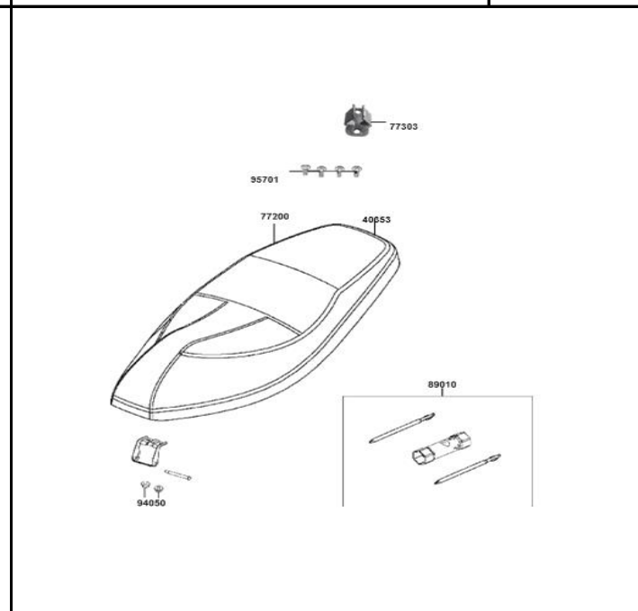
FIG. Nº 18 SILLIN
