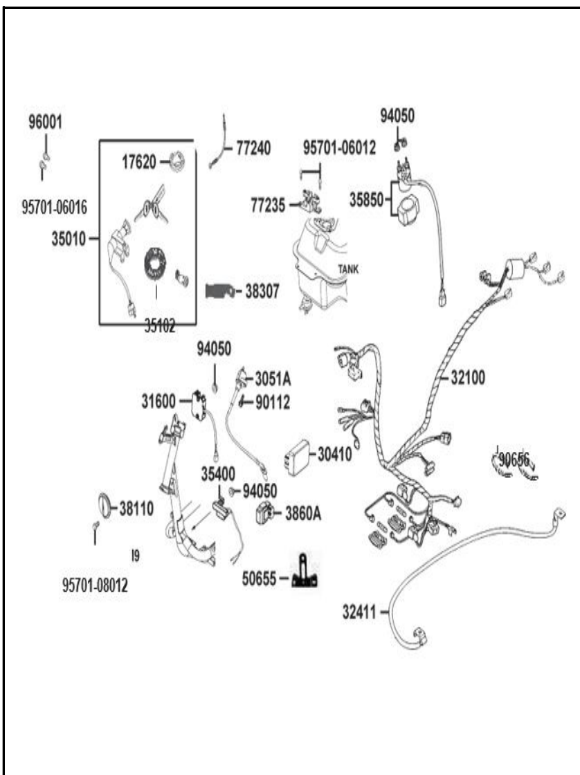
FIGURA N° 28: SISTEMA ELECTRICO
