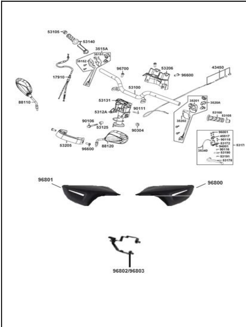
FIGURA N° 12: MANUBRIO - CUBIERTAS MANUBRIO 1/2
