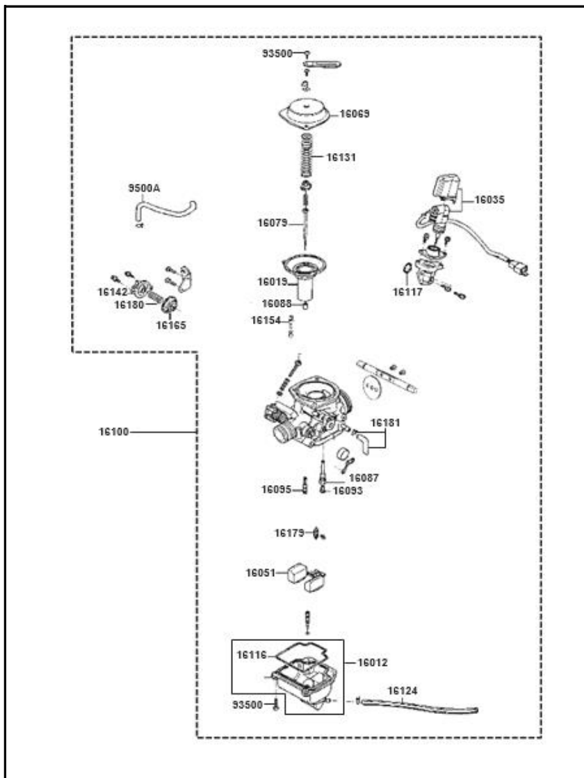
FIGURA N° 9: CARBURADOR
