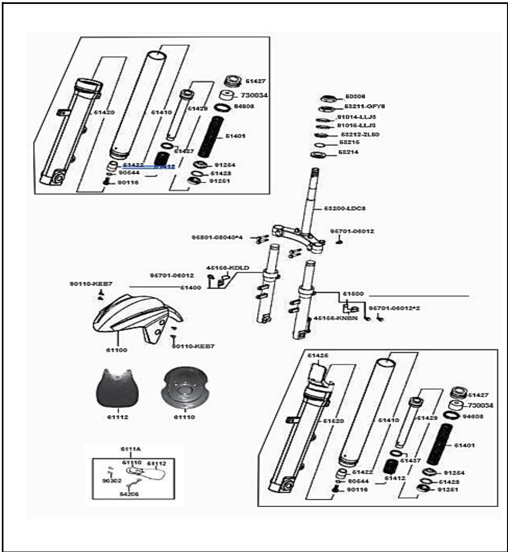
FIGURA N° 15: SUSPENSION DELANTERA 2/2
