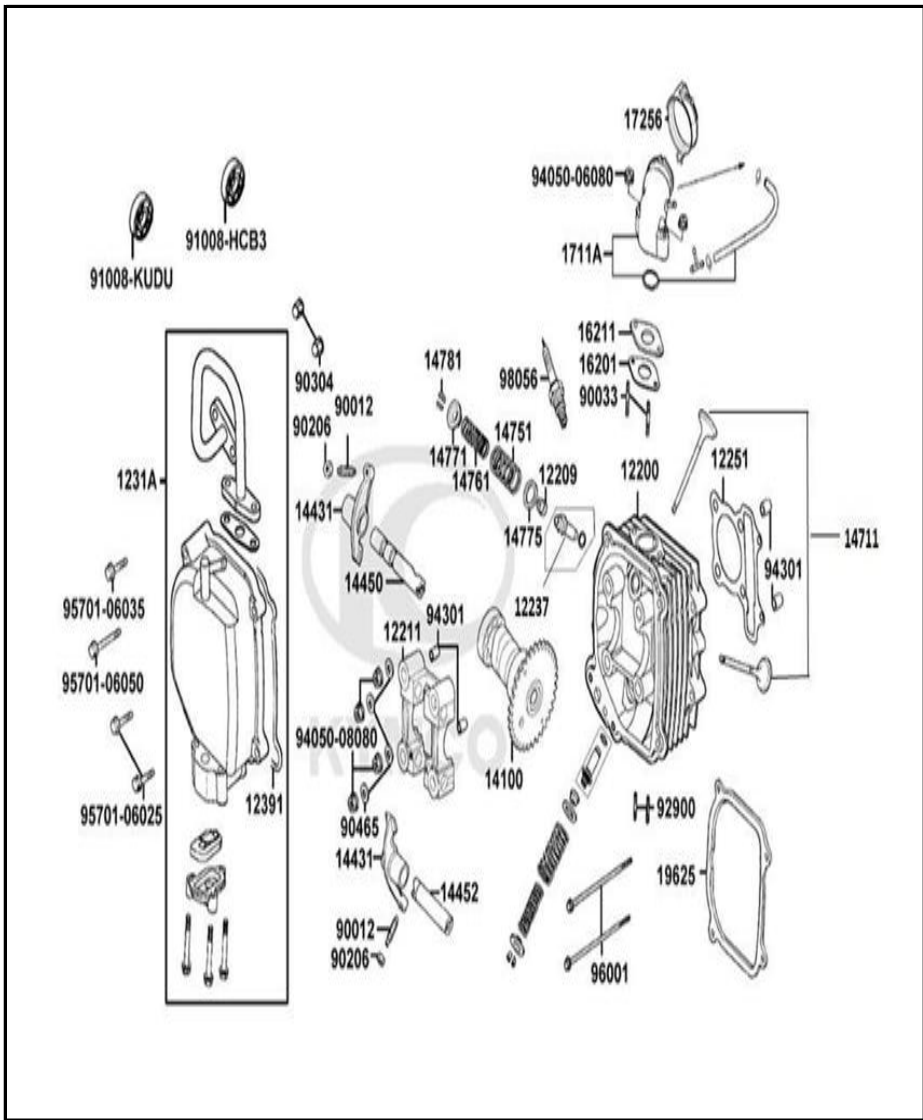
FIGURA N° 2: CULATA 2/2
