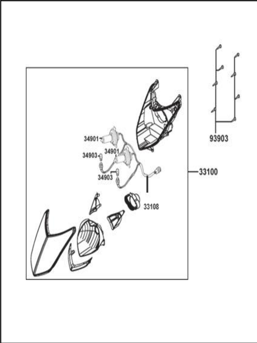
FIGURA N° 10: FAROLA
