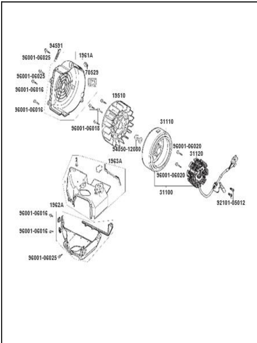
FIGURA N° 7: CUBIERTA VENTILADOR - PLATO BOBINAS
