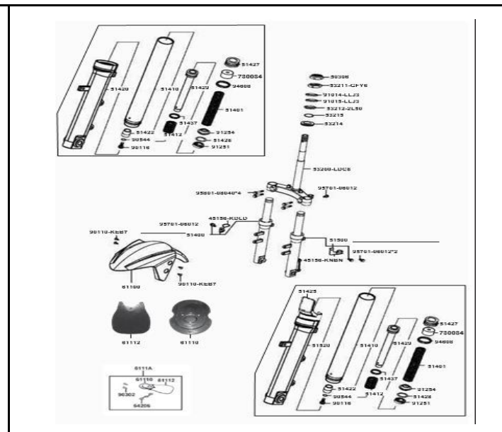
FIG. Nº 15 SUSPENSION DELANTERA
