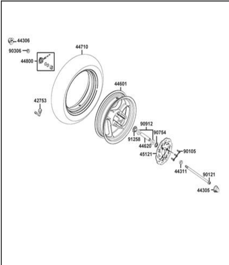
FIGURA N° 16: RIN DELANTERO
