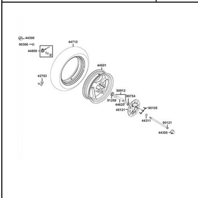
FIG. Nº 16 RIN DELANTERO
