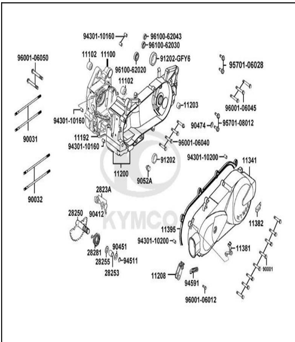
FIGURA N° 1: CARCASAS 2/2
