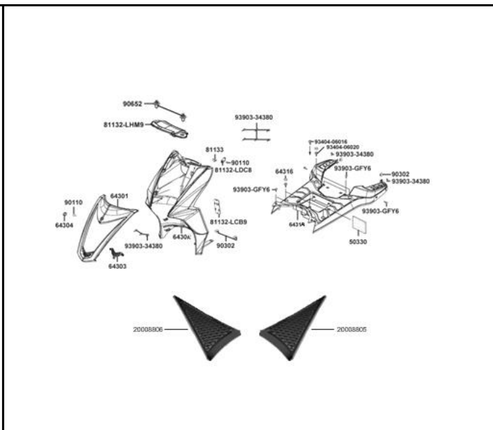
FIG. Nº 14 CUBIERTAS
