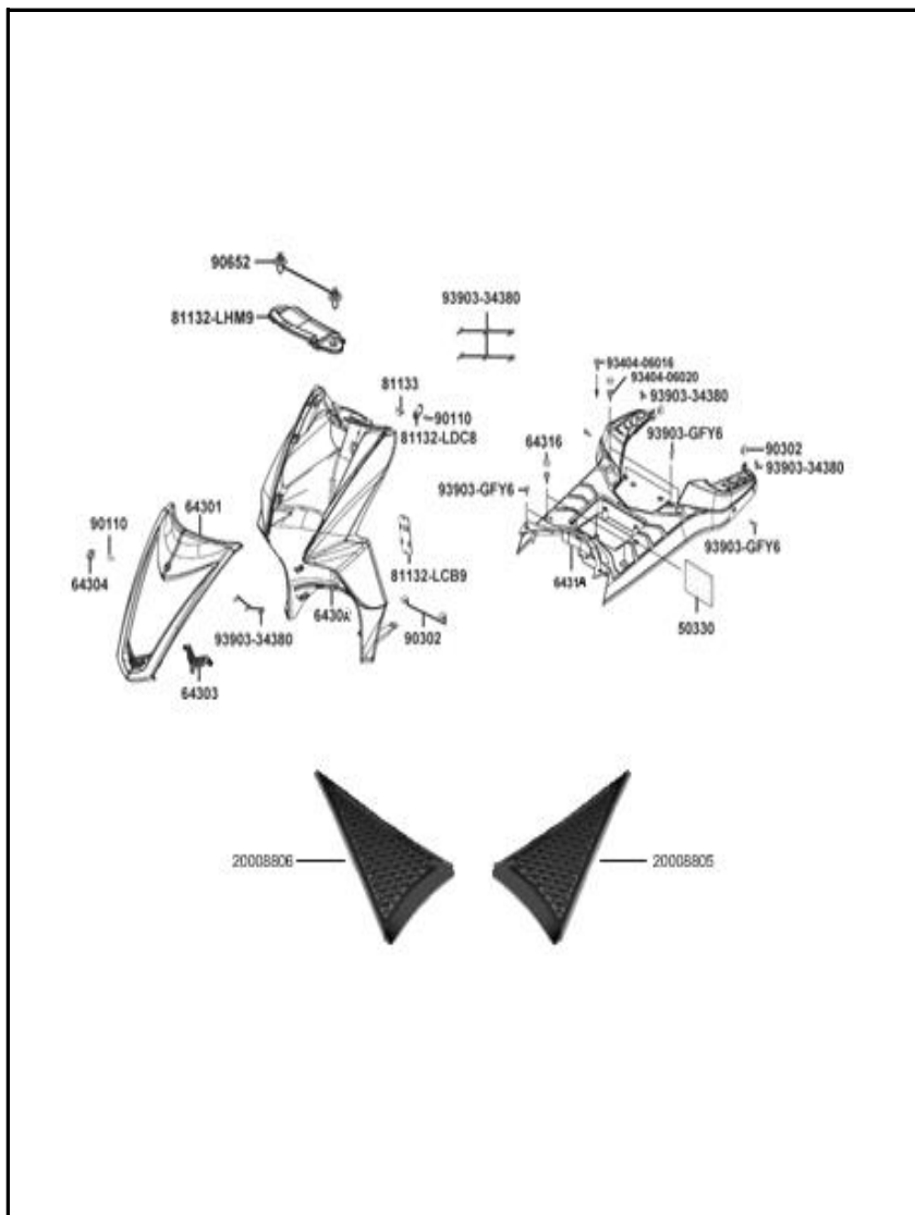
FIGURA N° 14: CUBIERTAS
