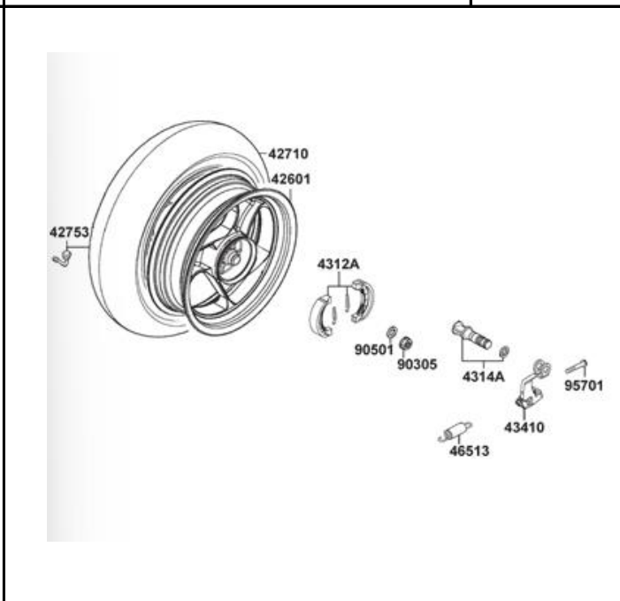
FIG. Nº 17 RIN TRASERO
