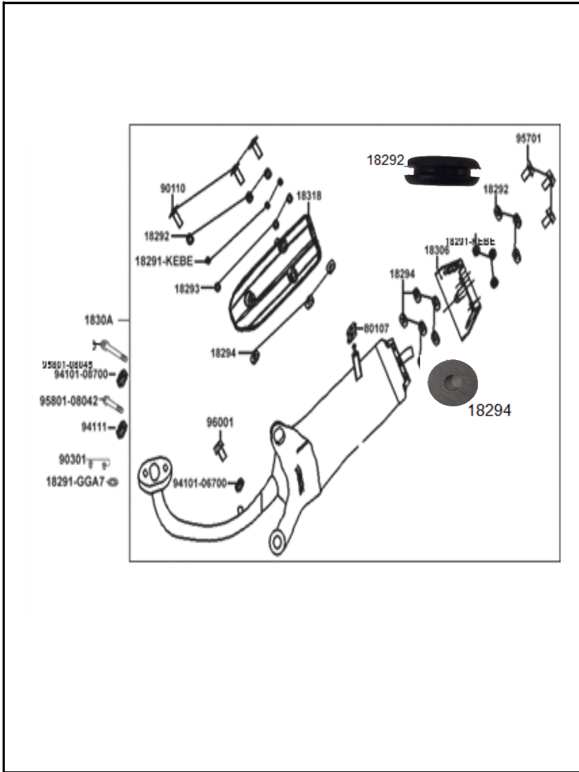
FIGURA N° 23: SILENCIADOR
