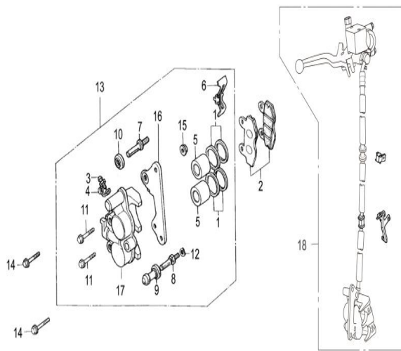
FIG. Nº 28 CALIPER DELANTERO
