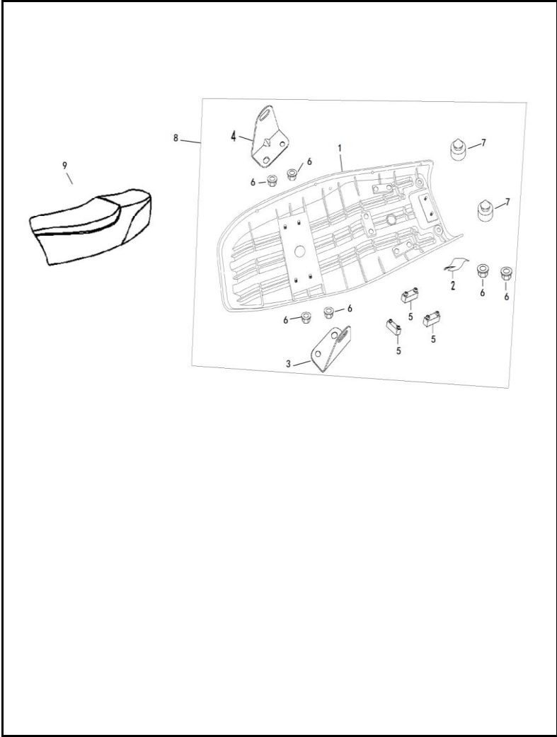
FIGURA N° 31: SILLIN
