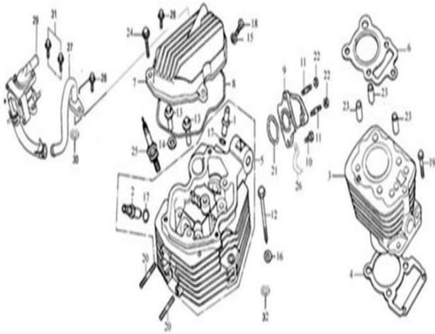
FIG. Nº 1 CULATA
