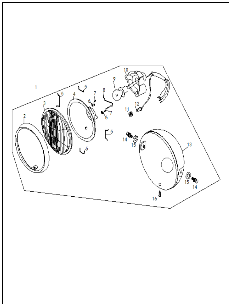
FIGURA N° 22: FAROLA
