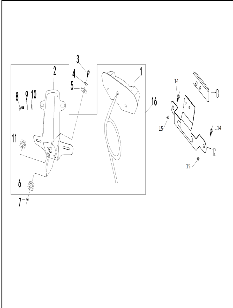
FIGURA N° 43: STOP
