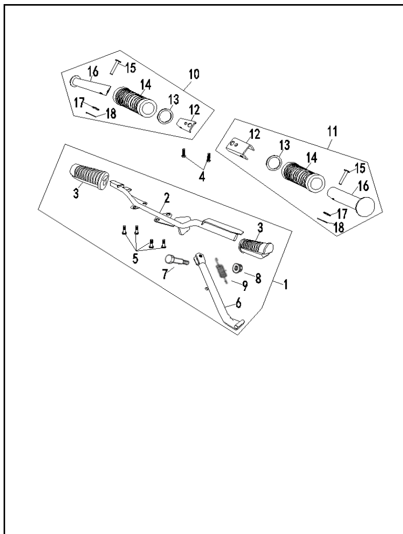
FIGURA N° 38: REPOSAPIE CONDUCTOR - REPOSAPIE PASAJERO - GATO LATERAL
