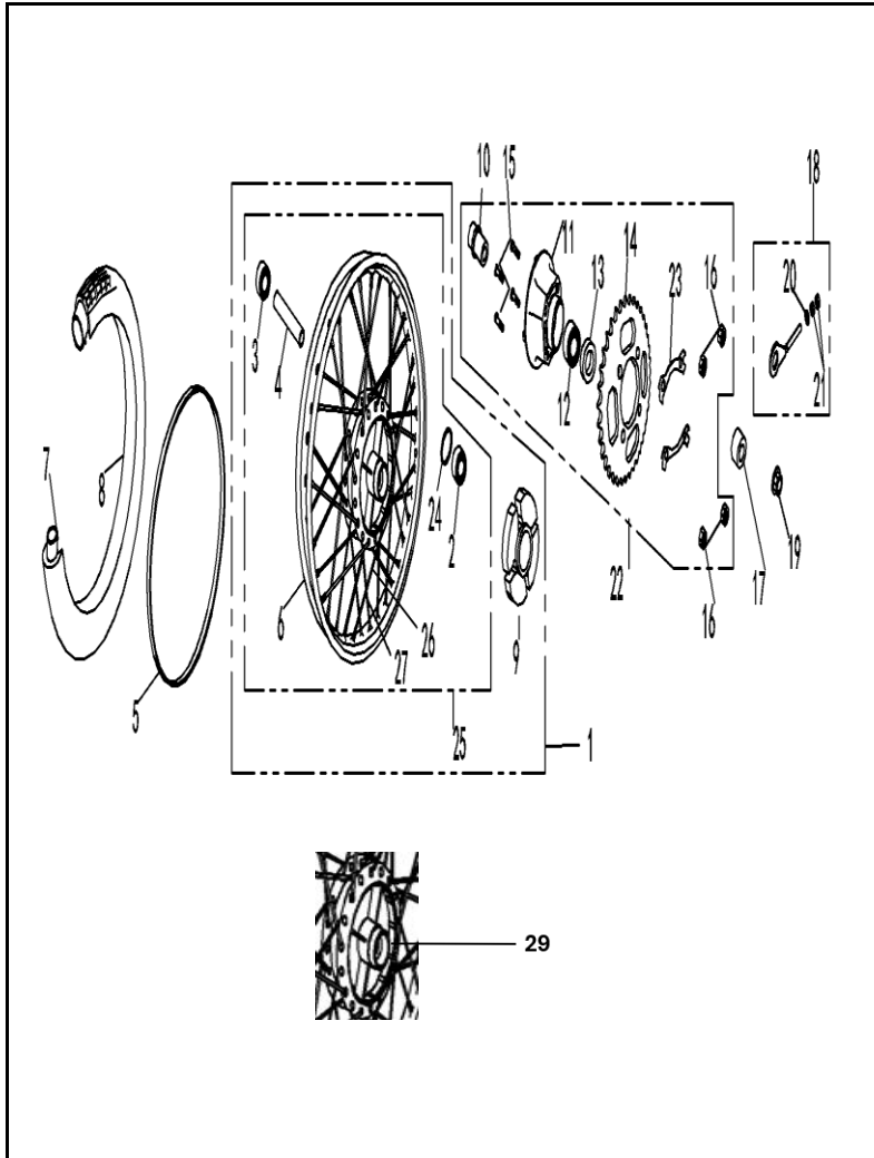
FIGURA N° 36: RUEDA TRASERA (2/2)
