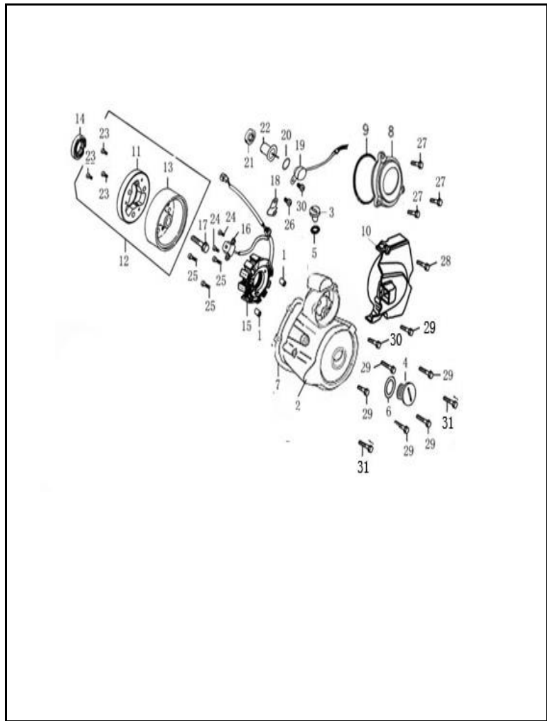
FIGURA N° 6: CUBIERTA VOLANTE - PLATO BOBINAS (2/2)
