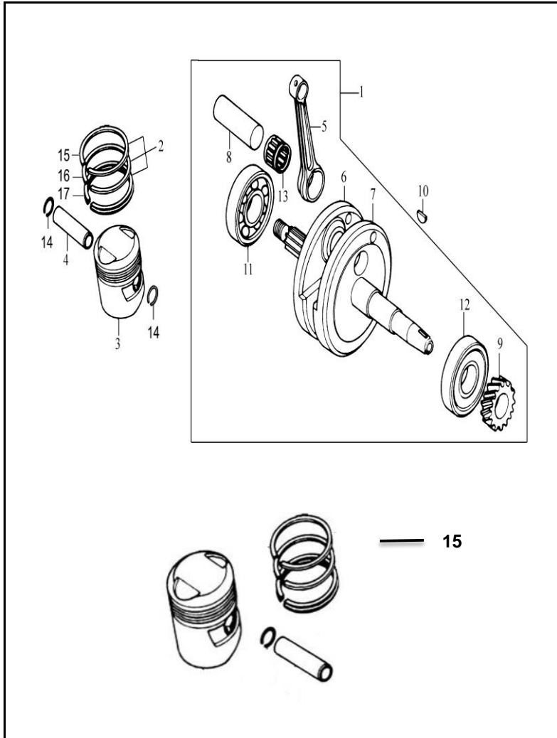
FIGURA N° 9: CIGÜEÑAL - PISTON
