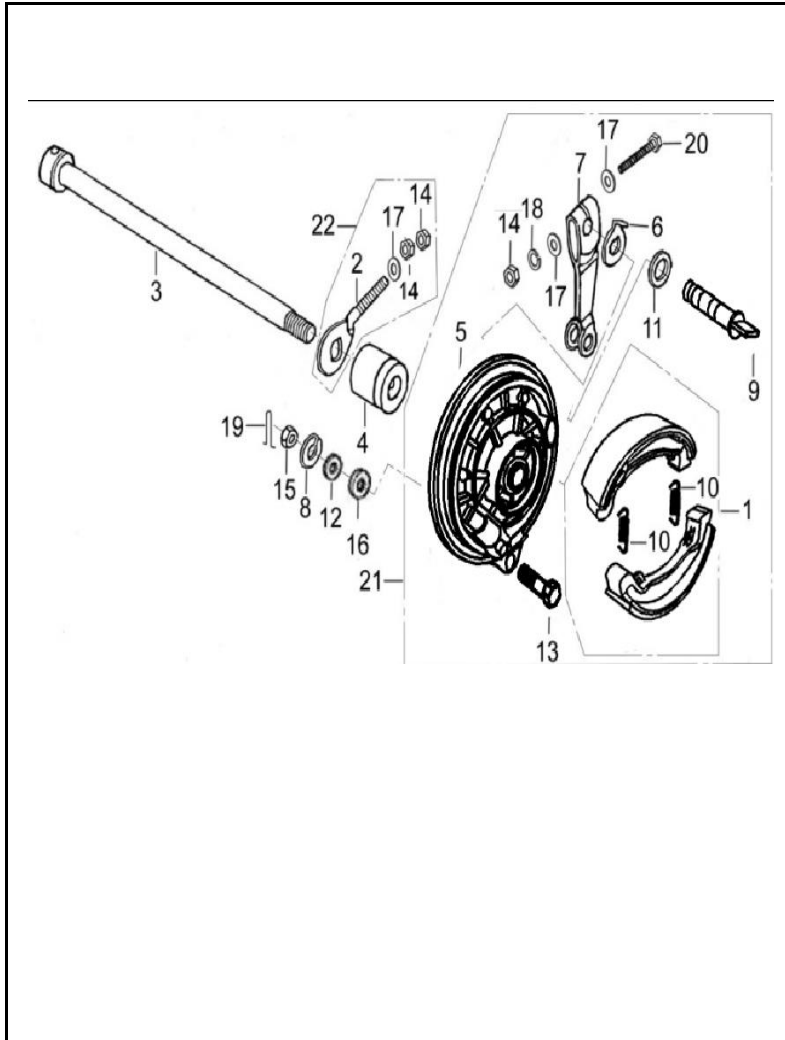
FIGURA N° 37: PORTA BANDAS TRASERO
