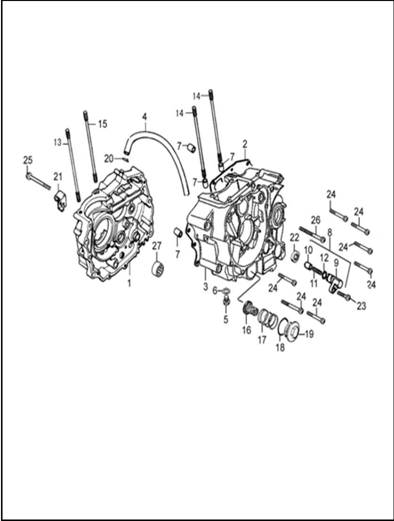
FIGURA N° 8: CARCASAS (2/2)
