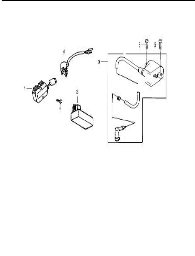
FIGURA N° 16: PARTES ELECTRICAS
