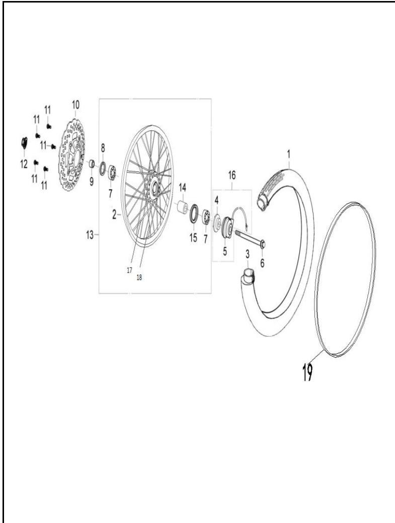
FIGURA N° 35: RUEDA DELANTERA
