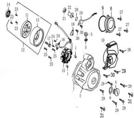
FIG. Nº 6 CUBIERTA VOLANTE - PLATO BOBINAS
