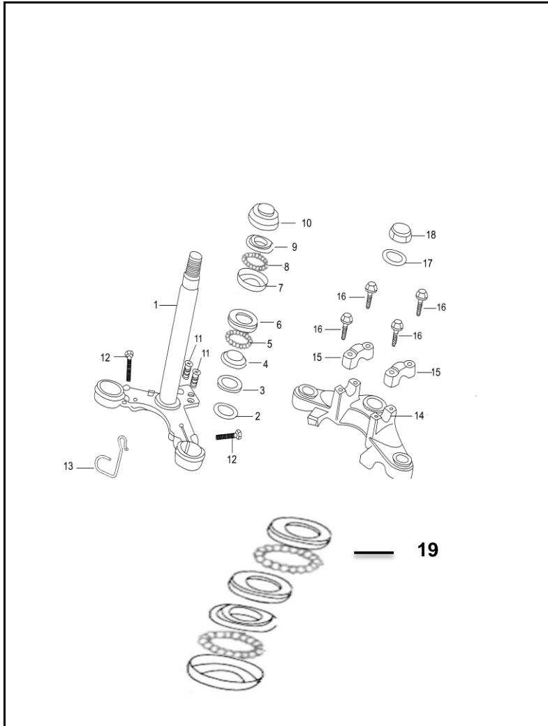
FIGURA N° 21: ESPIGA CENTRAL - CABEZA ESPIGA
