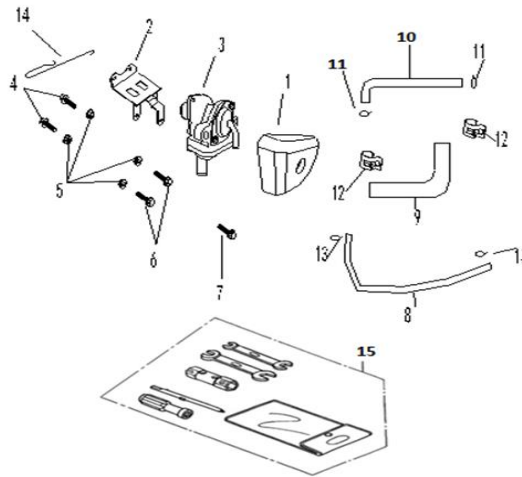
FIG. Nº 44 VALVULA DE AIRE - ESTUCHE HERRAMIENTAS
