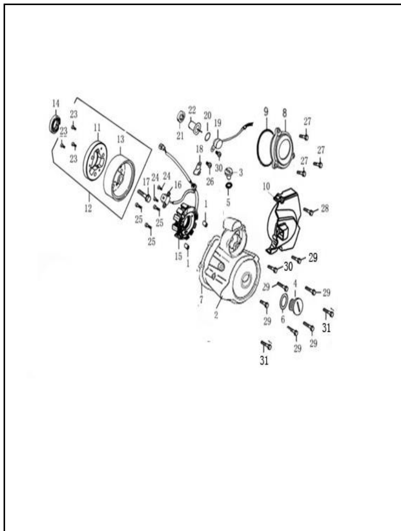
FIGURA N° 6: CUBIERTA VOLANTE - PLATO BOBINAS (1/2)
