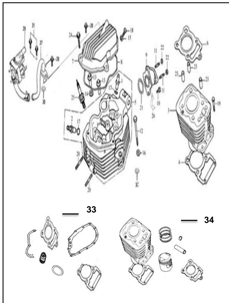
FIGURA N° 1: CULATA - CILINDRO (2/2)
