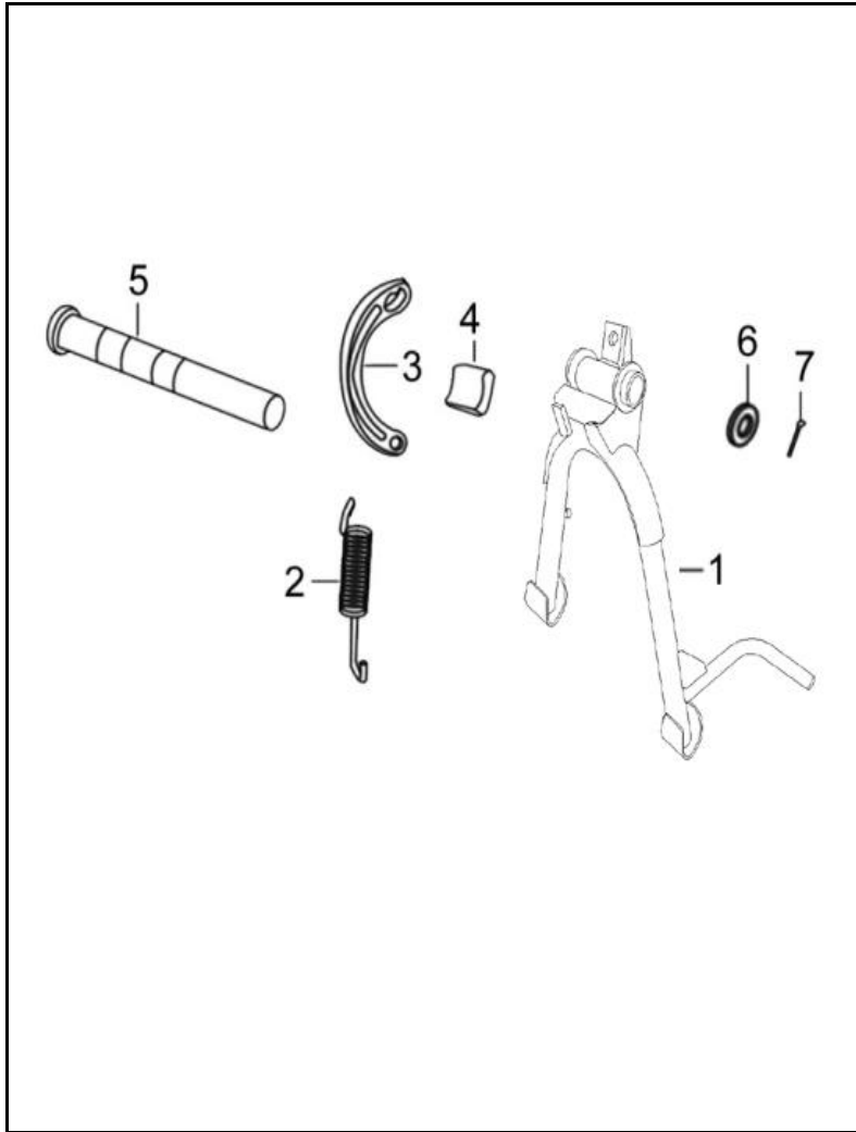
FIGURA N° 32: GATO CENTRAL
