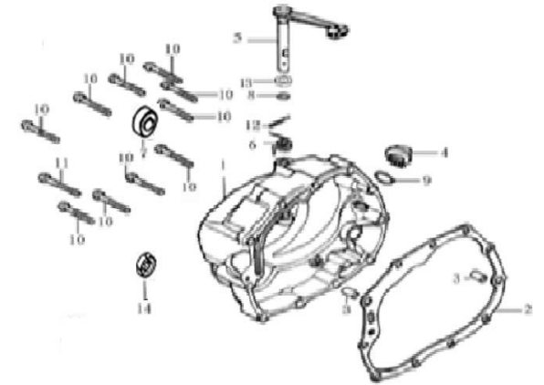
FIG. Nº 3 CUBIERTA CLUTCH
