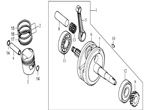
FIG. Nº 9 CIGÜEÑAL - PISTON
