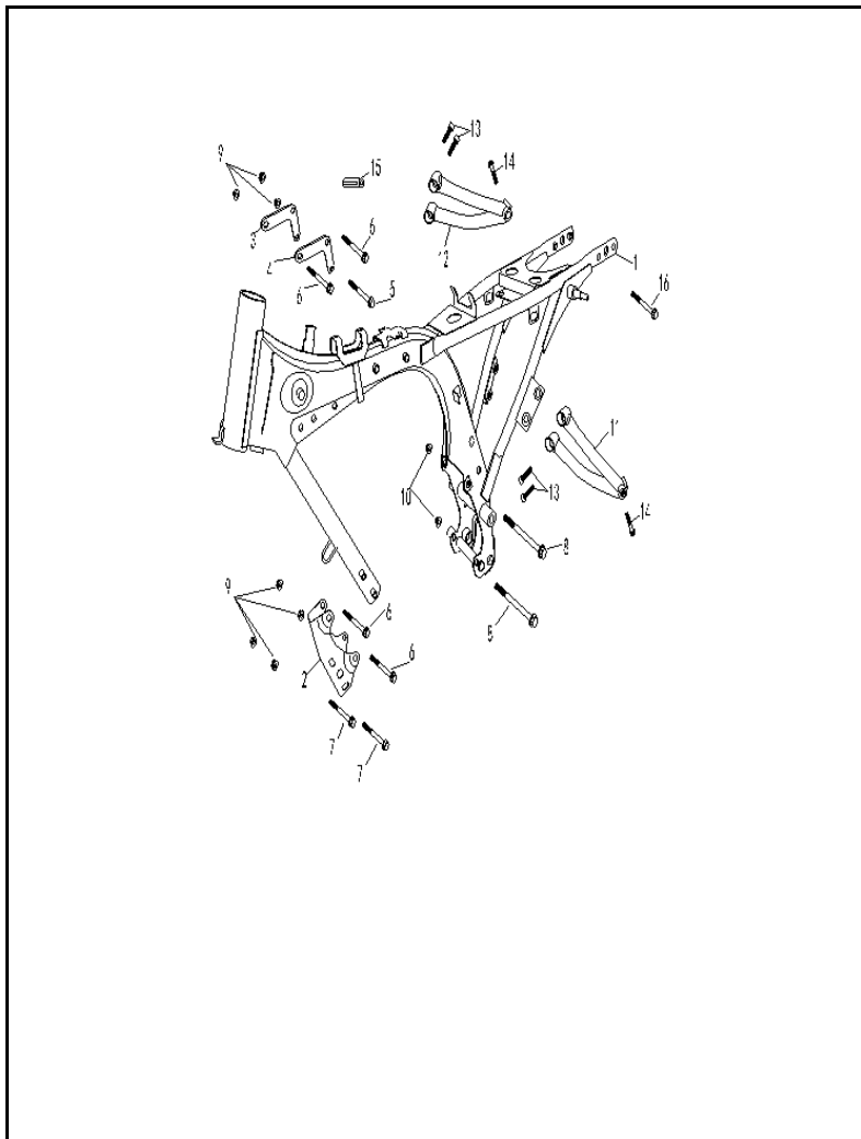
FIGURA N° 19: COMPLEMENTOS CHASIS
