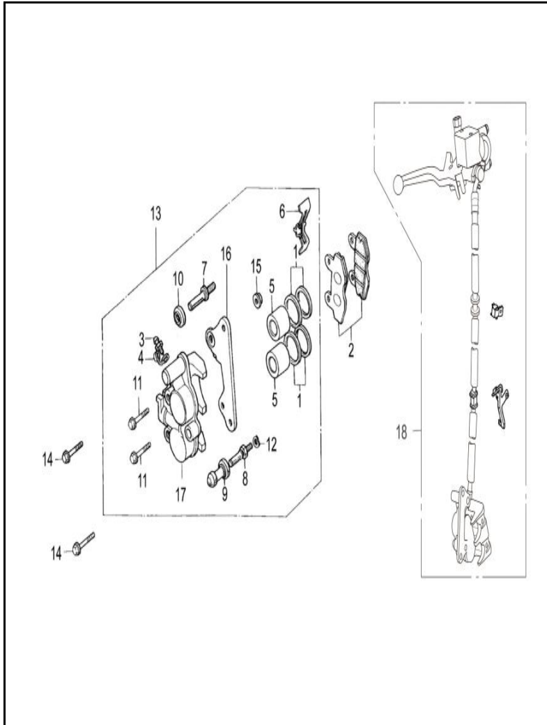
FIGURA N° 28: CALIPER DELANTERO
