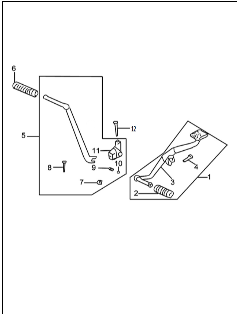
FIGURA N° 12: PEDAL CRANK - PEDAL CAMBIOS
