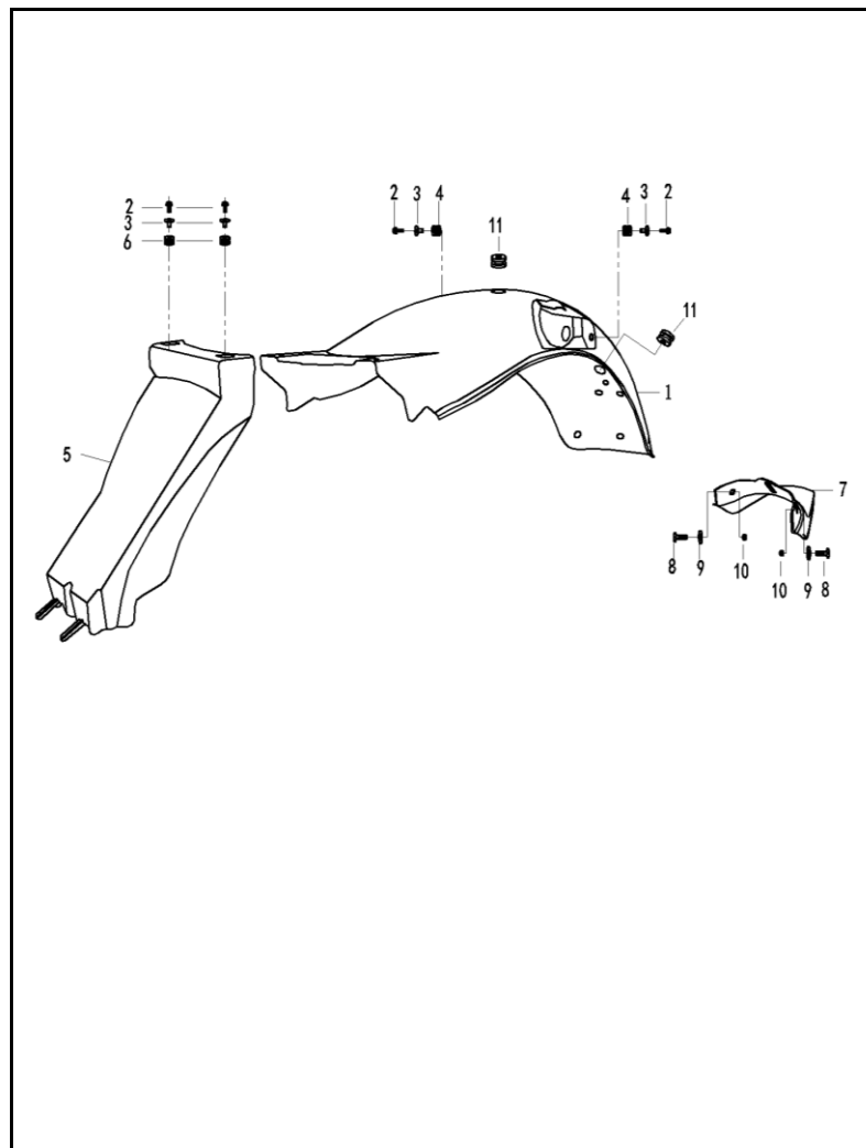
FIGURA N° 40: GUARDABARRO TRASERO
