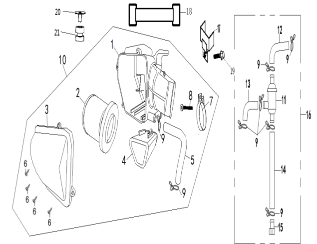
FIG. Nº 18 CAJA FILTRO AIRE - FILTRO GASOLINA
