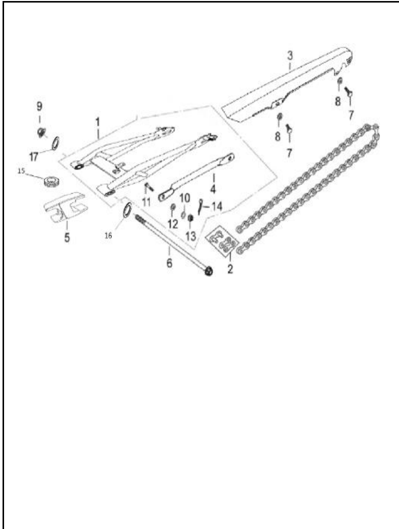
FIGURA N° 34: BRAZO OSCILANTE - GUARDACADENA
