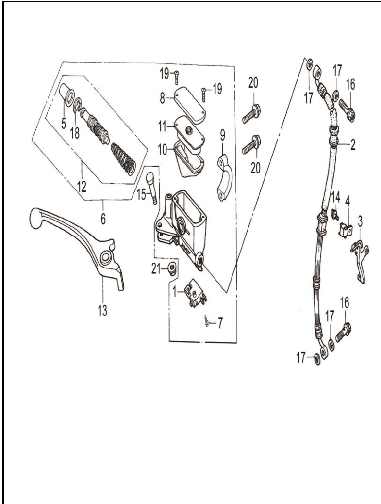
FIGURA N° 27: BOMBA FRENO DELANTERO
