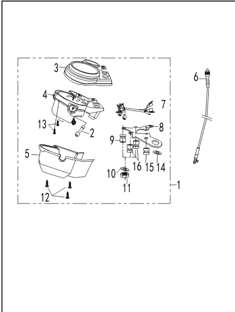
FIGURA N° 24: VELOCIMETRO
