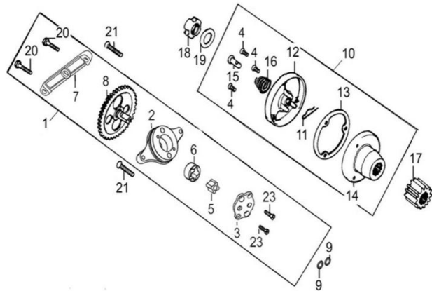
FIG. Nº 7 BOMBA ACEITE - FILTRO CENTRIFUGO ACEITE
