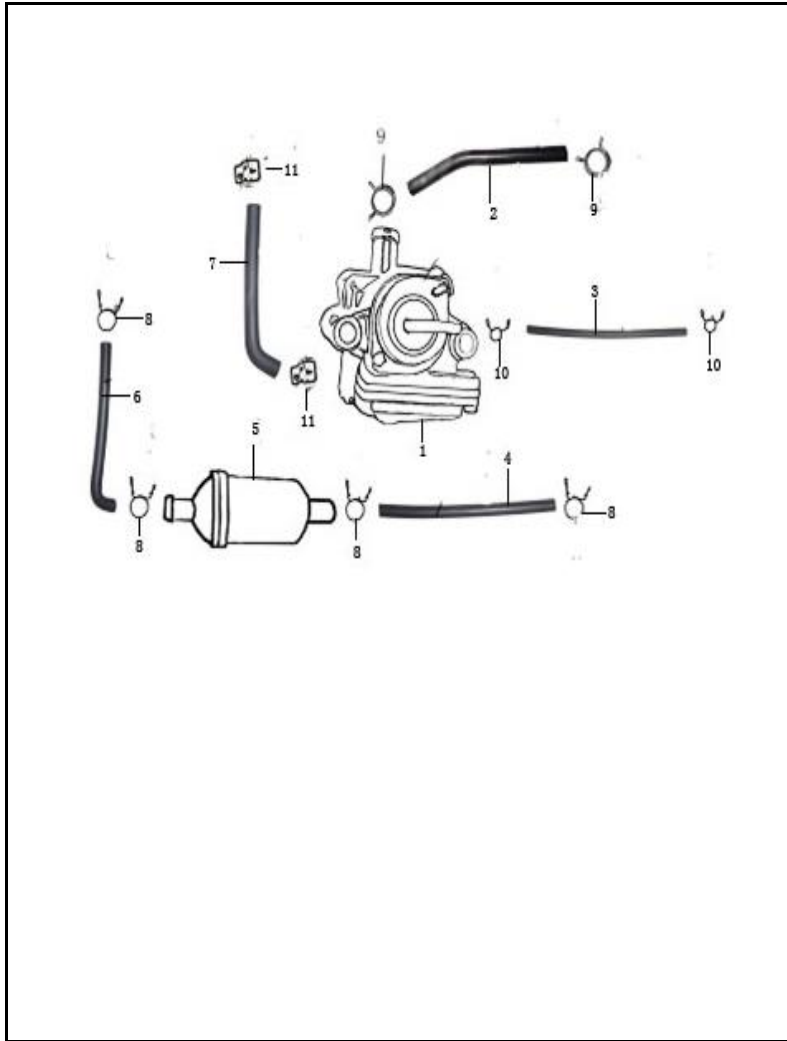
FIGURA N° 17: FILTRO DE GASOLINA
