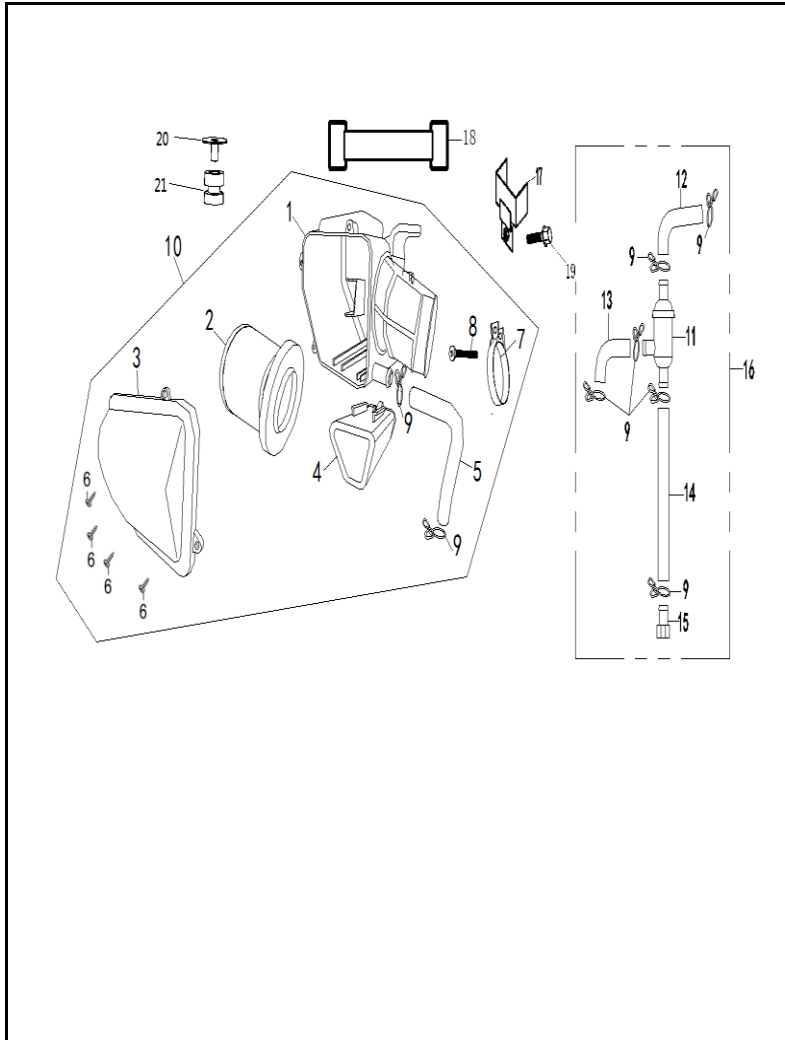
FIGURA N° 18: CAJA FILTRO AIRE - FILTRO GASOLINA
