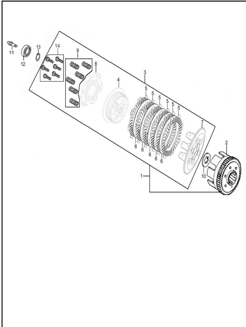
FIGURA N° 5: CLUTCH (6 DISCOS)
