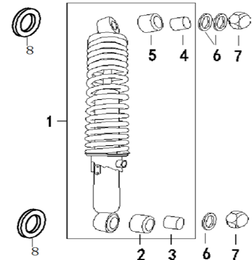
FIG. Nº 39 AMORTIGUADOR TRASERO
