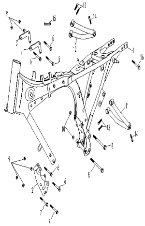
FIG. Nº 19 COMPLEMENTOS CHASIS
