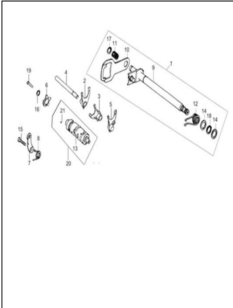
FIGURA N° 11: EJE CAMBIOS - EJE SELECTOR CAMBIOS
