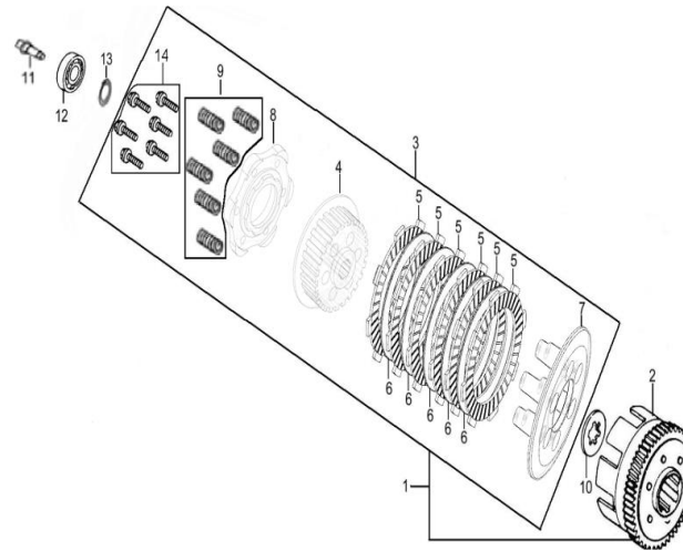
FIG. Nº 5 CLUTCH 6 DISCOS
