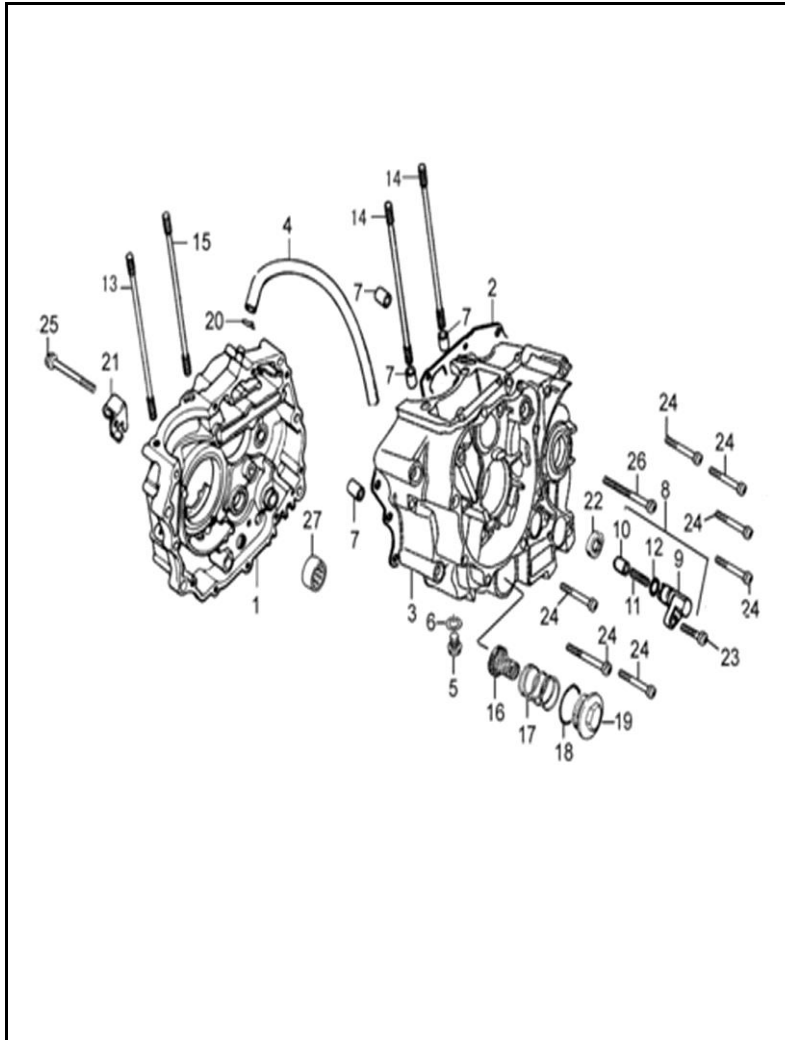
FIGURA N° 8: CARCASAS (1/2)
