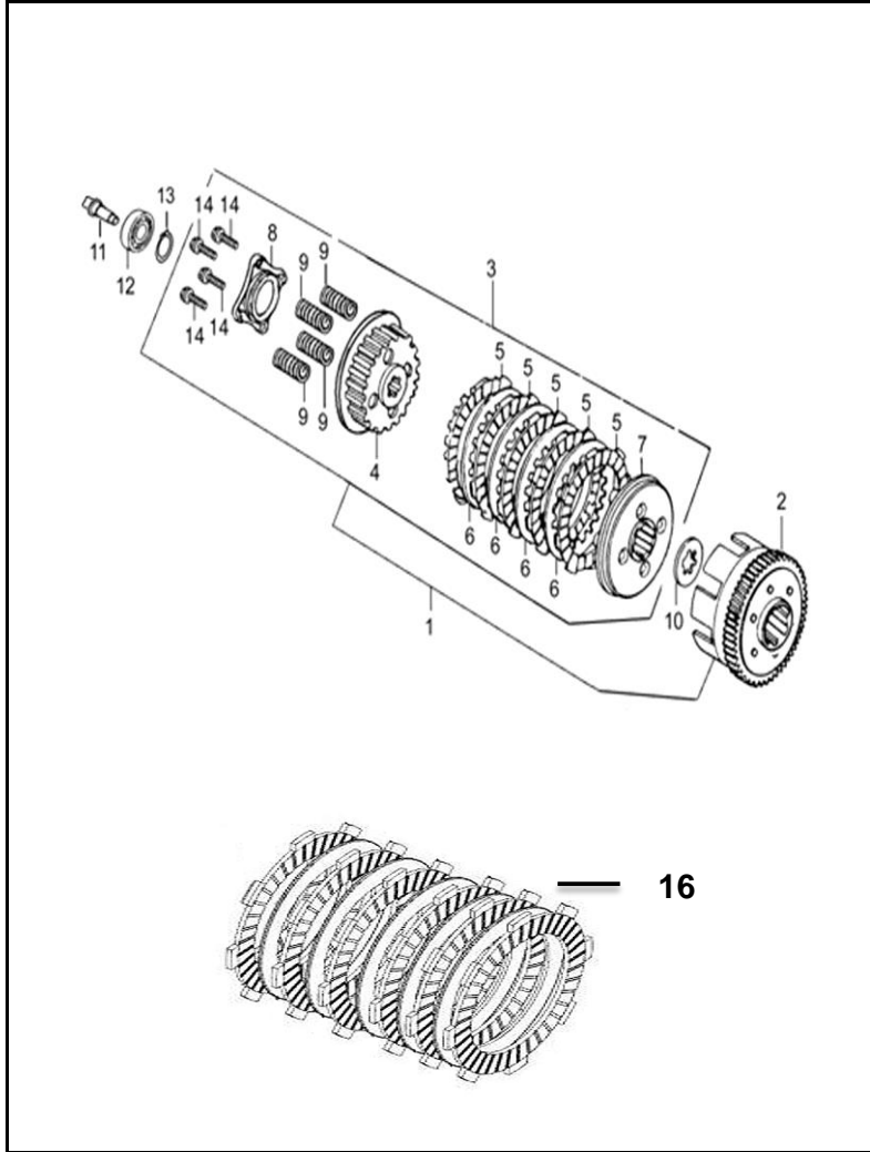
FIGURA N° 4: CLUTCH (5 DISCOS)
