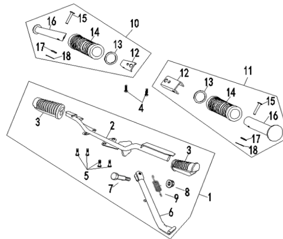
FIG. Nº 38 REPOSAPIE CONDUCTOR - REPOSAPIE PASAJERO - GATO LATERAL
