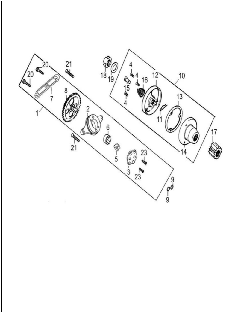
FIGURA N° 7: BOMBA ACEITE - FILTRO CENTRIFUGO ACEITE
