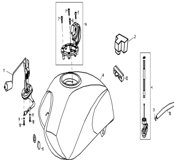
FIG. Nº 29 TANQUE GASOLINA
