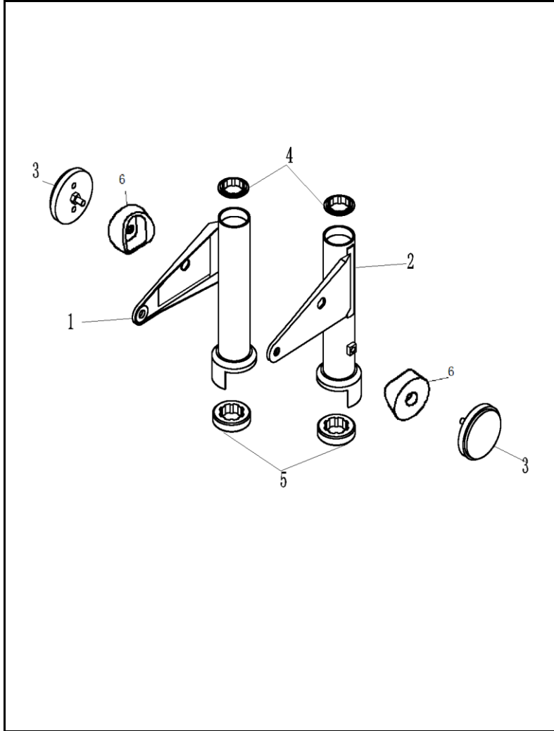
FIGURA N° 23: SOPORTE FAROLA
