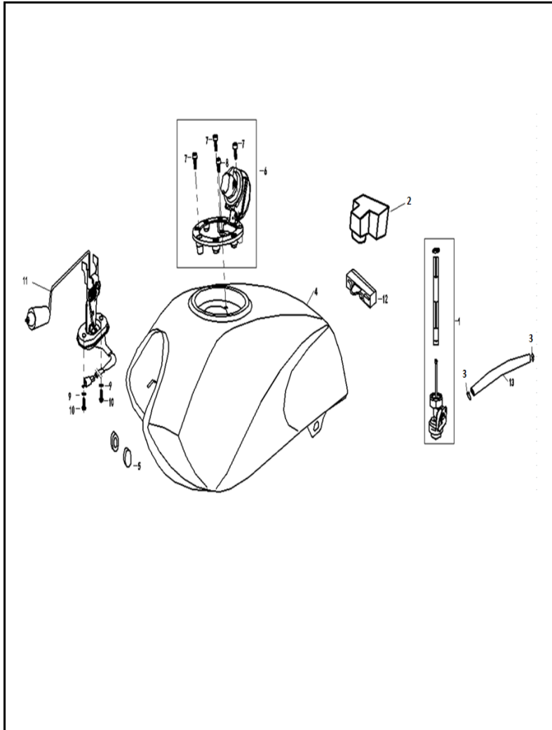
FIGURA N° 29: TANQUE GASOLINA
