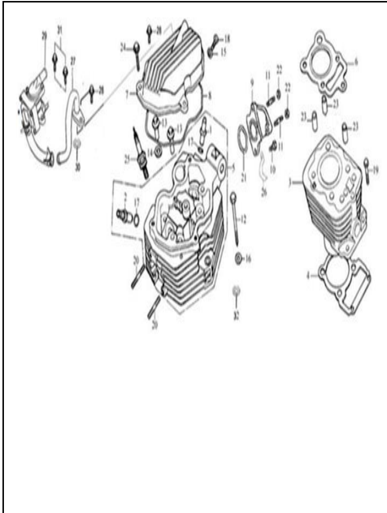
FIGURA N° 1: CULATA - CILINDRO (1/2)
