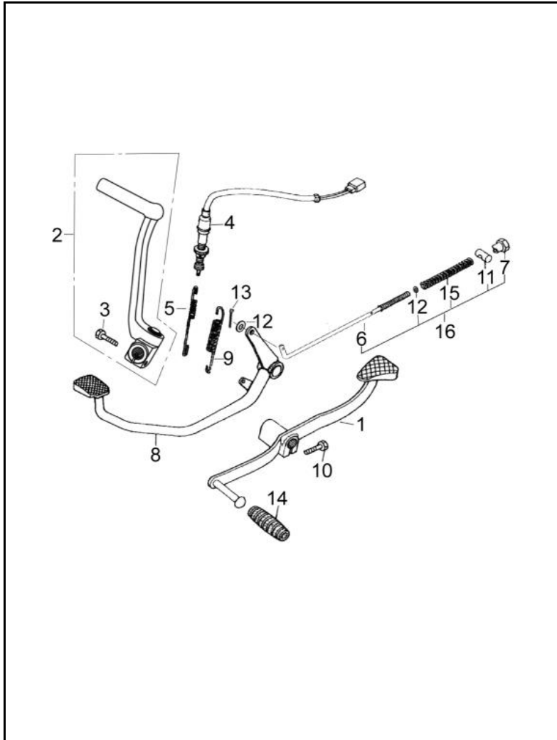
FIGURA N° 13: PEDAL FRENO
