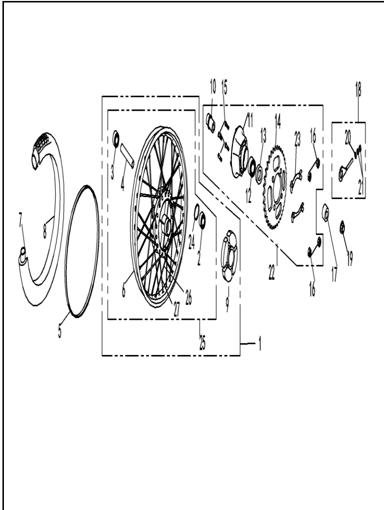
FIGURA N° 36: RUEDA TRASERA (1/2)
