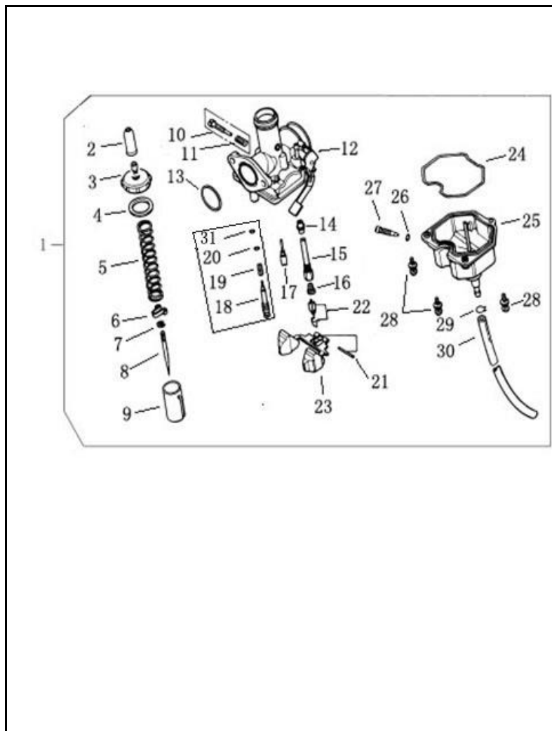
FIGURA N° 14: CARBURADOR (2/2)
