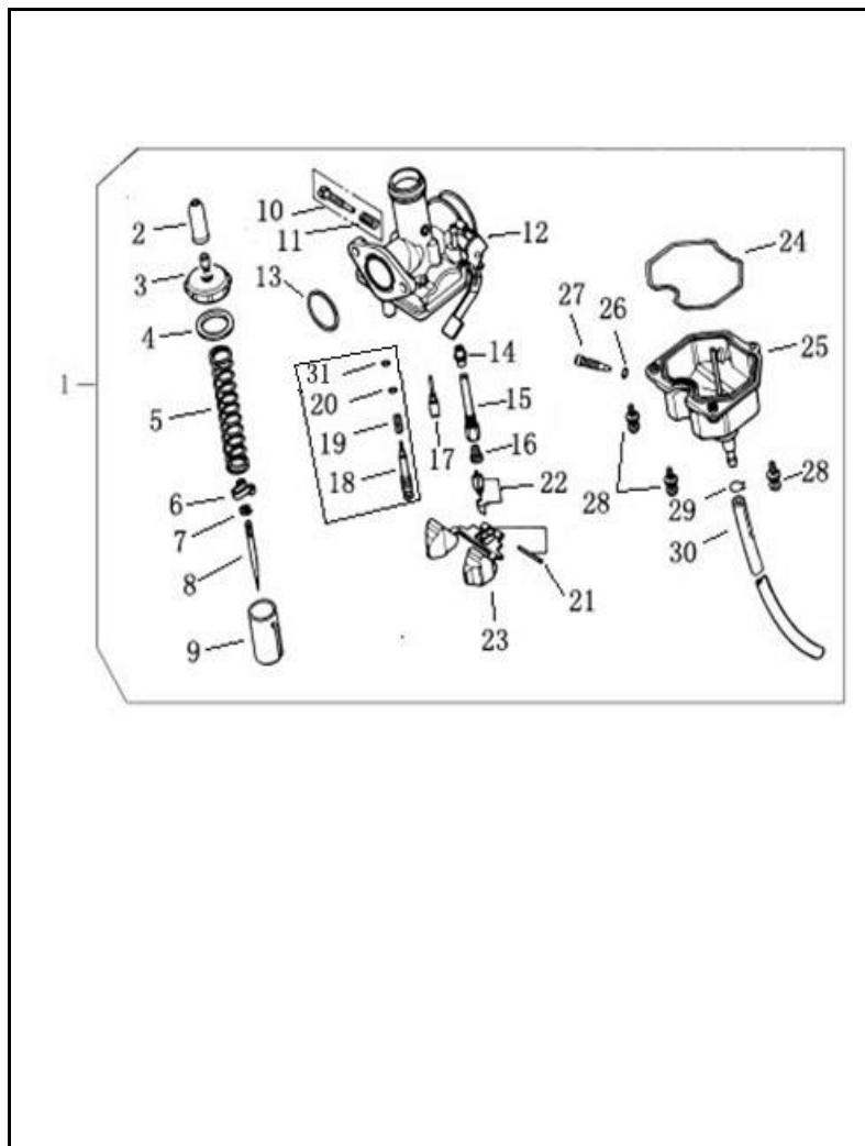
FIGURA N° 14: CARBURADOR (1/2)
