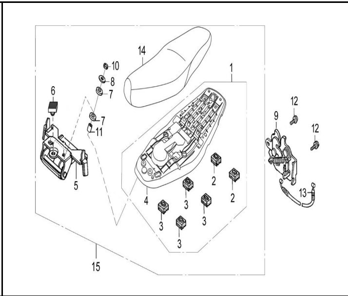
FIG. N° 38 SILLIN
