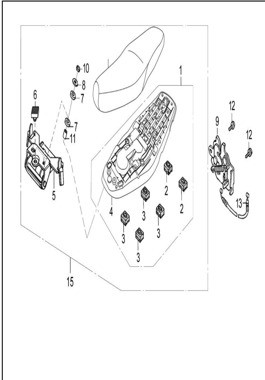
FIGURA N° 38: SILLIN
