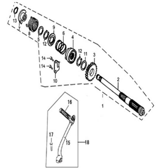
FIG. Nº 15 PEDAL CRANK
