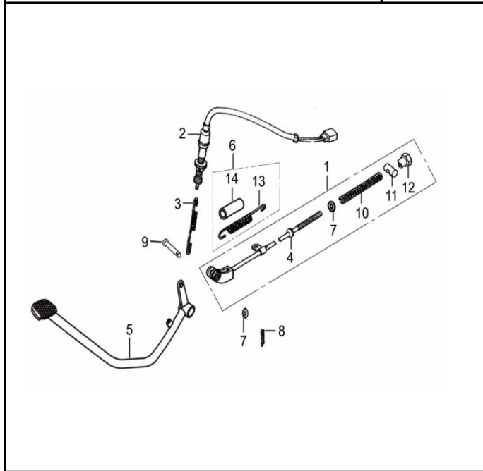
FIG. N° 40 PEDAL FRENO
