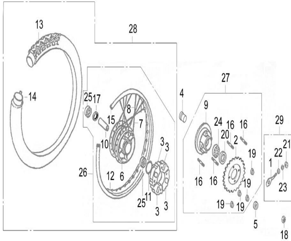
FIG. Nº 31 RUEDA TRASERA (RIN DE RADIOS)
