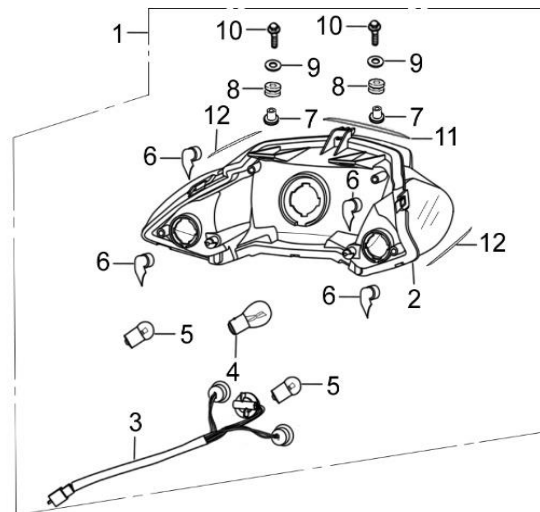
FIG. Nº 47 STOP
