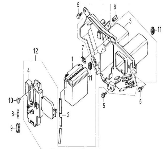
FIG. Nº 48 BATERIA - CAJA BATERIA
