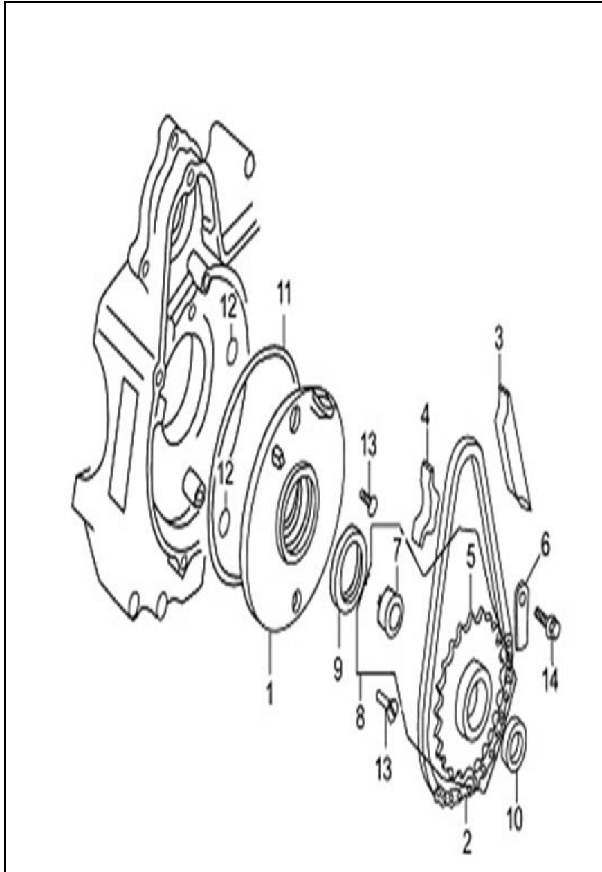
FIGURA N° 10: CADENILLA MOTOR DE ARRANQUE
