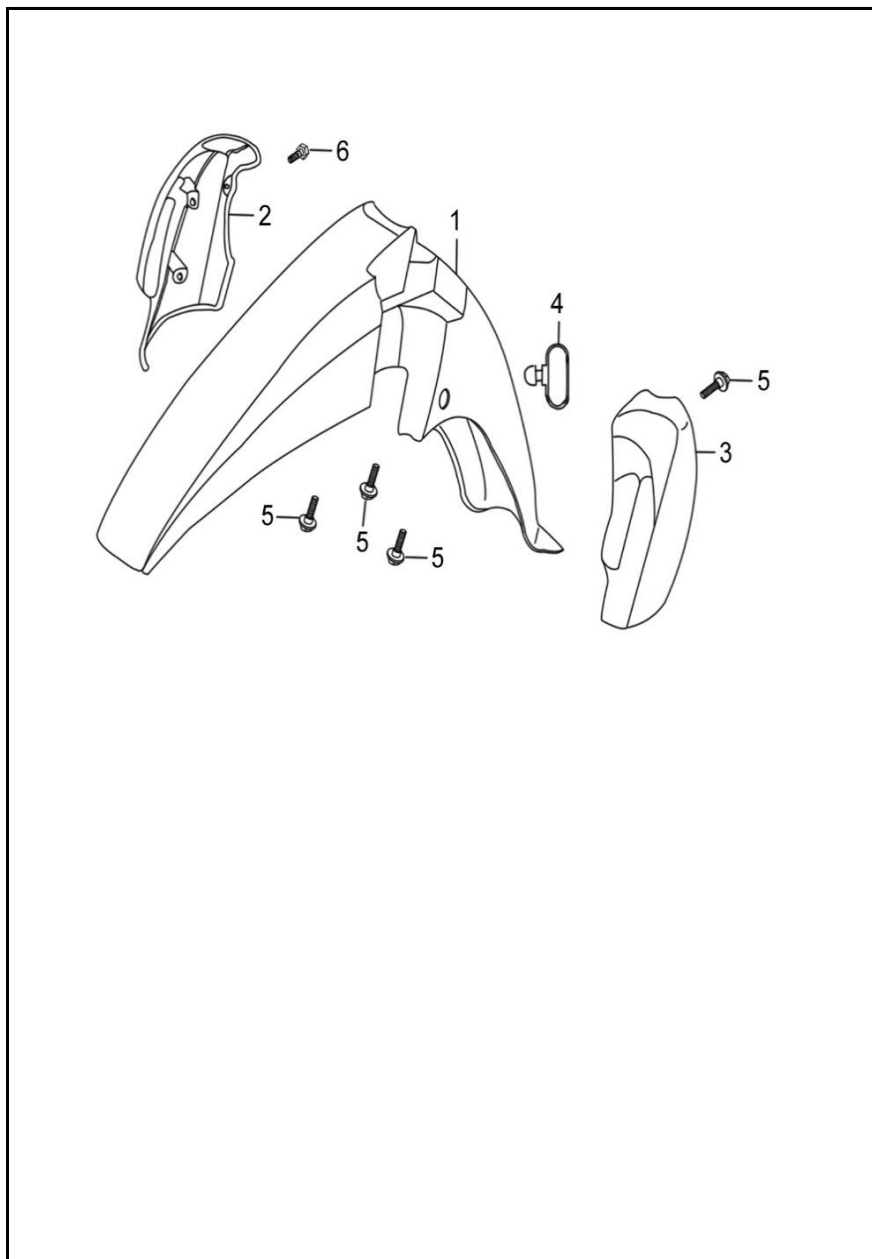
FIGURA N° 26: GUARDABARRO DELANTERO
