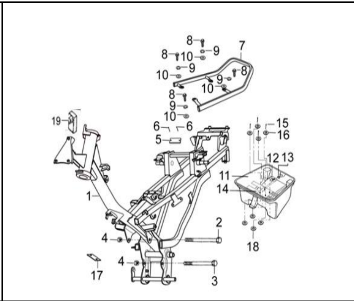
FIG. Nº 50 COMPLEMENTOS CHASIS
