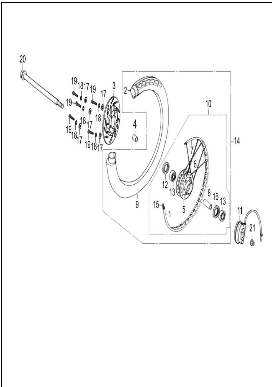
FIGURA N° 28: RUEDA DELANTERA (RIN DE RADIOS)
