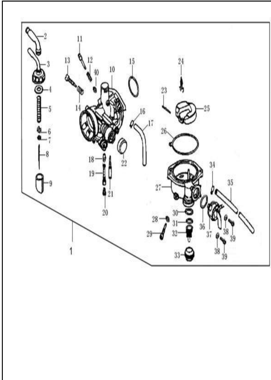
FIGURA N° 17: CARBURADOR 2/2
