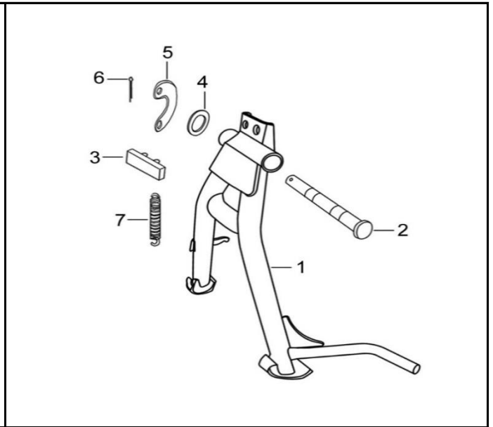
FIG. N° 39 GATO CENTRAL
