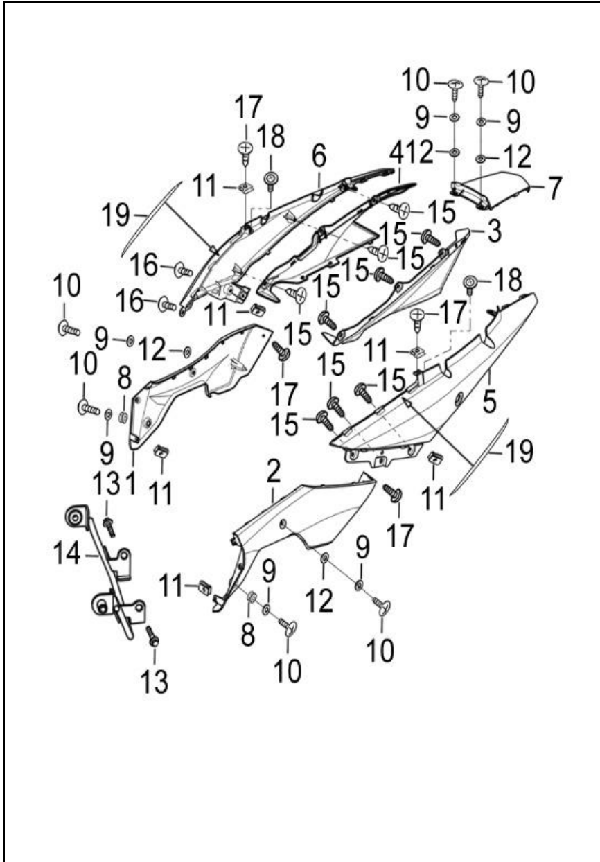
FIGURA N° 45: CUBIERTAS LATERALES
