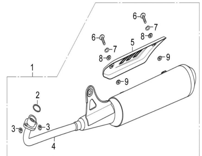
FIG. Nº 36 SILENCIADOR
