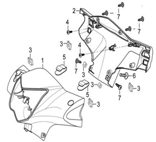
FIG. Nº 21 CUBIERTAS MANUBRIO
