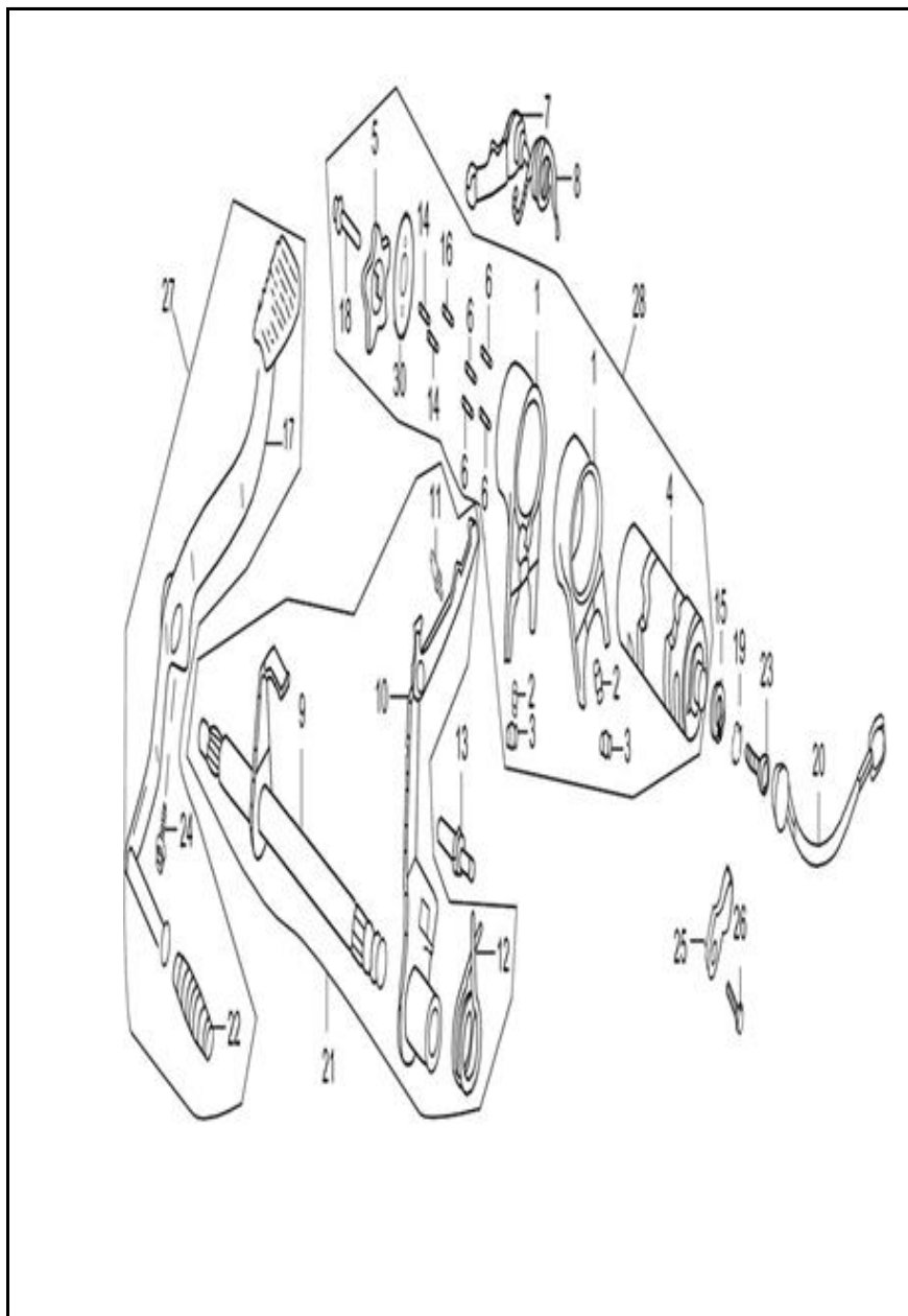
FIGURA N° 16: EJE DE CAMBIOS - SELECTOR DE CAMBIOS 2/2
