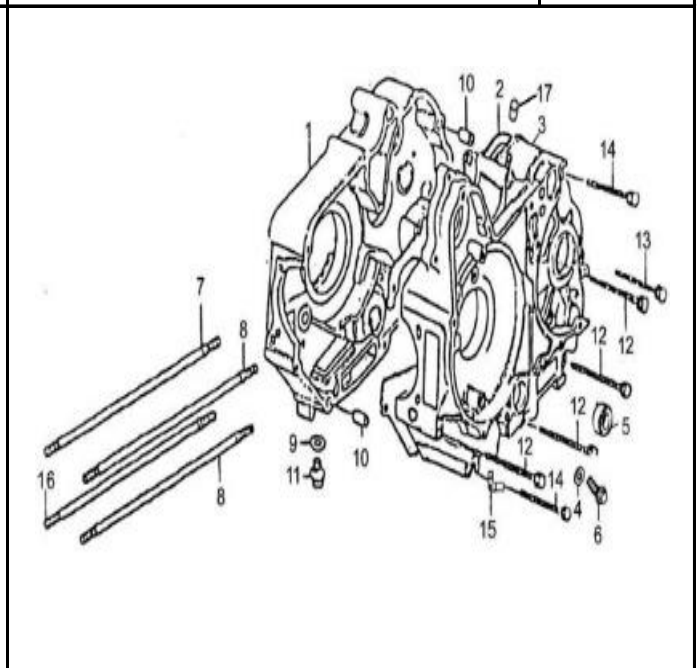
FIG. Nº 12 CARCASAS
