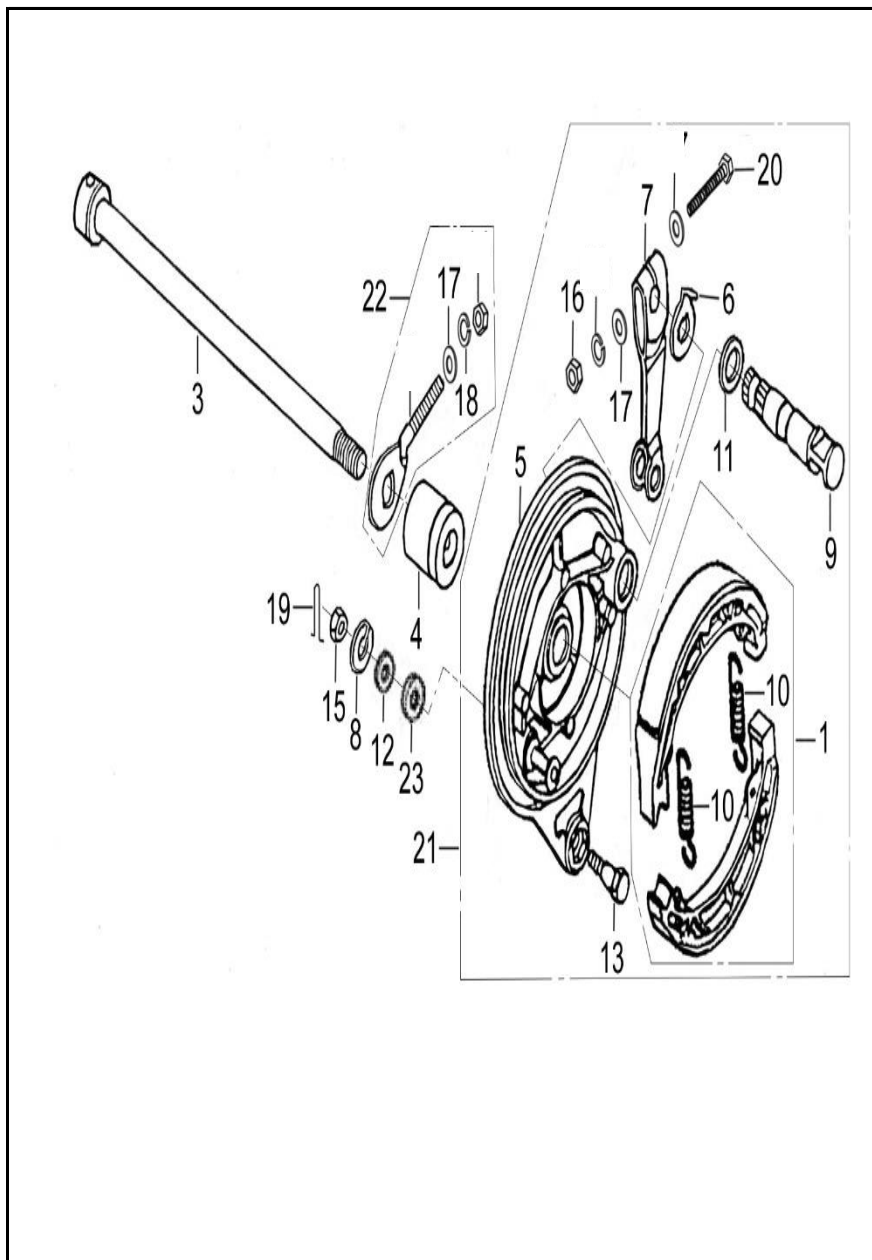
FIGURA N° 33: PORTABANDAS RUEDA TRASERA (RIN DE ASPAS & RADIOS)
