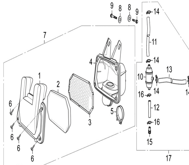
FIG. Nº 35 FILTRO DE AIRE - FILTRO DE GASOLINA
