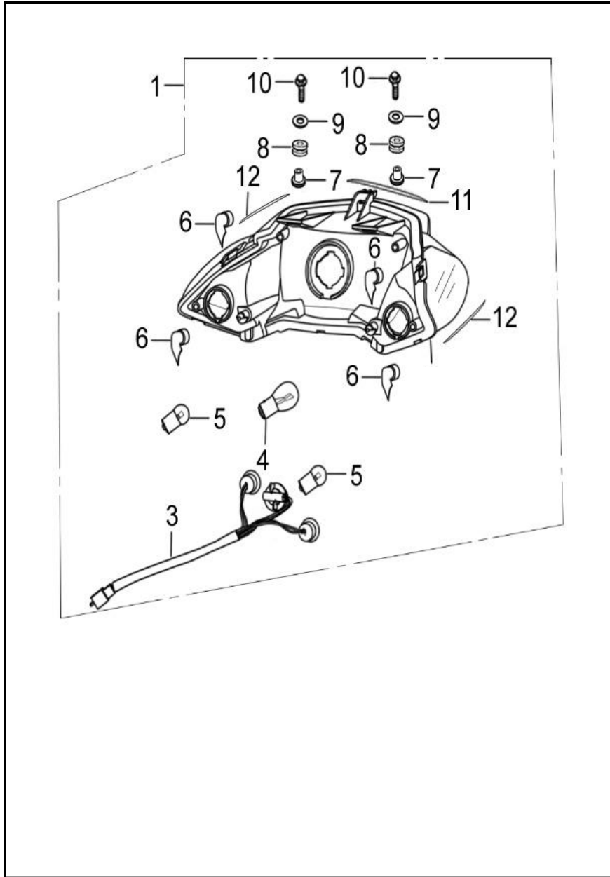
FIGURA N° 47: STOP
