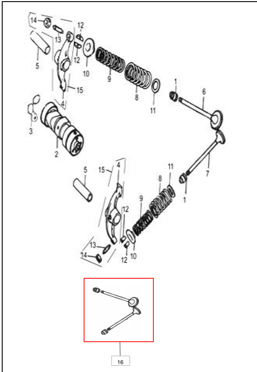
FIGURA N° 3: EJE DE LEVAS - VALVULAS
