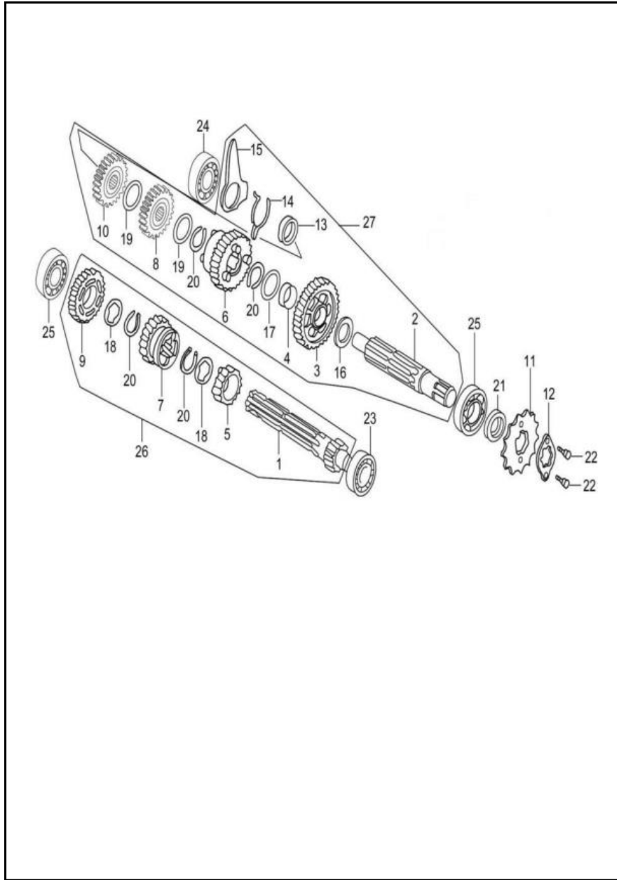
FIGURA N° 14: TRANSMISION
