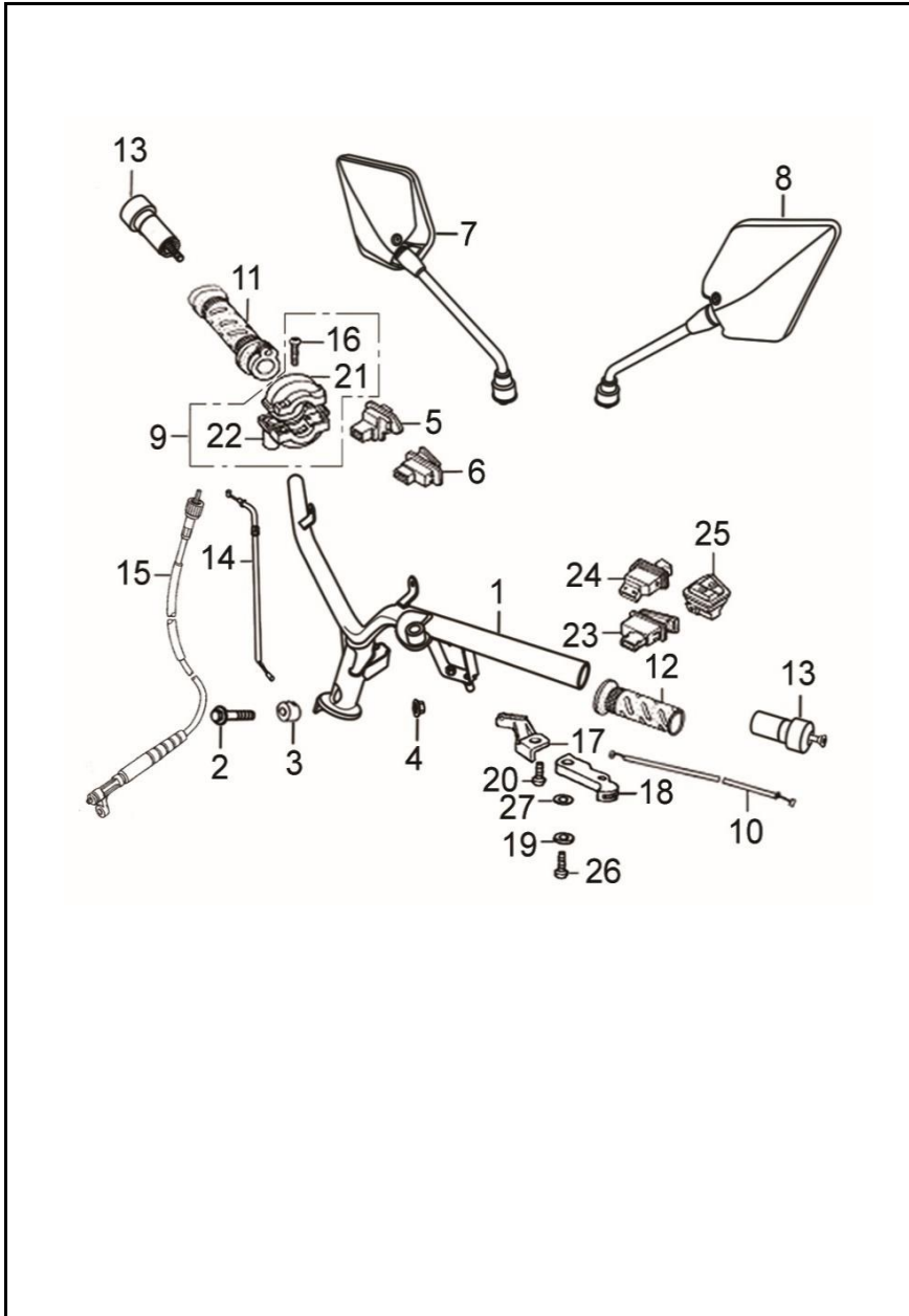
FIGURA N° 24: MANUBRIO - ESPEJOS 2/2
