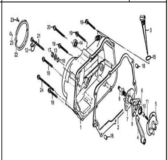
FIG. Nº 6 CUBIERTA CLUTCH
