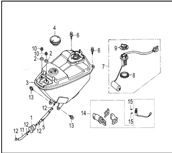
FIG. N° 37 TANQUE GASOLINA
