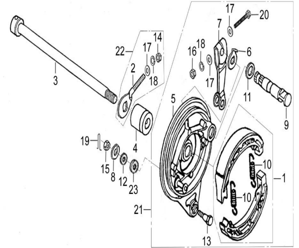
FIG. Nº 33 PORTABANDAS RUEDA TRASERA (RIN DE ASPAS & RADIOS)
