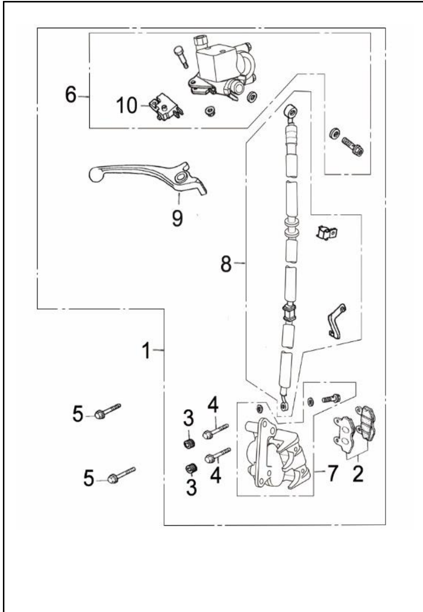
FIGURA N° 30: BOMBA DE FRENO - CALIPER DELANTERO
