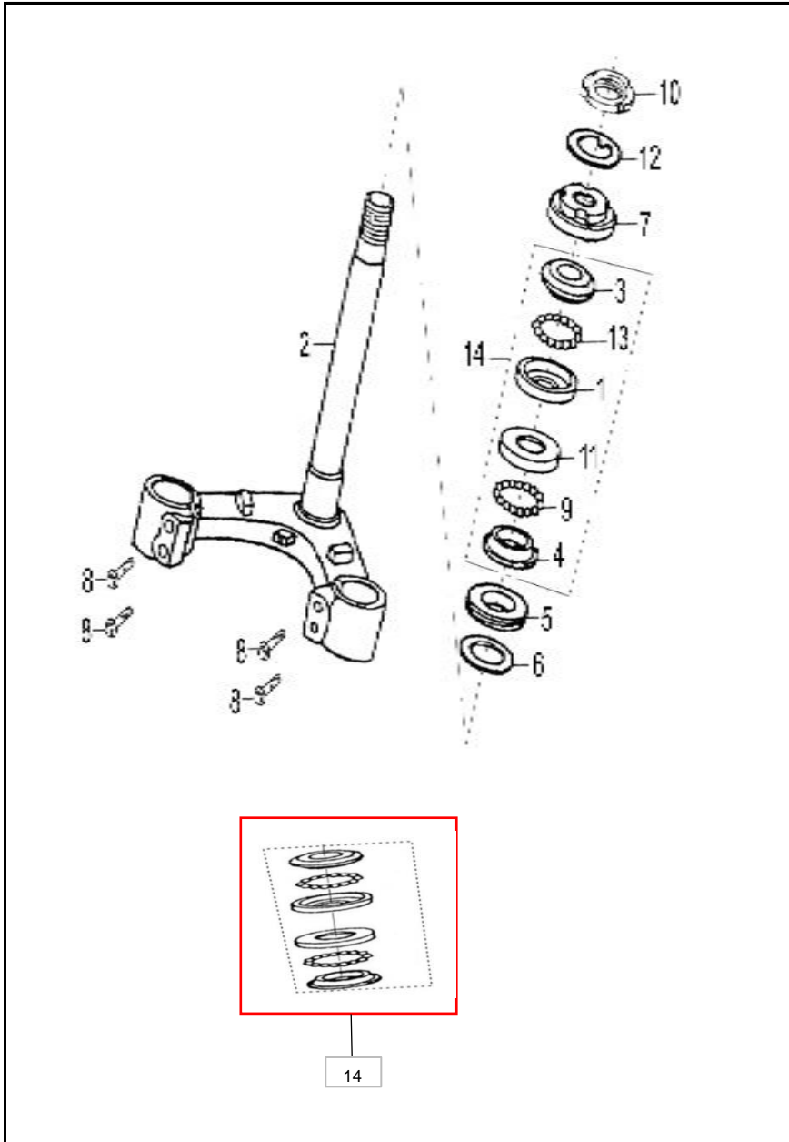
FIGURA N° 25: ESPIGA CENTRAL
