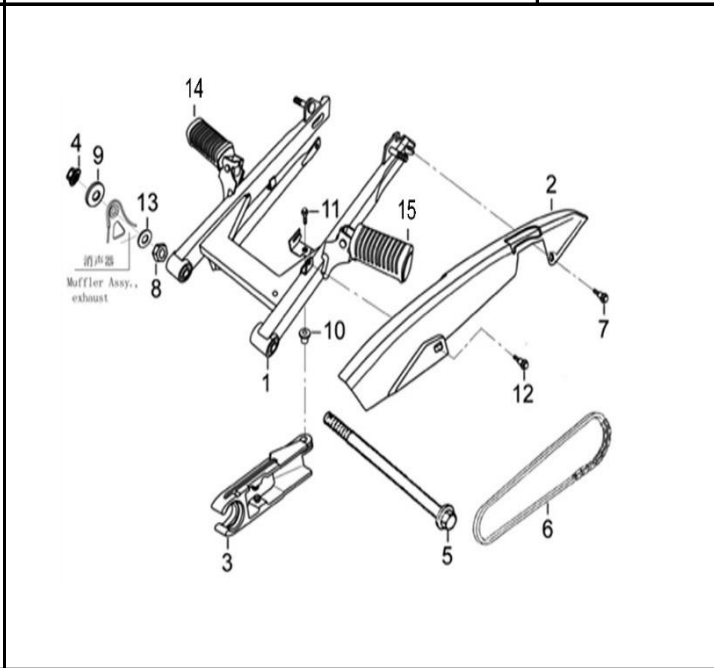
FIG. N° 41 BRAZO OSCILANTE
