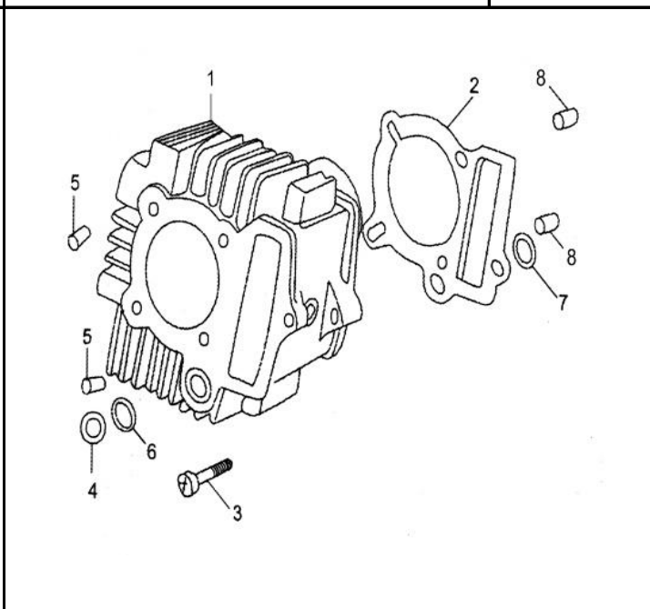
FIG. Nº 5 CILINDRO
