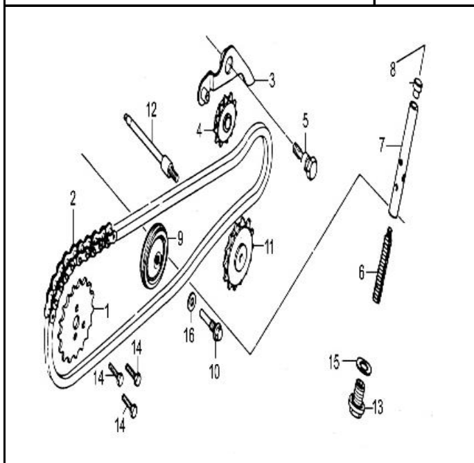
FIG. Nº 4 CADENILLA DISTRIBUCION
