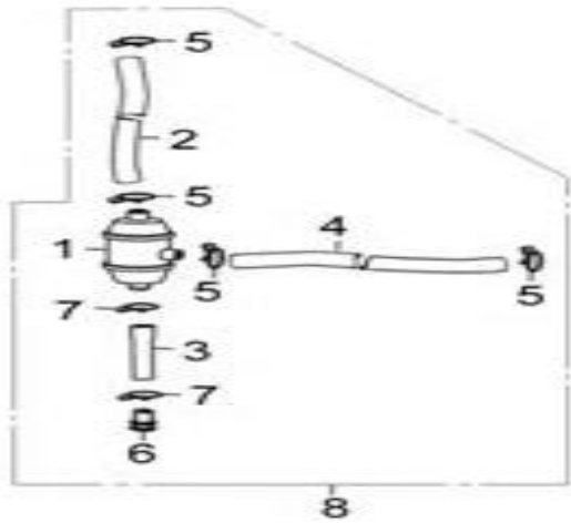
FIG. Nº 19 FILTRO DE GASOLINA
