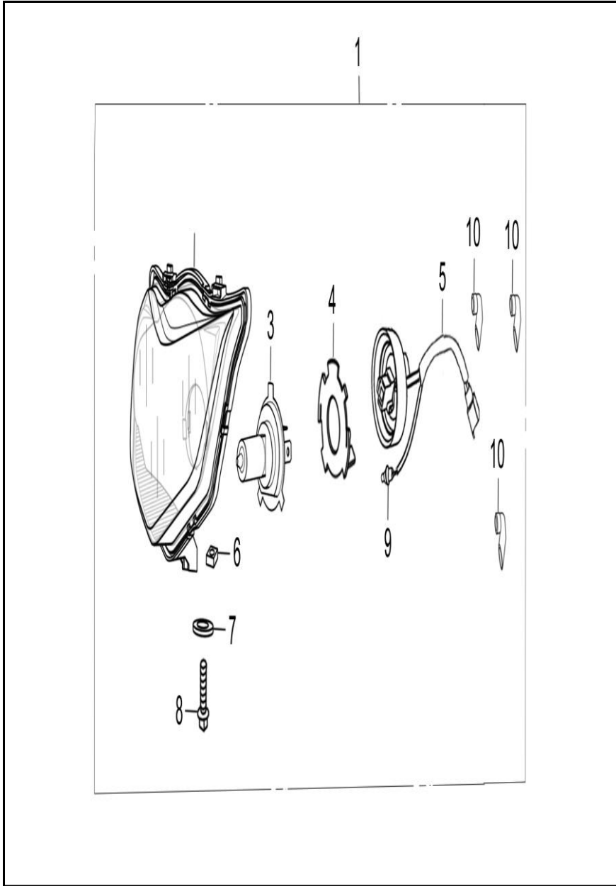
FIGURA N° 20: FAROLA
