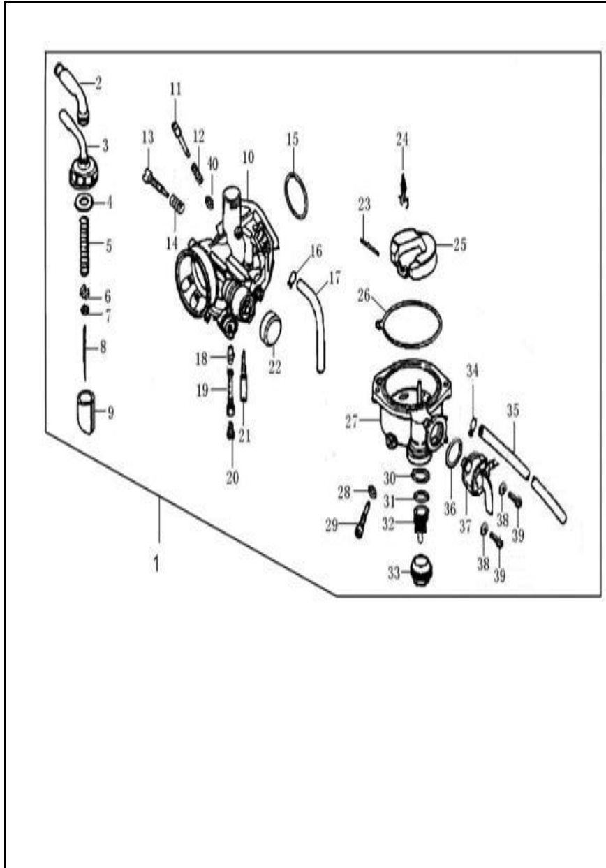
FIGURA N° 17: CARBURADOR 1/2
