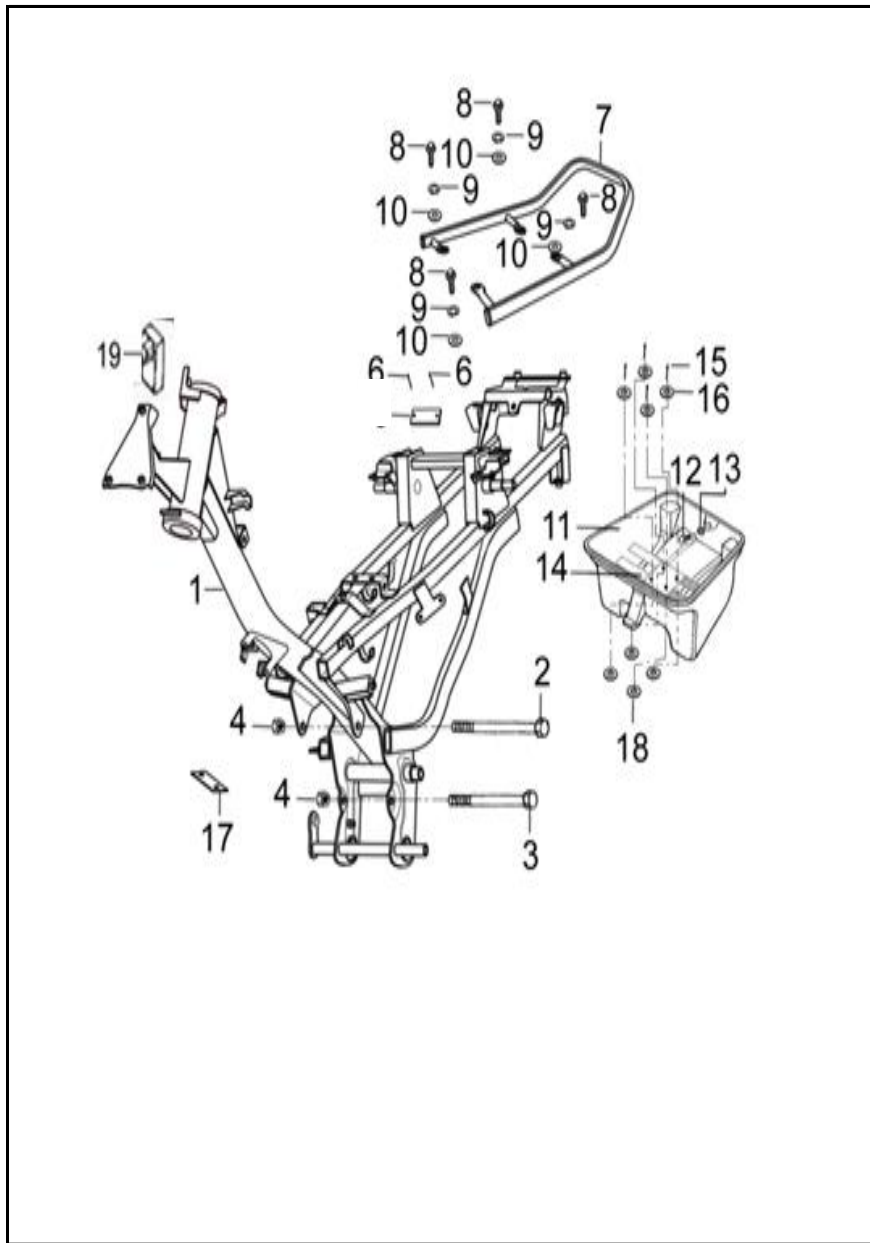
FIGURA N° 50: COMPLEMENTOS CHASIS
