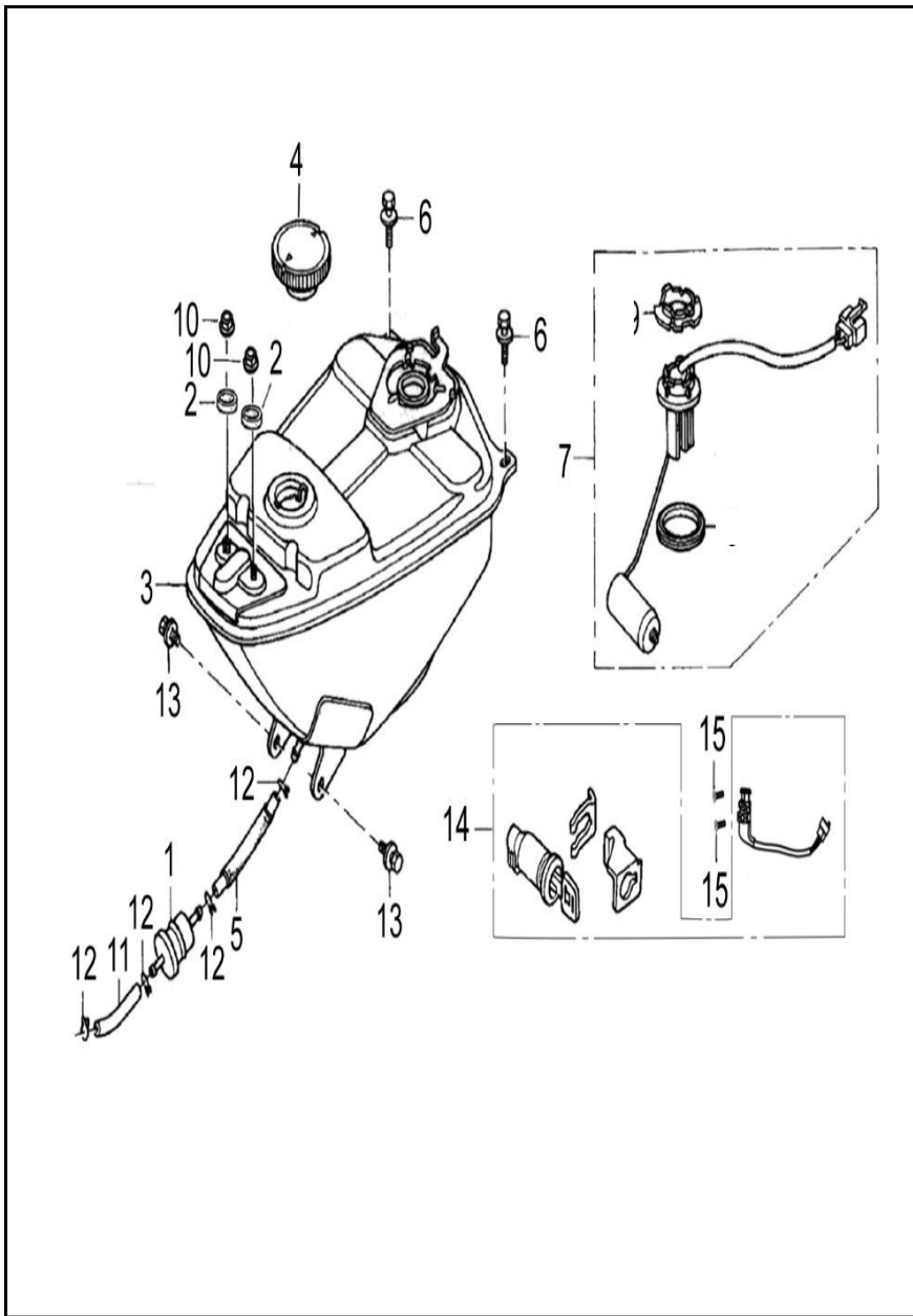
FIGURA N° 37: TANQUE GASOLINA
