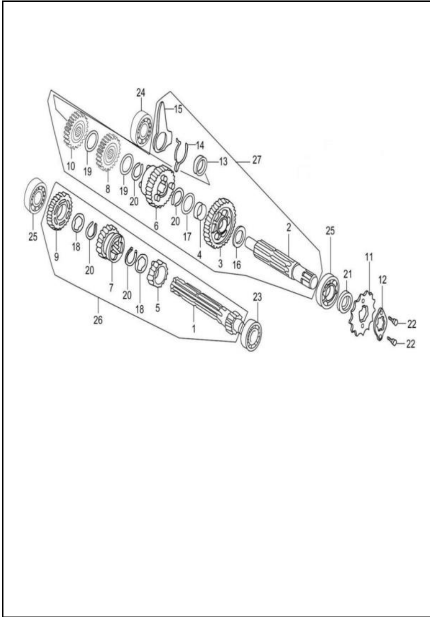
FIGURA N° 14: TRANSMISION
