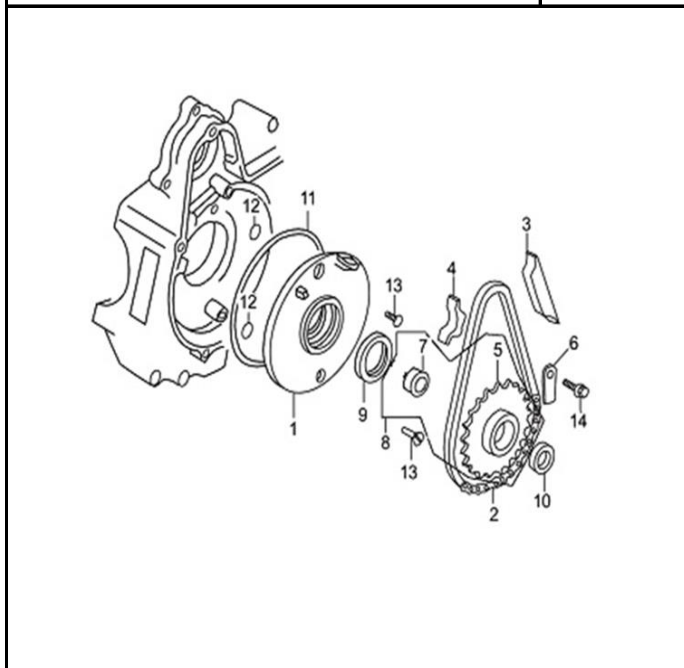
FIG. Nº 10 CADENILLA MOTOR DE ARRANQUE
