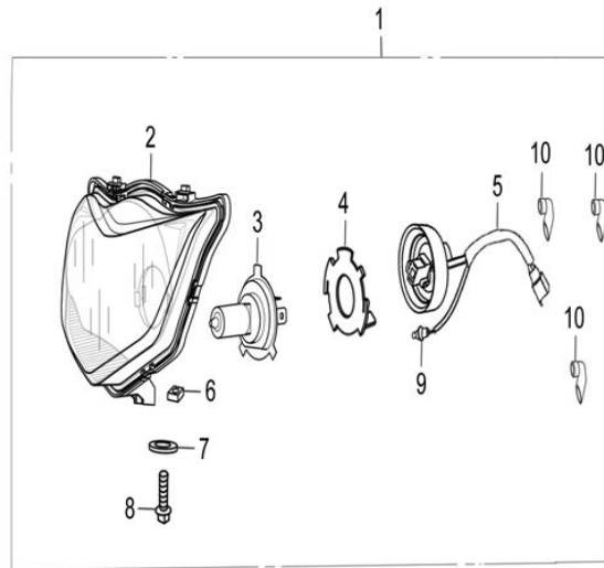
FIG. Nº 20 FAROLA
