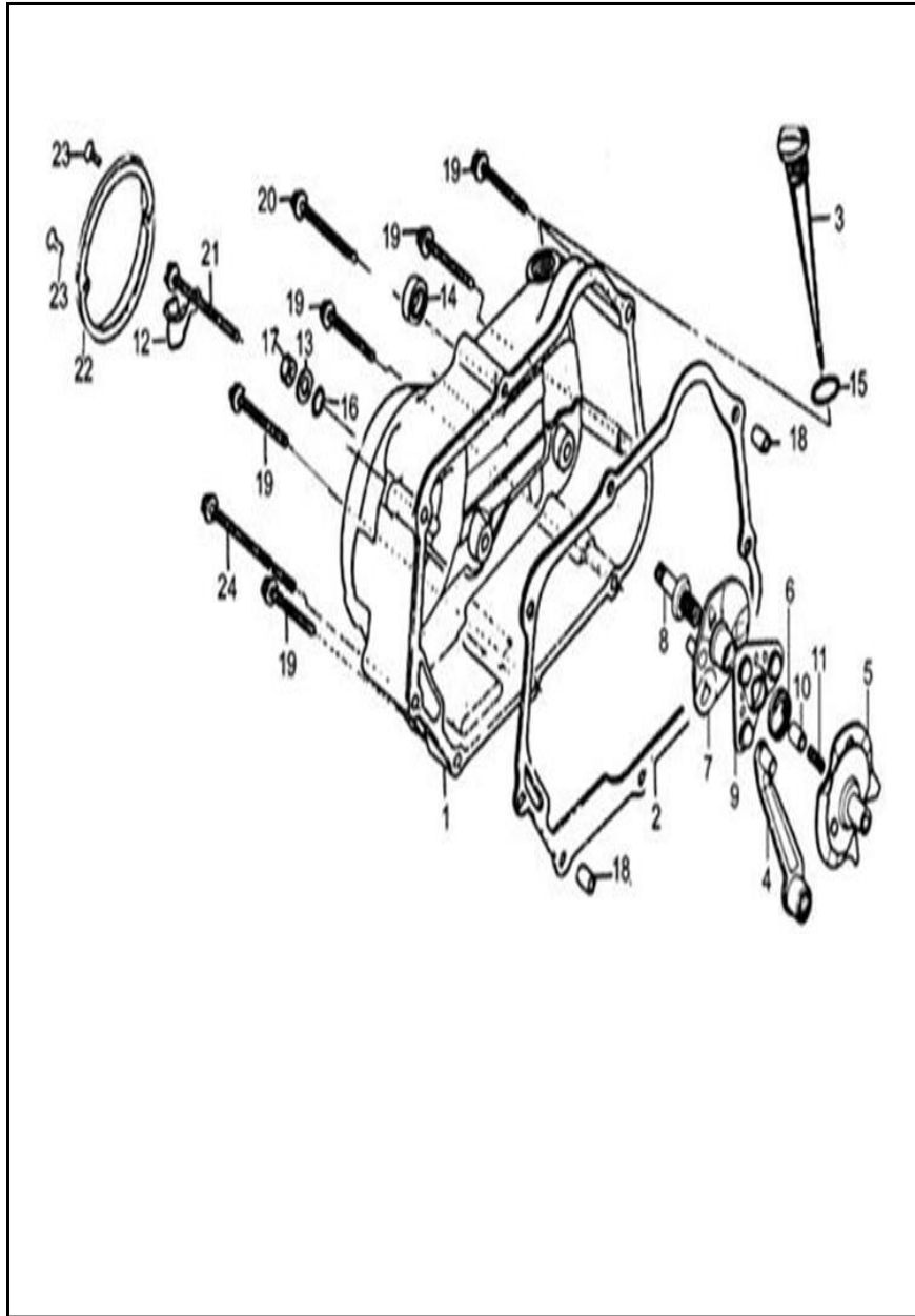
FIGURA N° 6: CUBIERTA CLUTCH
