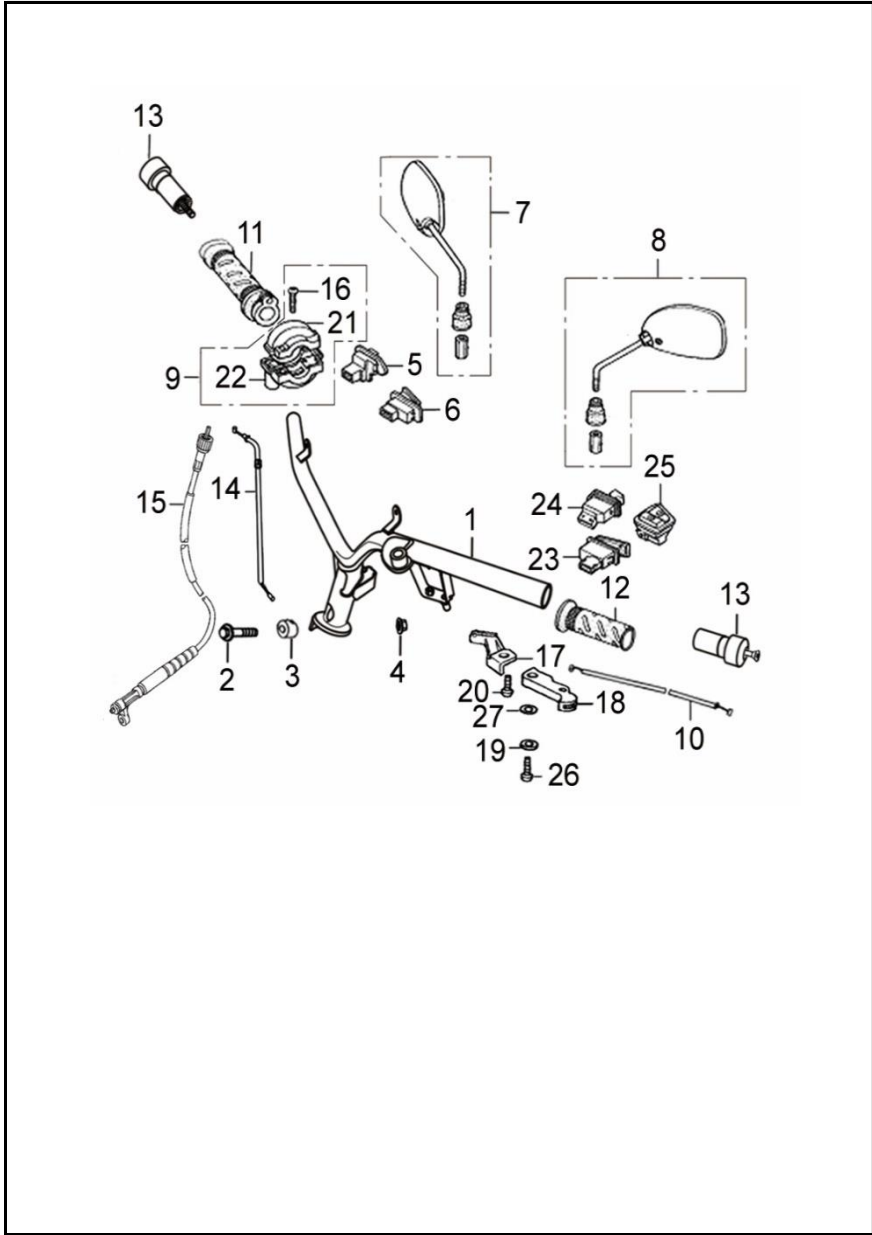
FIGURA N° 23: MANUBRIO - ESPEJOS 2/2
