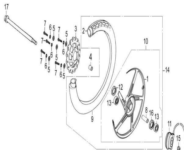
FIG. Nº 29 RUEDA DELANTERA (RIN DE ASPAS)
