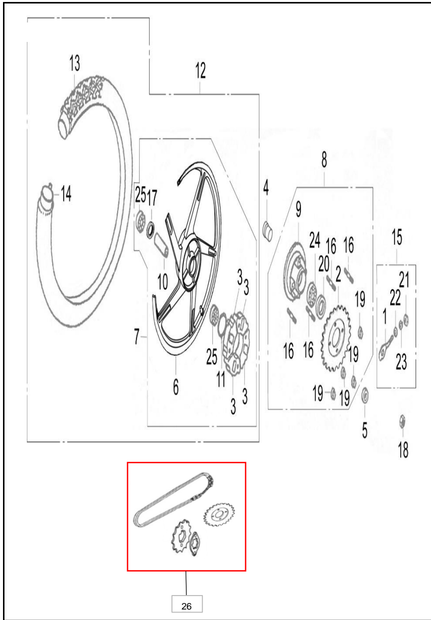
FIGURA N° 32: : RUEDA TRASERA (RIN DE ASPAS)
