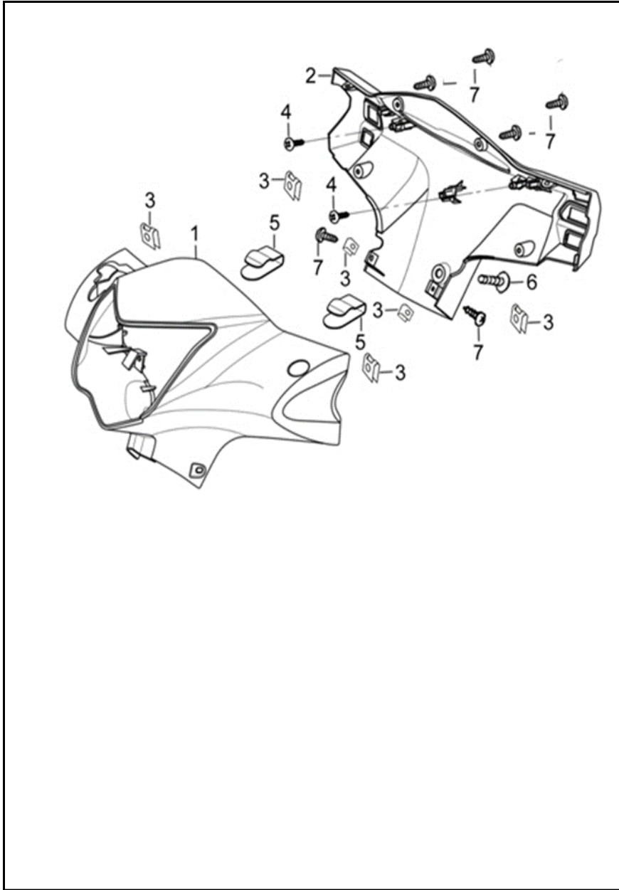
FIGURA N° 21: CUBIERTAS MANUBRIO
