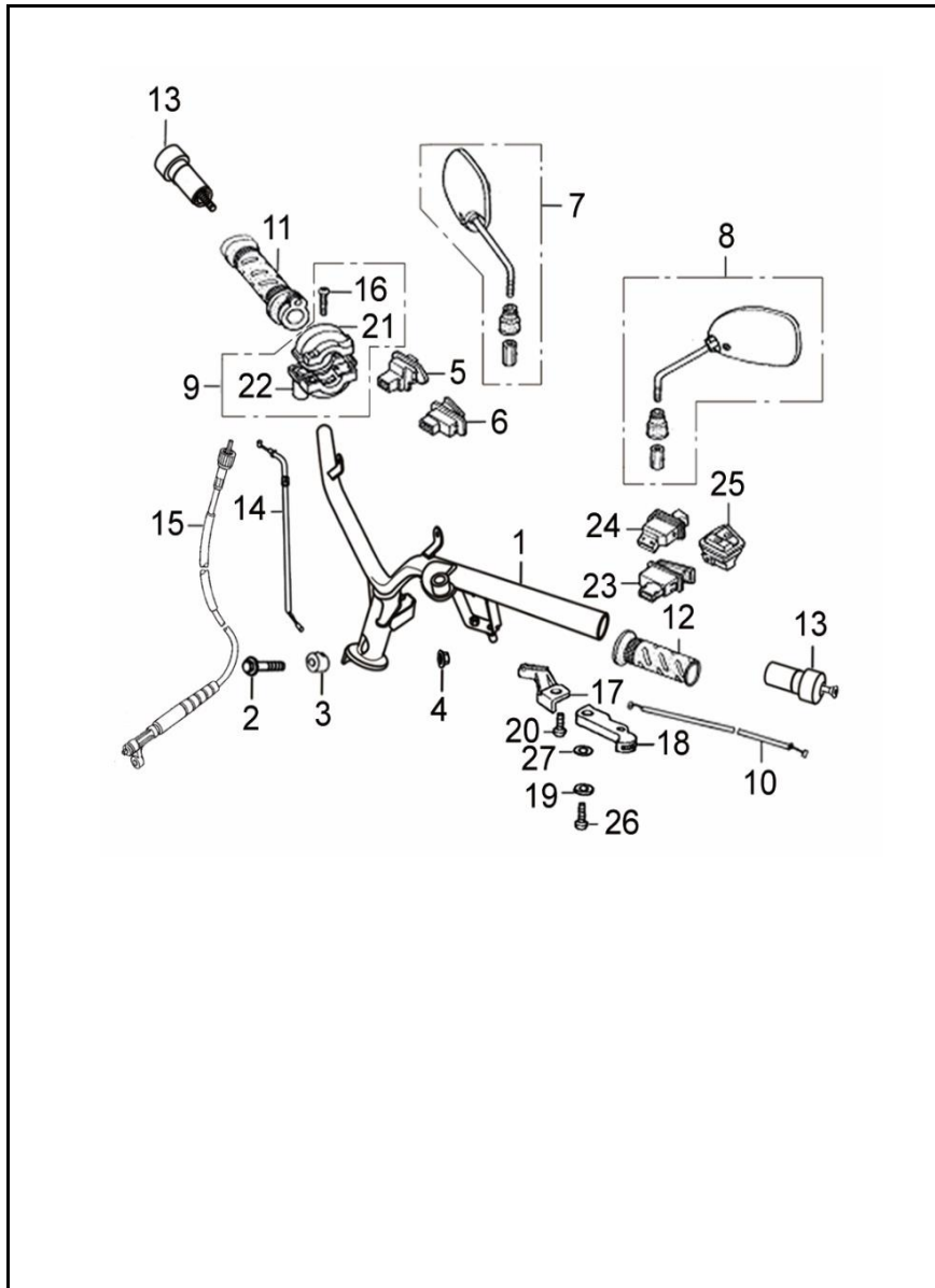
FIGURA N° 23: MANUBRIO - ESPEJOS 1/2
