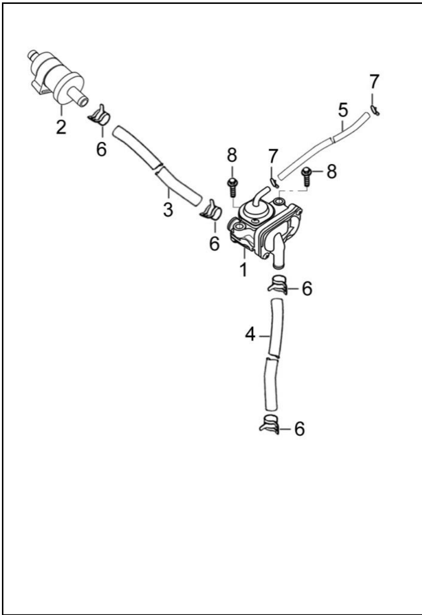
FIGURA N° 51: VALVULA DE GASES
