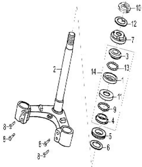
FIG. Nº 25 ESIPIGA CENTRAL
