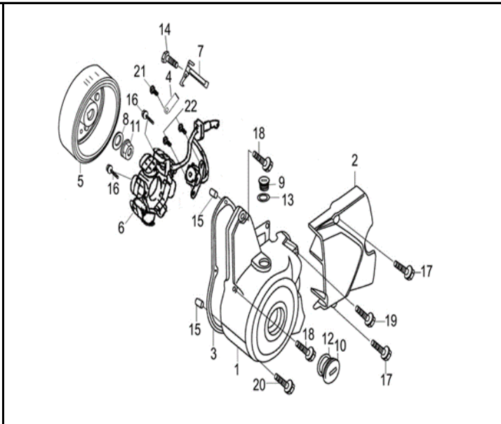
FIG. Nº 8 CUBIERTA VOLANTE - MAGNETO
