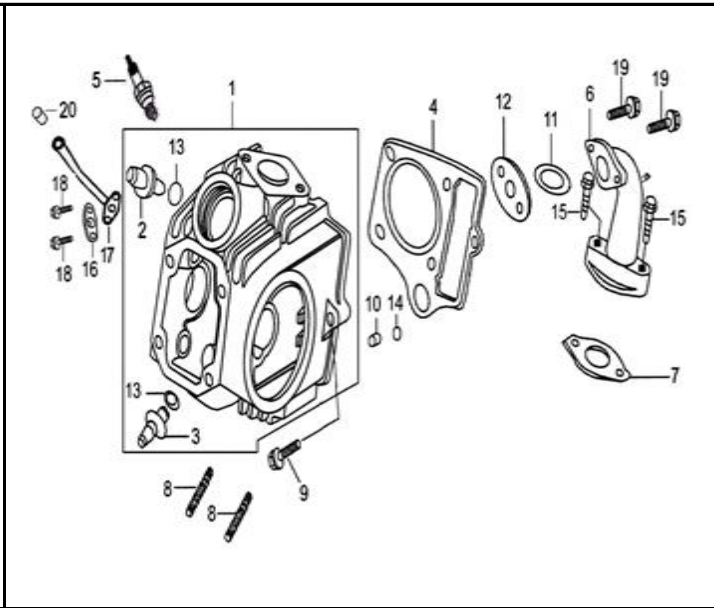
FIG. Nº 2 CULATA
