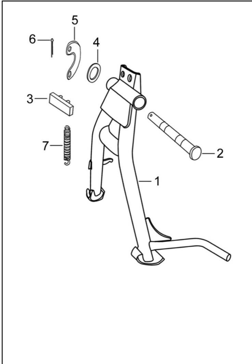
FIGURA N° 39: GATO CENTRAL
