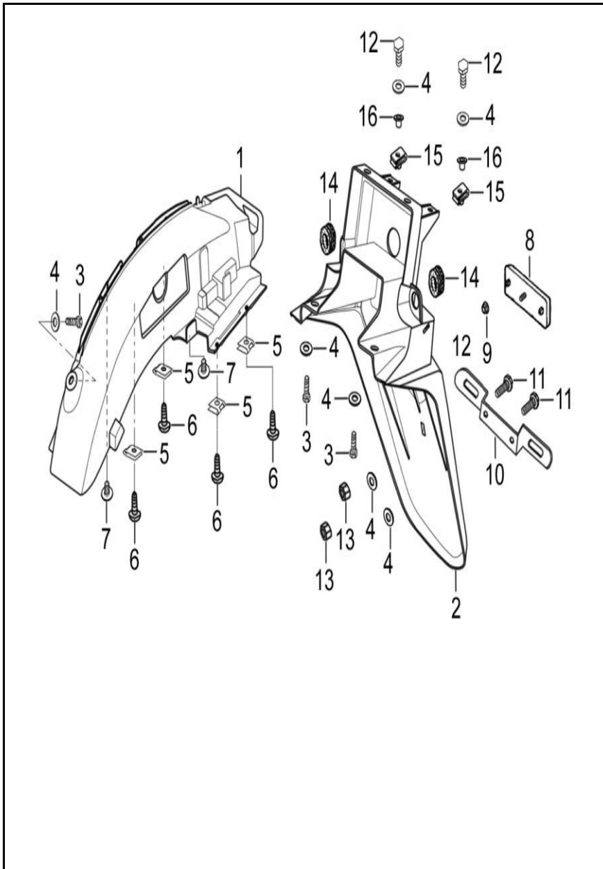
FIGURA N° 46: GUARDABARRO TRASERO
