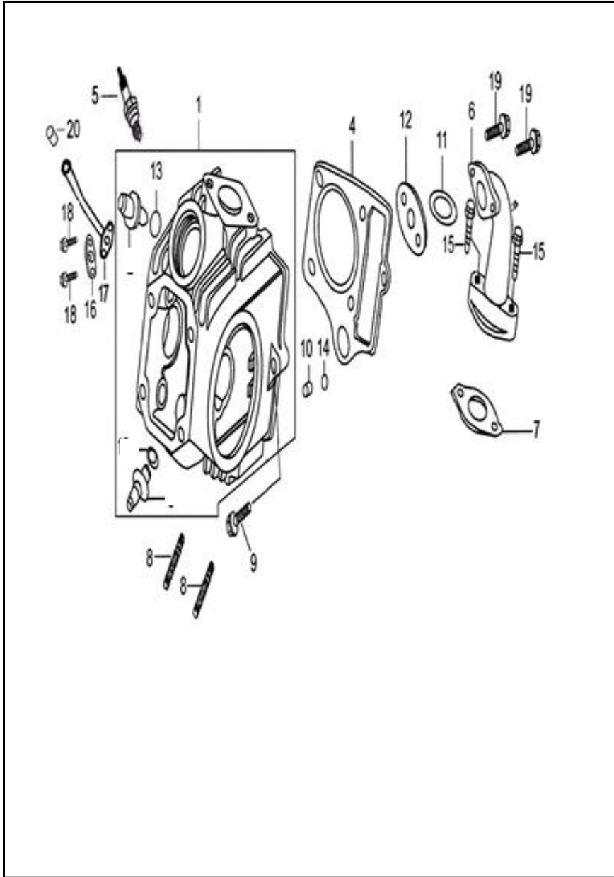
FIGURA N° 2: CULATA
