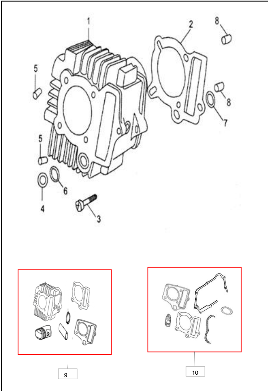
FIGURA N° 5: CILINDRO
