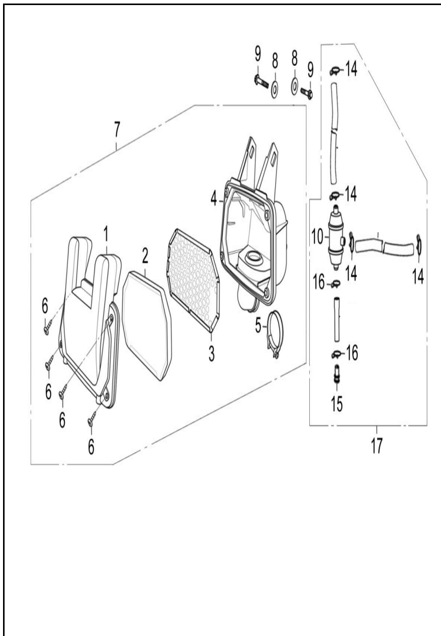
FIGURA N° 35: FILTRO DE AIRE - FILTRO DE GASOLINA
