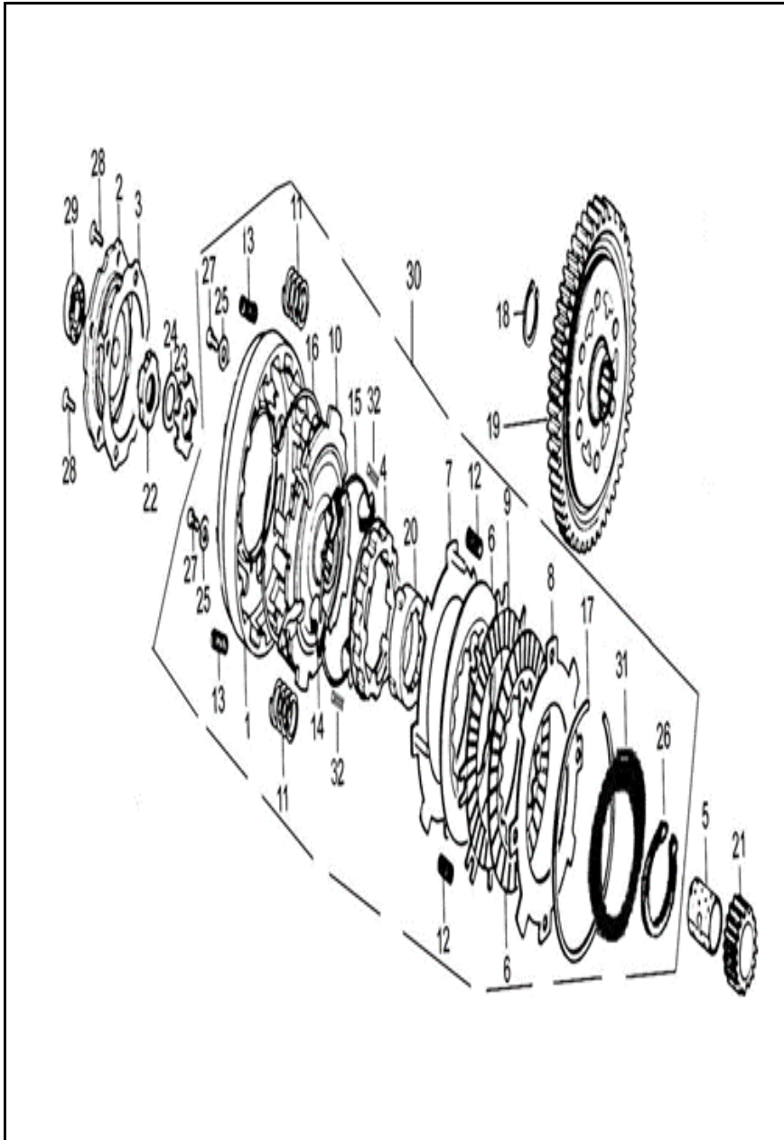
FIGURA N° 7: CLUTCH 1/2
