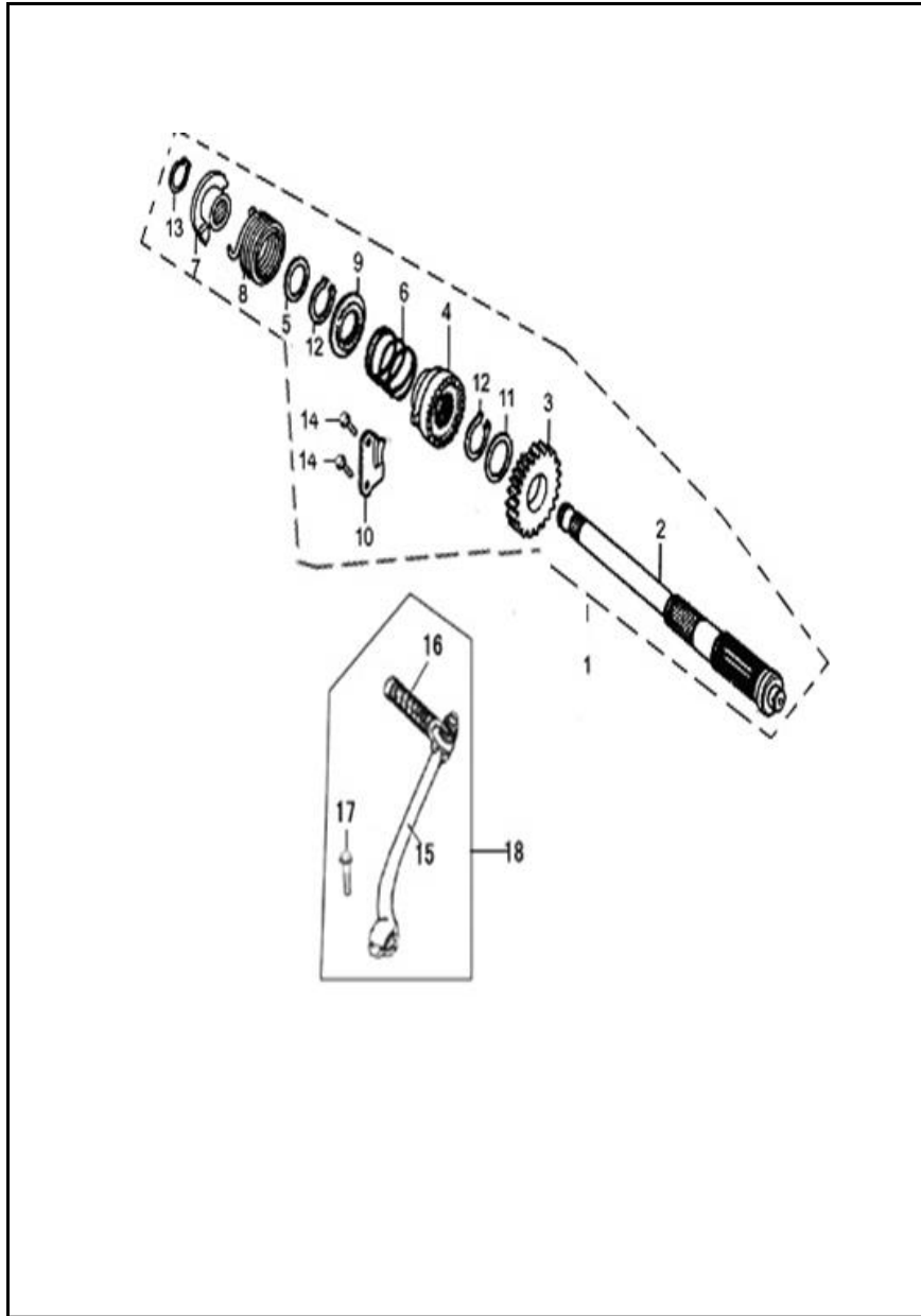
FIGURA N° 15: PEDAL CRANK
