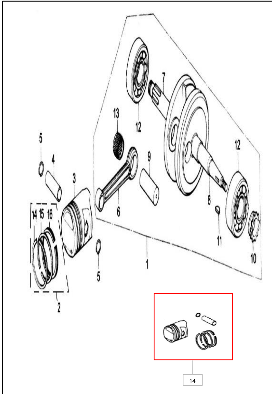
FIGURA N° 13: CIGÜEÑAL - PISTON
