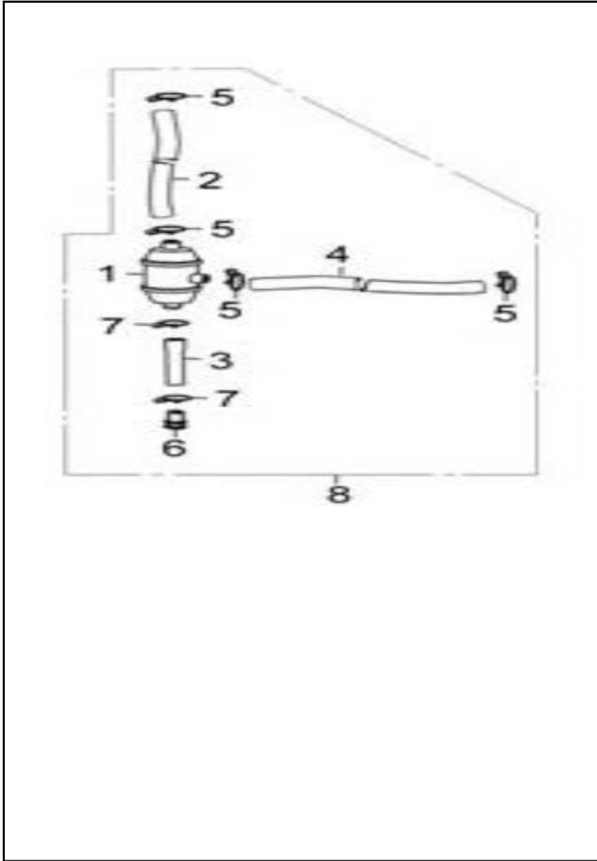
FIGURA N° 19: FILTRO DE GASOLINA
