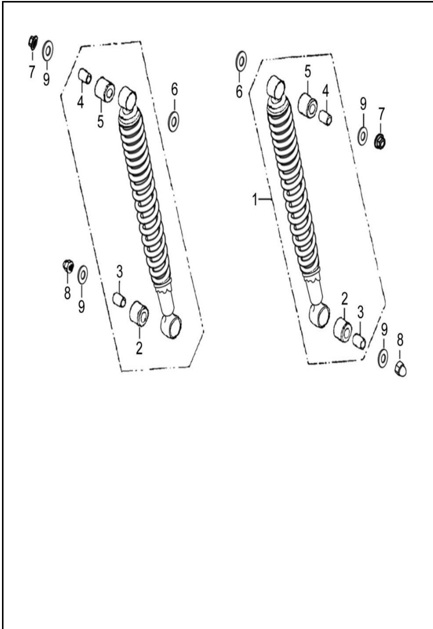
FIGURA N° 42: SUSPENSION TRASERA
