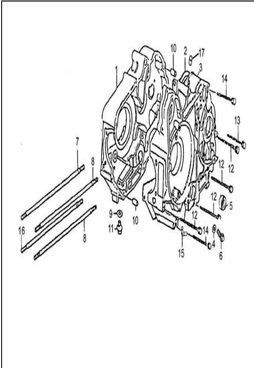
FIGURA N° 12: CARCASAS
