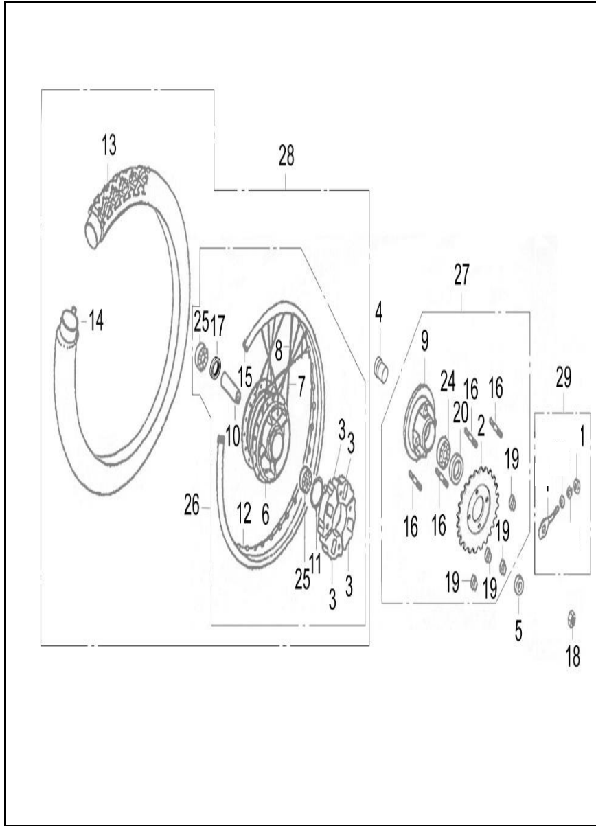
FIGURA N° 31: RUEDA TRASERA (RIN DE RADIOS)
