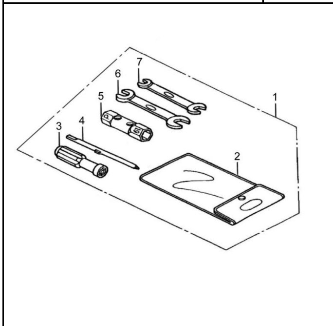
FIG. Nº 52 HERRAMIENTA
