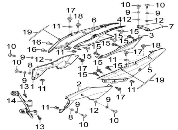
FIG. Nº 45 CUBIERTAS LATERALES
