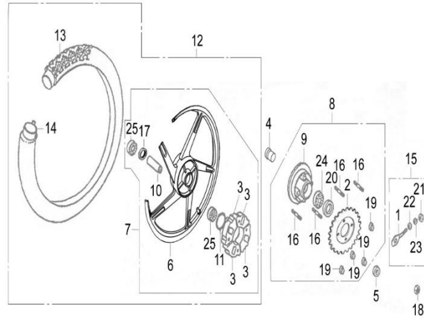
FIG. Nº 32 RUEDA TRASERA (RIN DE ASPAS)
