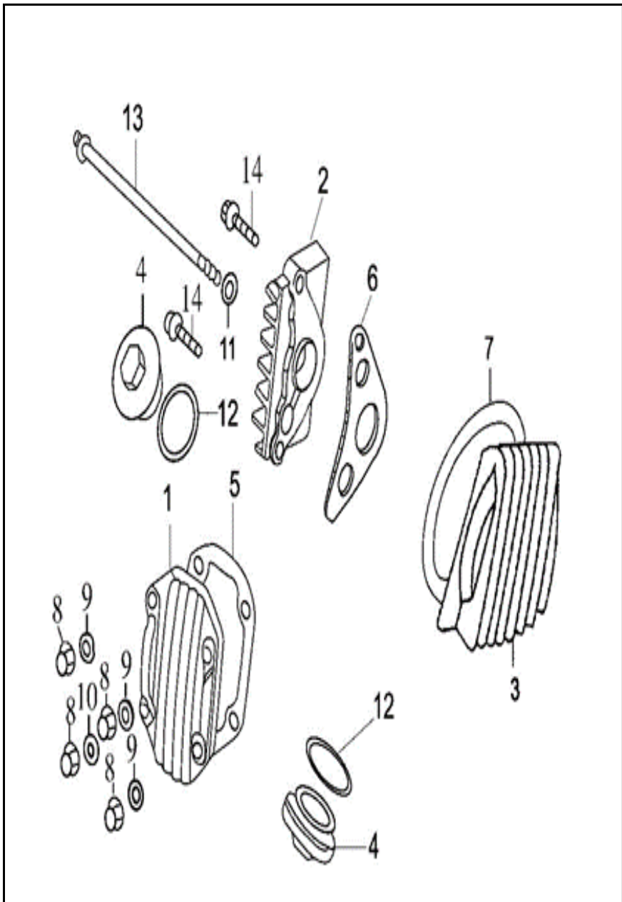
FIGURA N° 1: TAPA CULATA
