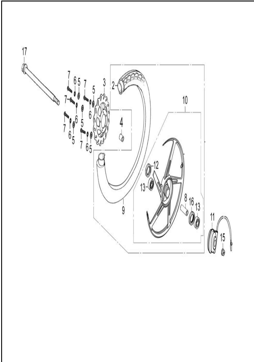
FIGURA N° 29: RUEDA DELANTERA (RIN DE ASPAS)
