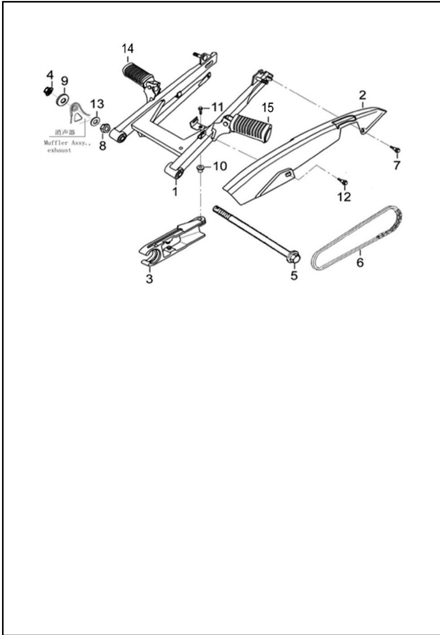
FIGURA N° 41: BRAZO OSCILANTE
