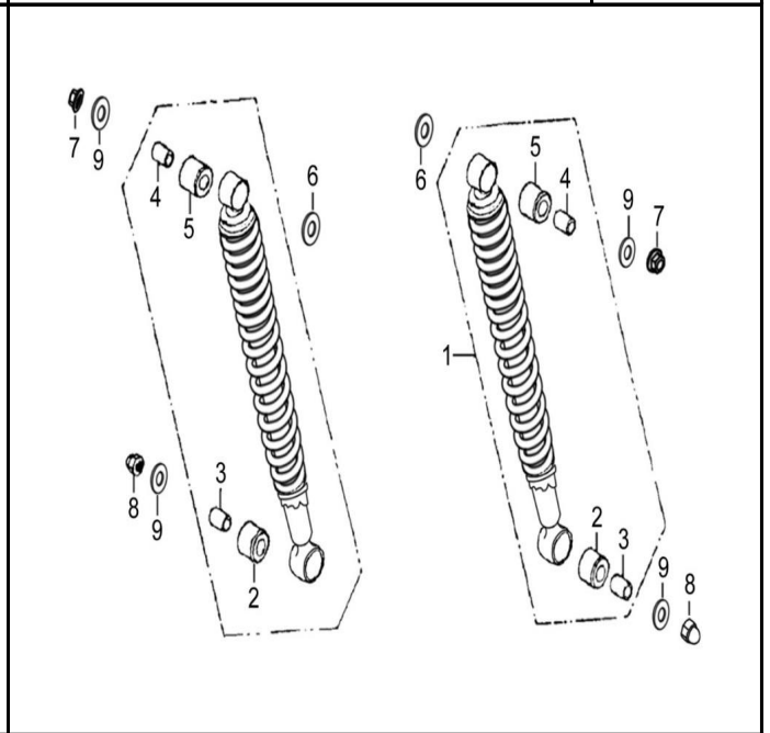
FIG. N° 42 SUSPENSION TRASERA
