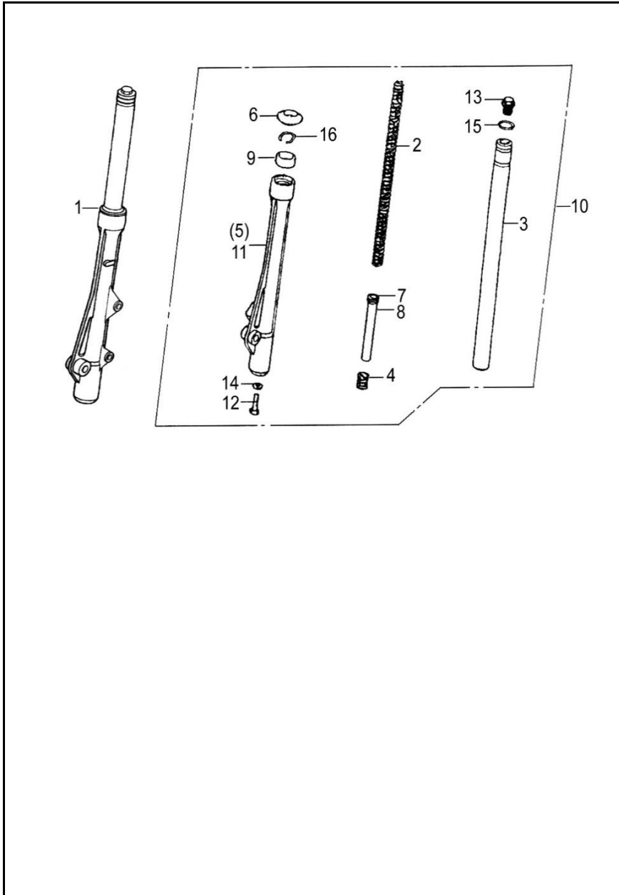
FIGURA N° 27: SUSPENSION DELANTERA
