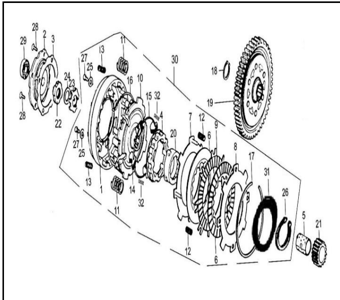
FIG. Nº 7 CLUTCH
