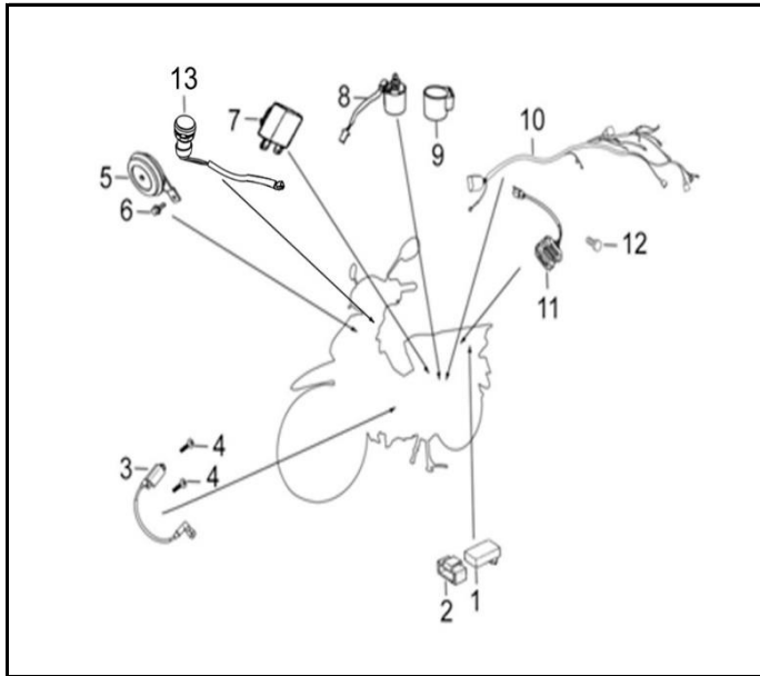
FIG. Nº 49 SISTEMA ELECTRICO
