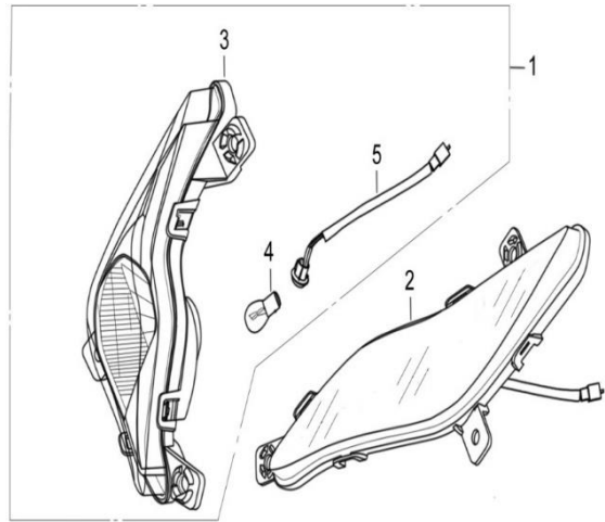
FIG. Nº 43 DIRECCIONALES
