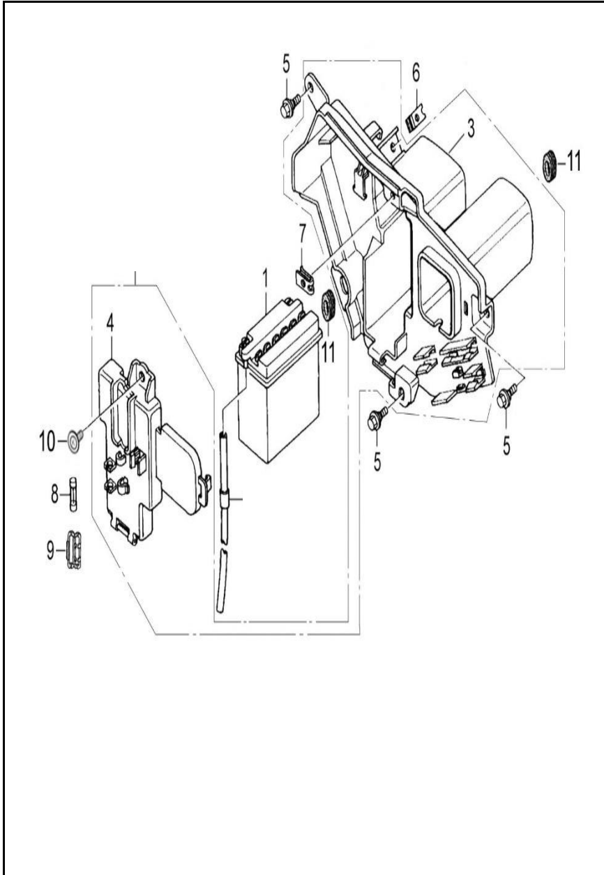
FIGURA N° 48: BATERIA - CAJA BATERIA
