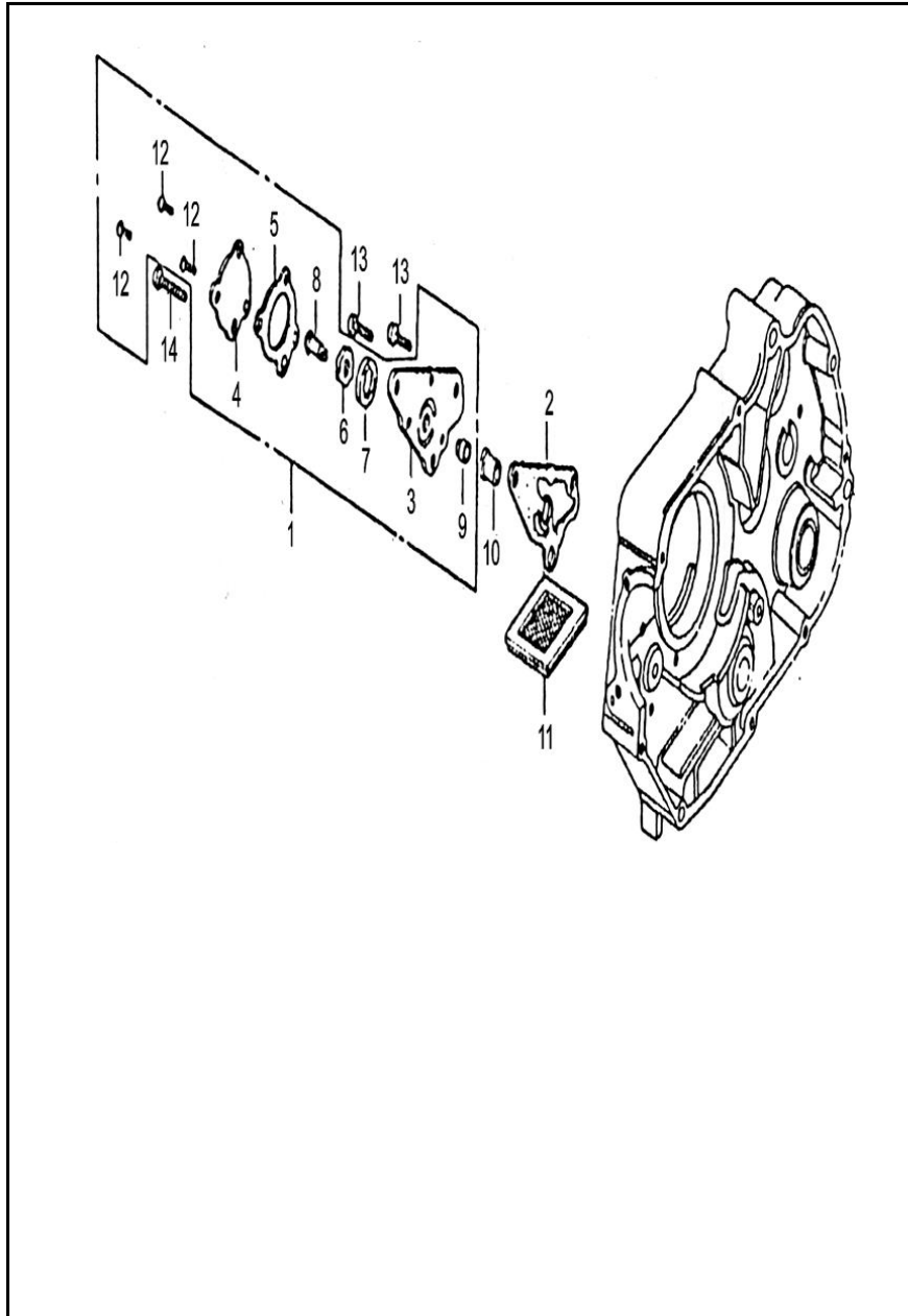
FIGURA N° 9: BOMBA DE ACEITE
