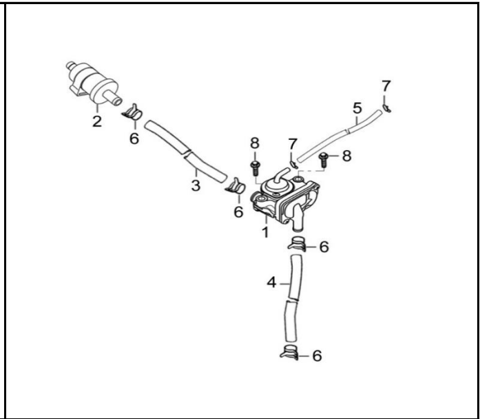
FIG. Nº 51 VALVULA DE GASES
