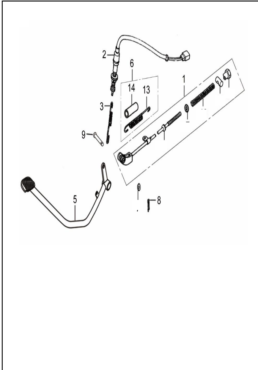
FIGURA N° 40: PEDAL FRENO
