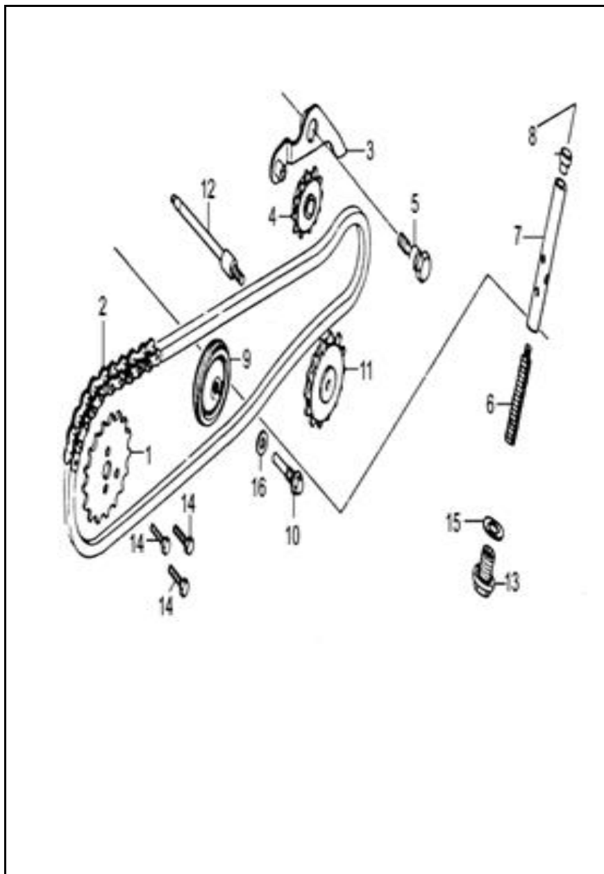
FIGURA N° 4: CADENILLA DISTRIBUCION
