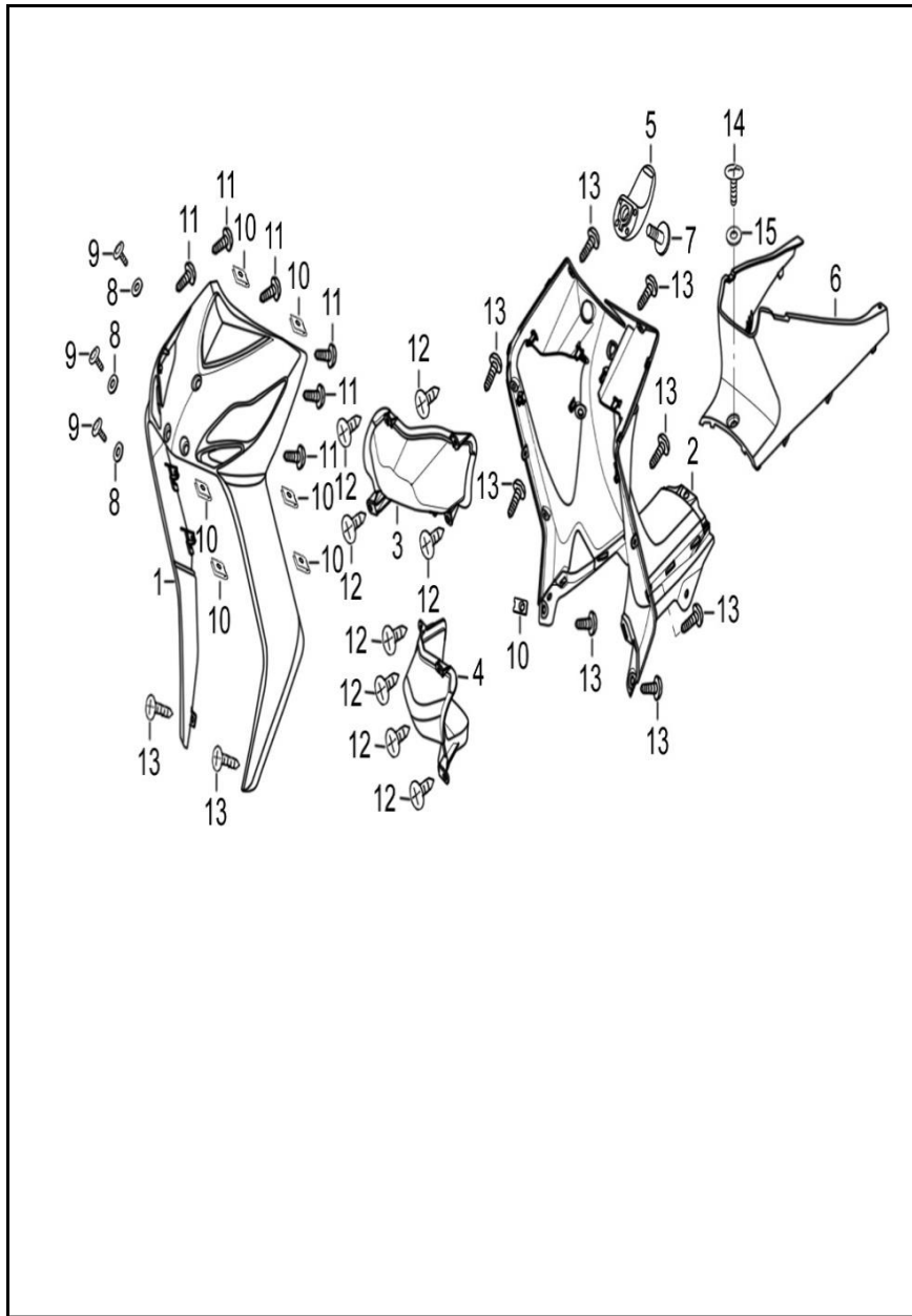
FIGURA N° 44: CARENAJES
