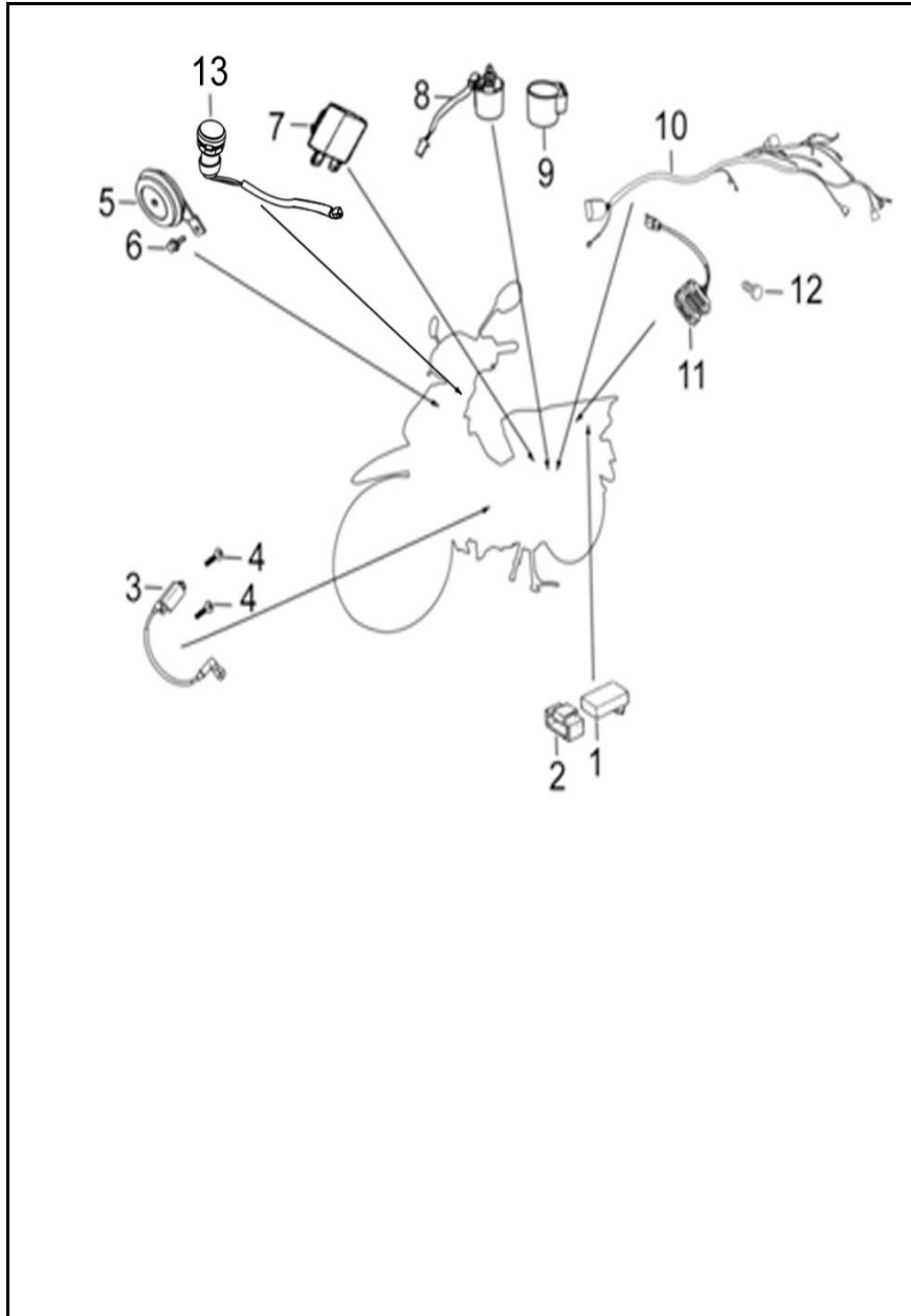
FIGURA N° 49: SISTEMA ELECTRICO
