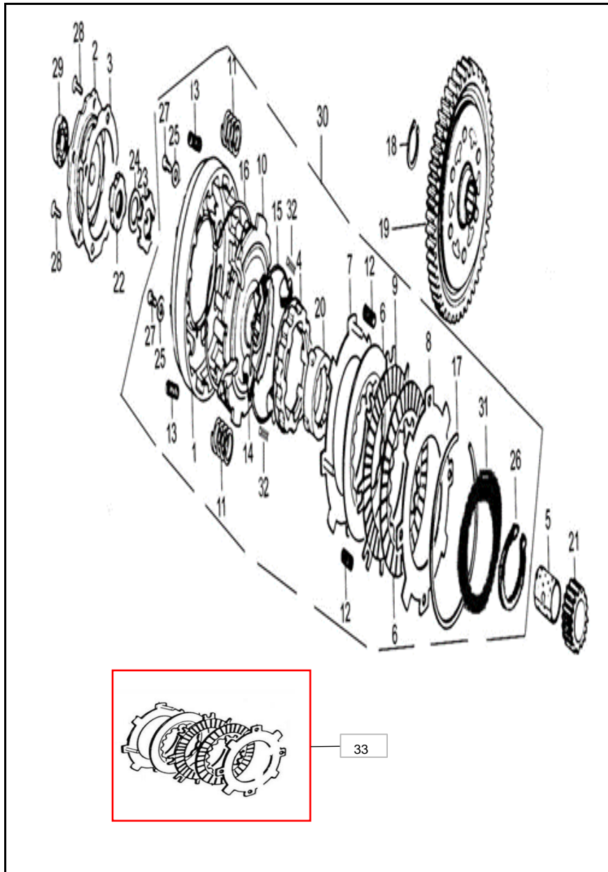
FIGURA N° 7: CLUTCH 2/2
