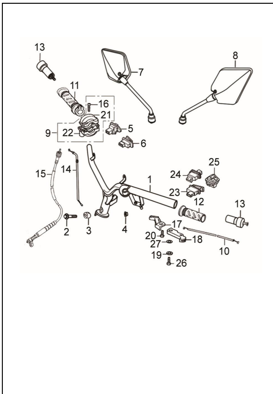
FIGURA N° 24: MANUBRIO - ESPEJOS 1/2
