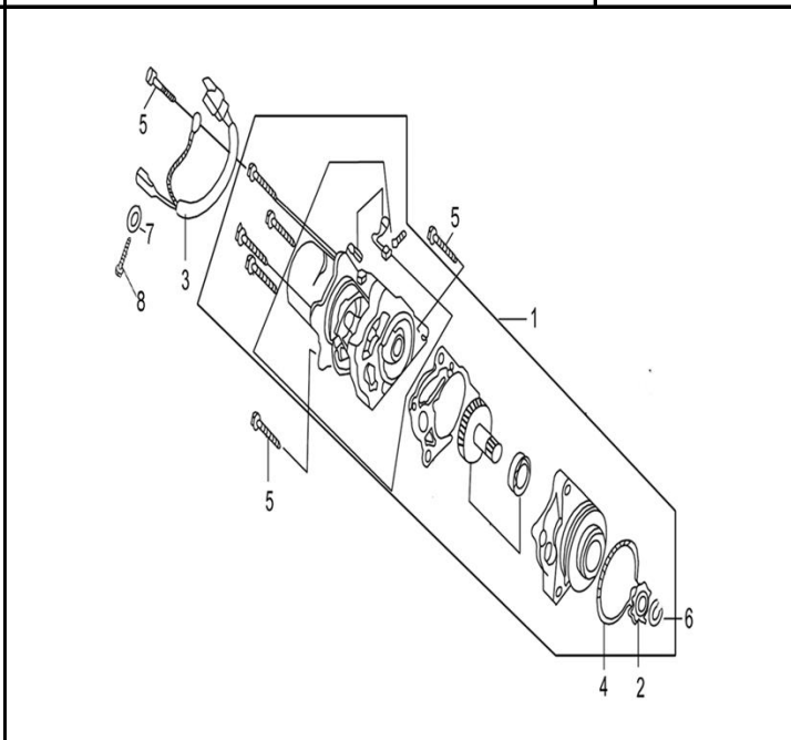
FIG. Nº 11 MOTOR DE ARRANQUE
