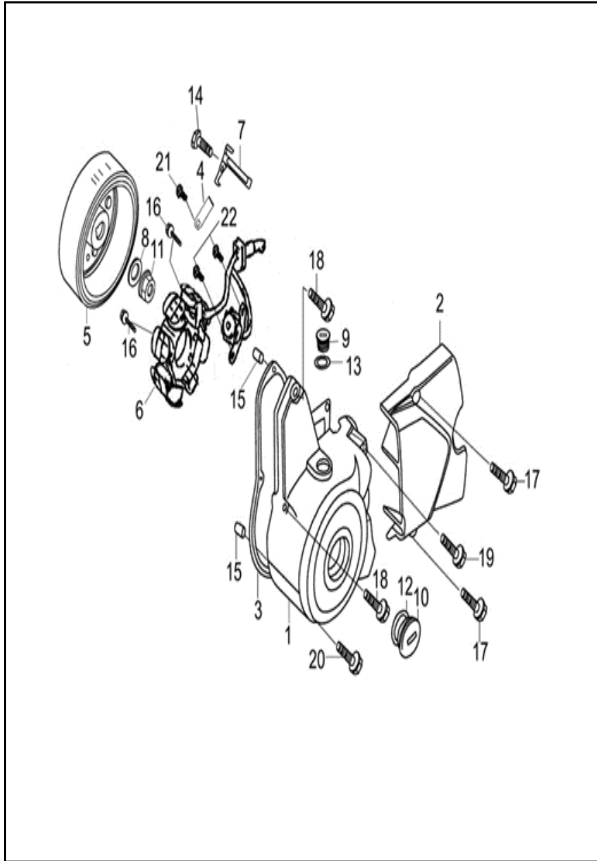
FIGURA N° 8: CUBIERTA VOLANTE - MAGNETO
