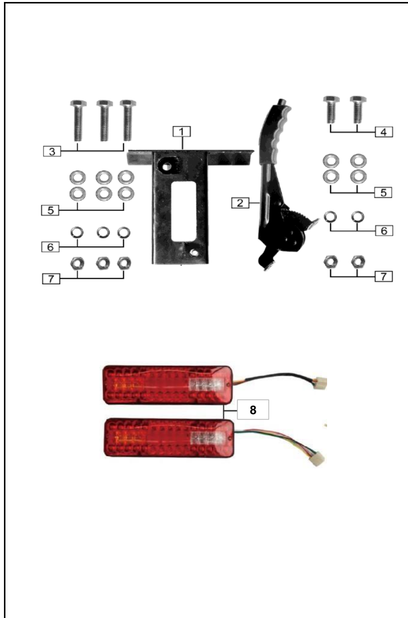
FIGURA N° 28: PALANCA DE REVERSA - STOP
