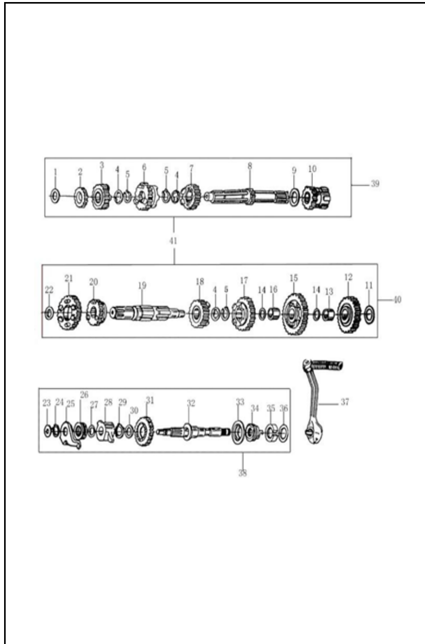
FIGURA N°8: TRANSMISIÓN (1/2)
