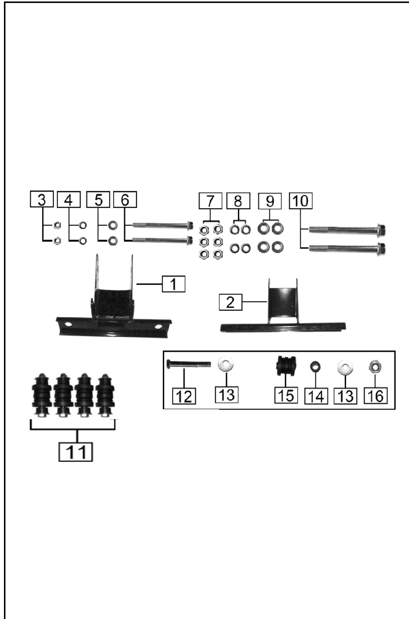
FIGURA N° 22: COMPLEMENTOS CHASIS
