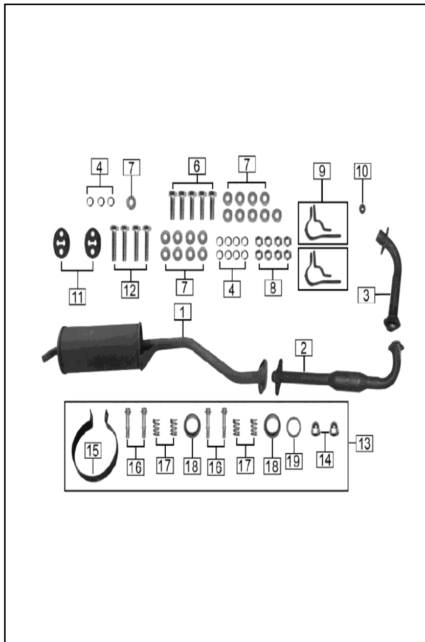
FIGURA N° 26: SILENCIADOR
