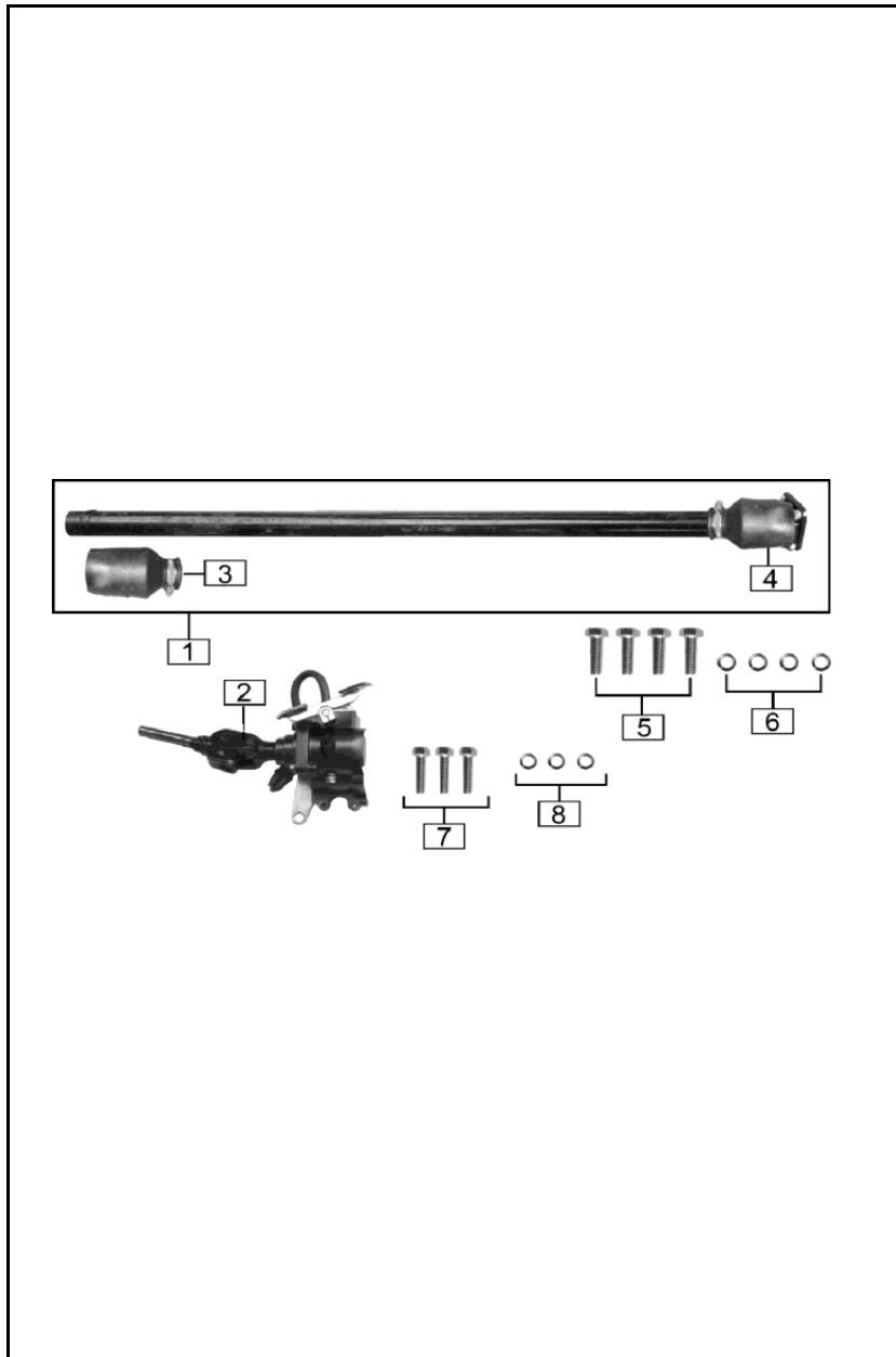
FIGURA N° 38: EJE DE TRANSMISIÓN
