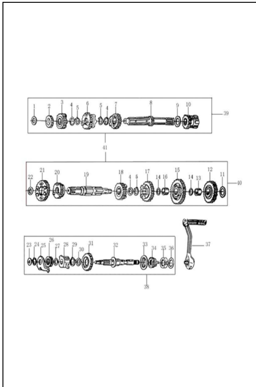
FIGURA N°8: TRANSMISIÓN (2/2)
