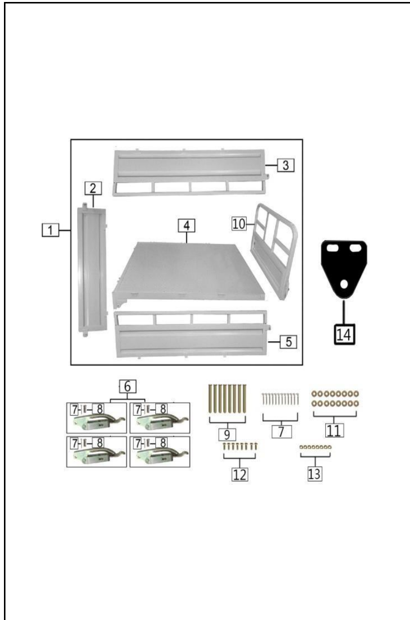
FIGURA N° 34: CARROCERÍA
