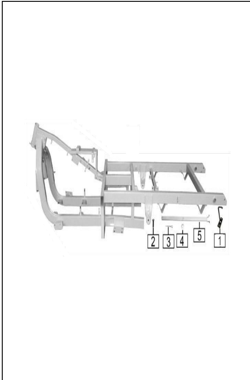
FIGURA N° 33: CHASIS
