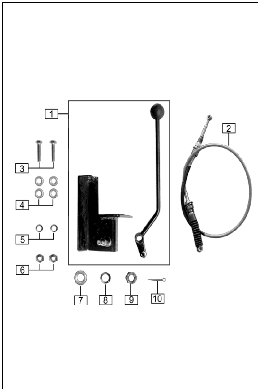
FIGURA N° 29: PALANCA CONTROL TRACCIÓN
