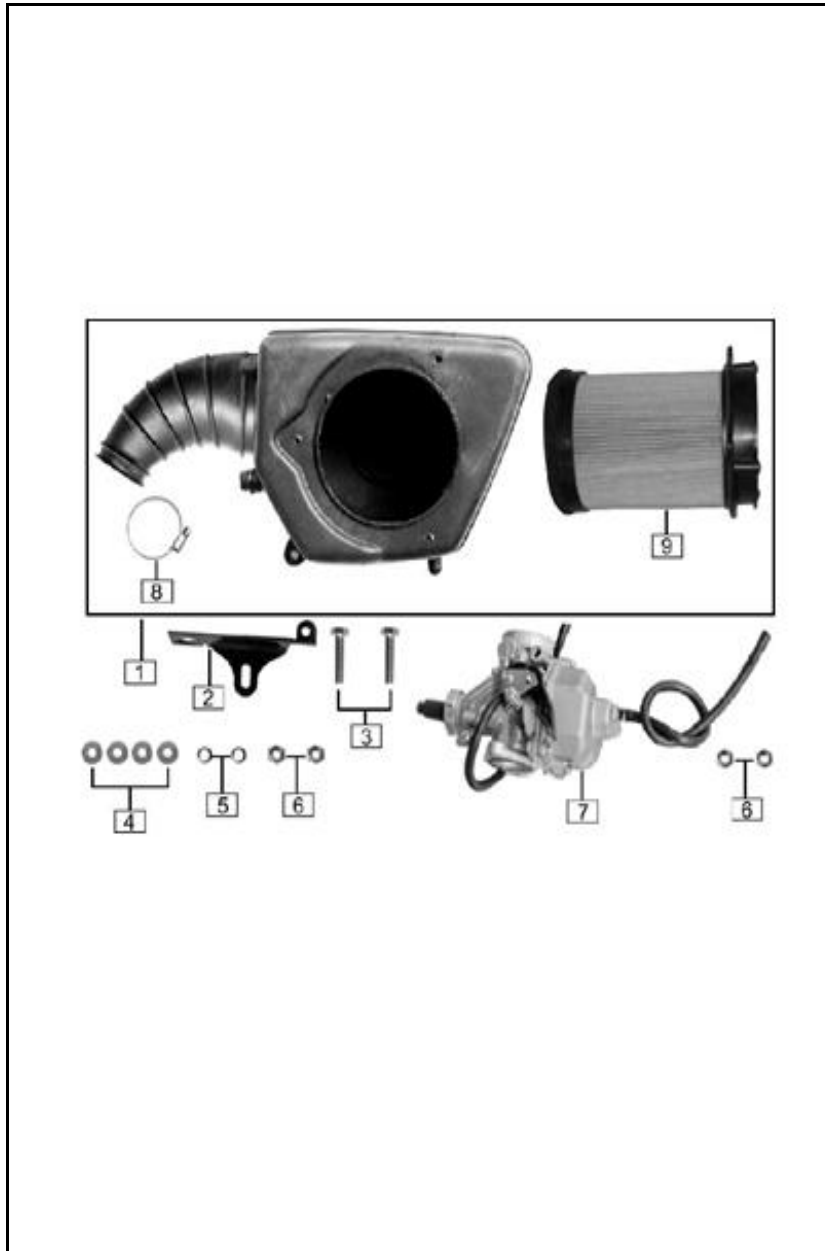
FIGURA N° 12: CAJA FILTRO AIRE - CARBURADOR
