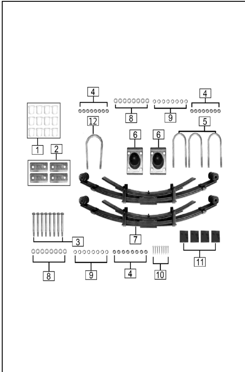
FIGURA N° 36: SUSPENSIÓN TRASERA
