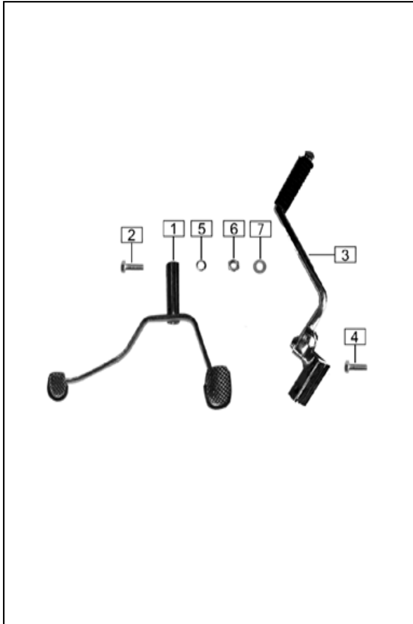
FIGURA N° 16: PEDAL CAMBIOS - PEDAL FRENO
